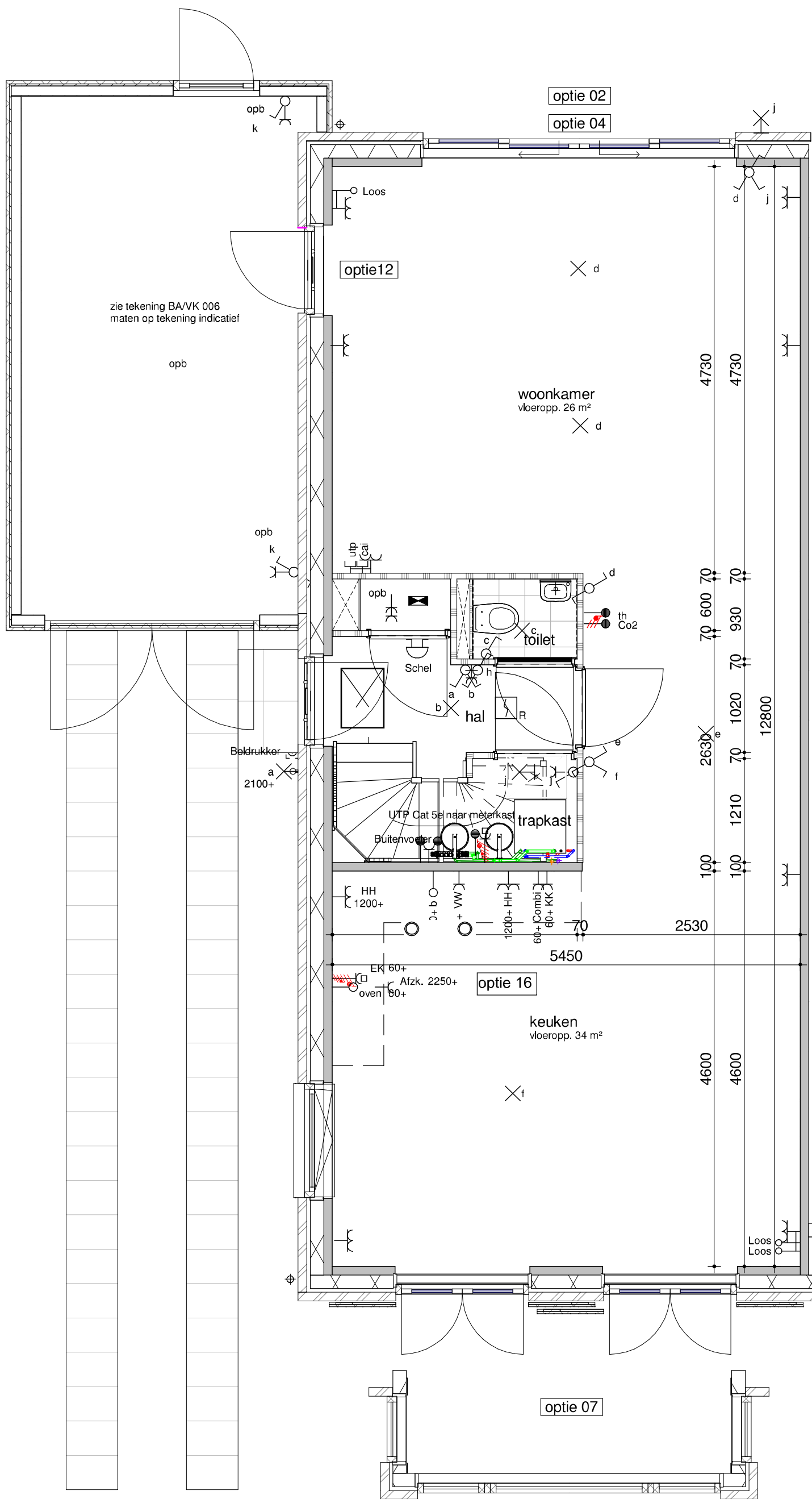
bouwnummer get. 21 begane grond - optie 2400
