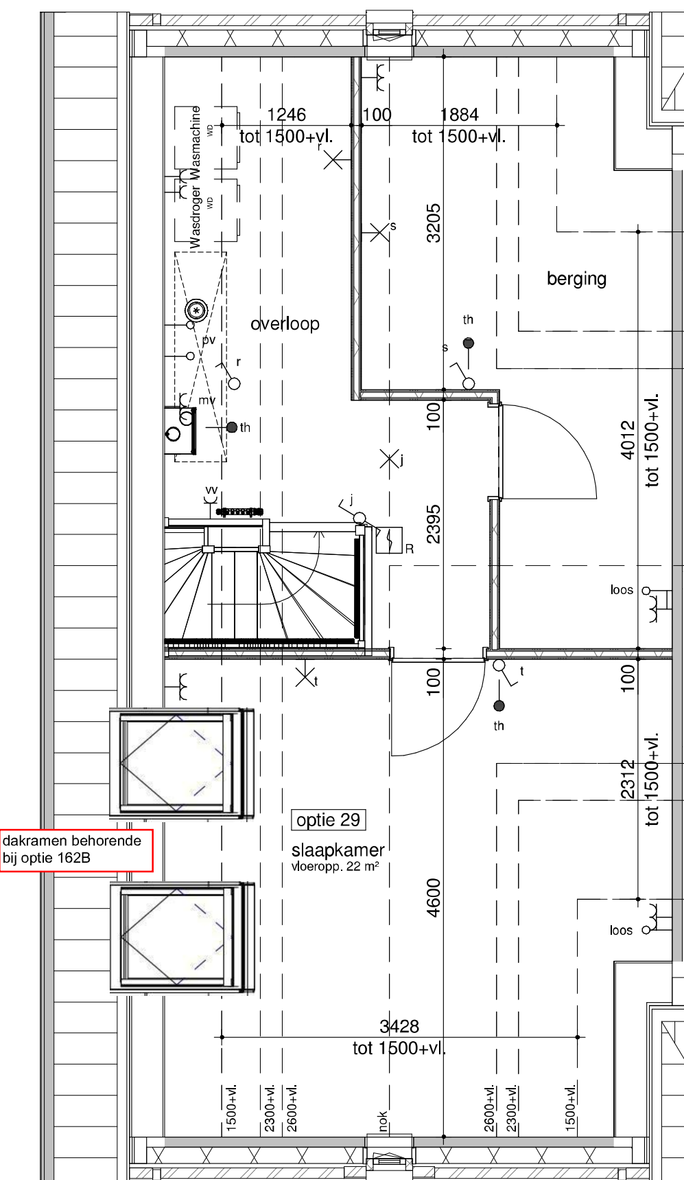
bouwnummer get. 21 tweede verdieping - zolderindeling
