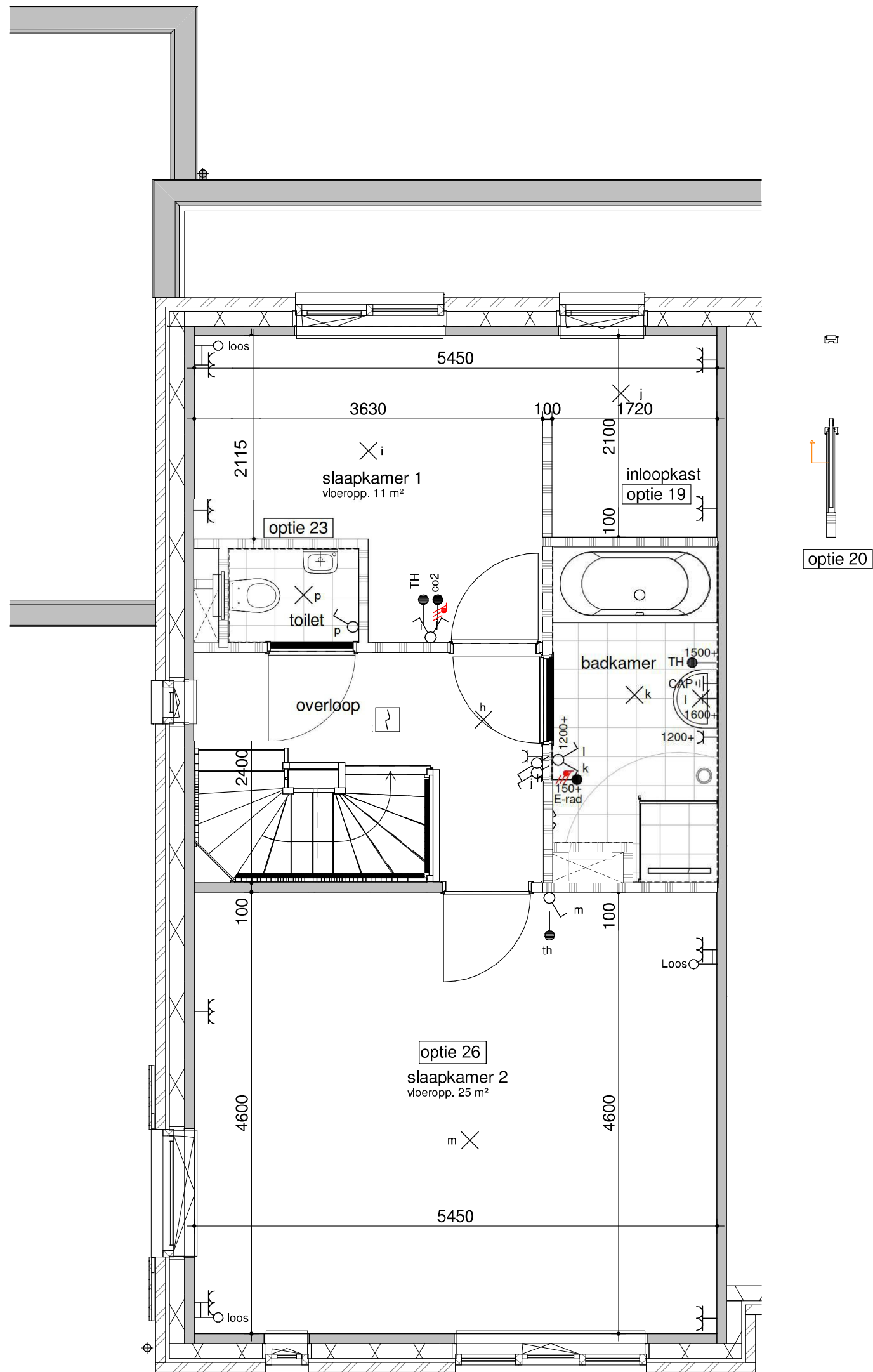
bouwnummer get. 21 eerste verdieping - samenvoegen slaapkamer 2 en 3
