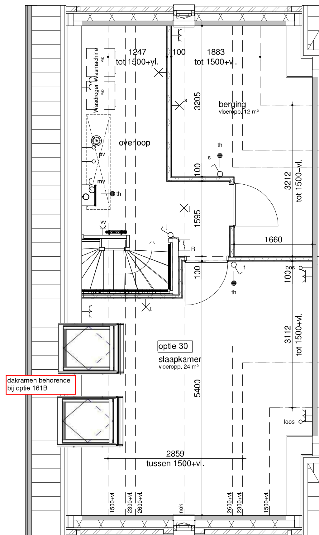
bouwnummer get. 21 tweede verdieping - zolderindeling
