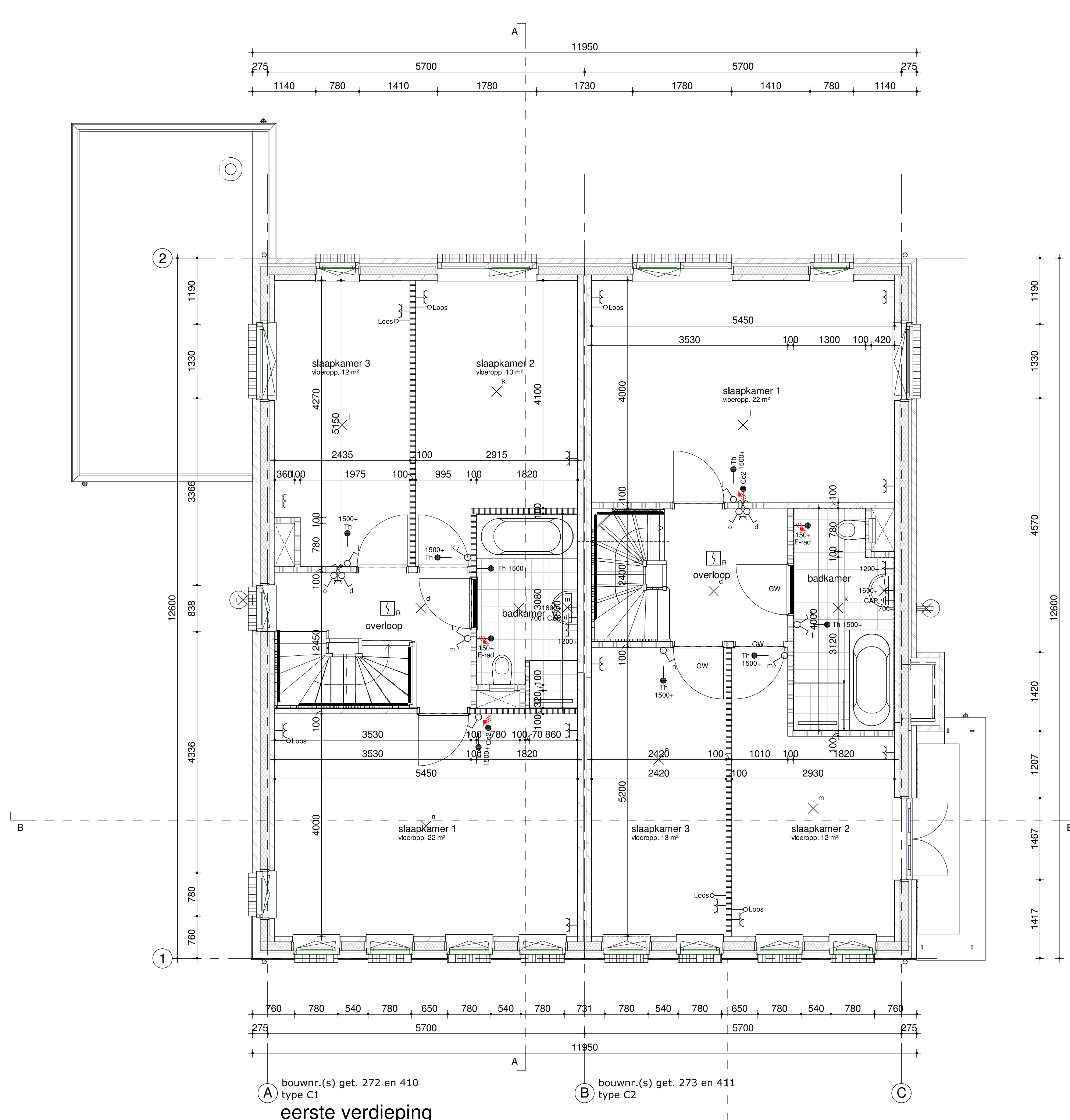
eerste verdieping
