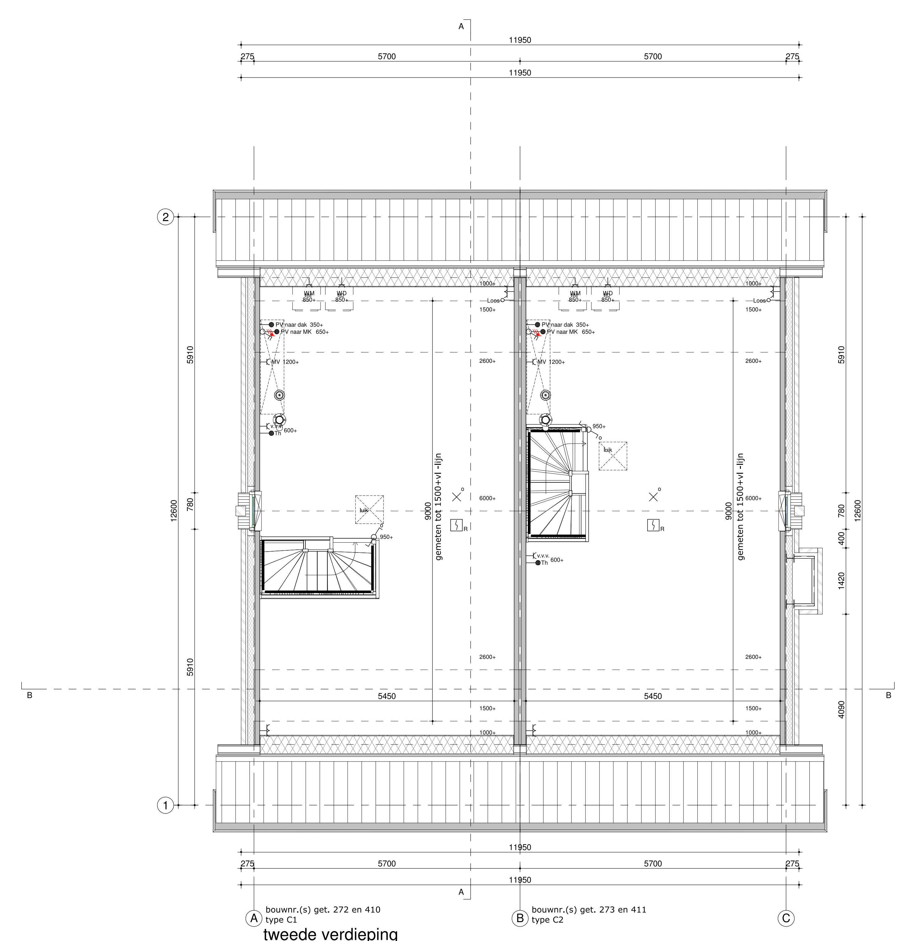
tweede verdieping
