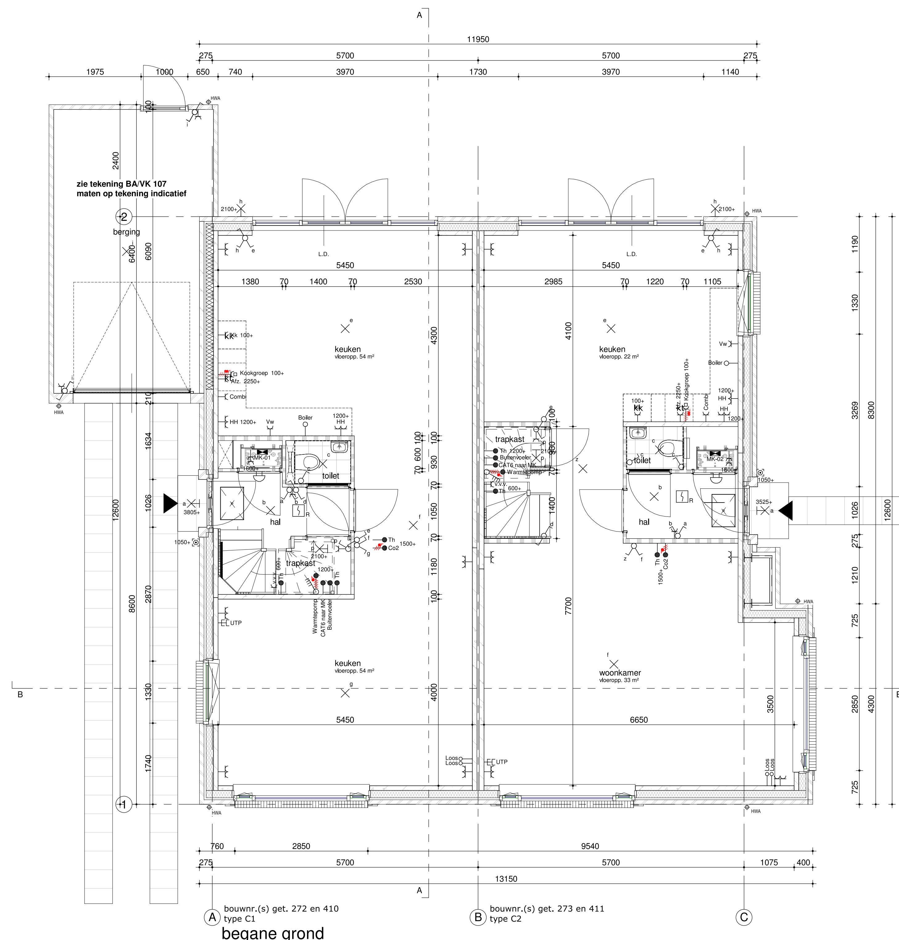
begane grond
