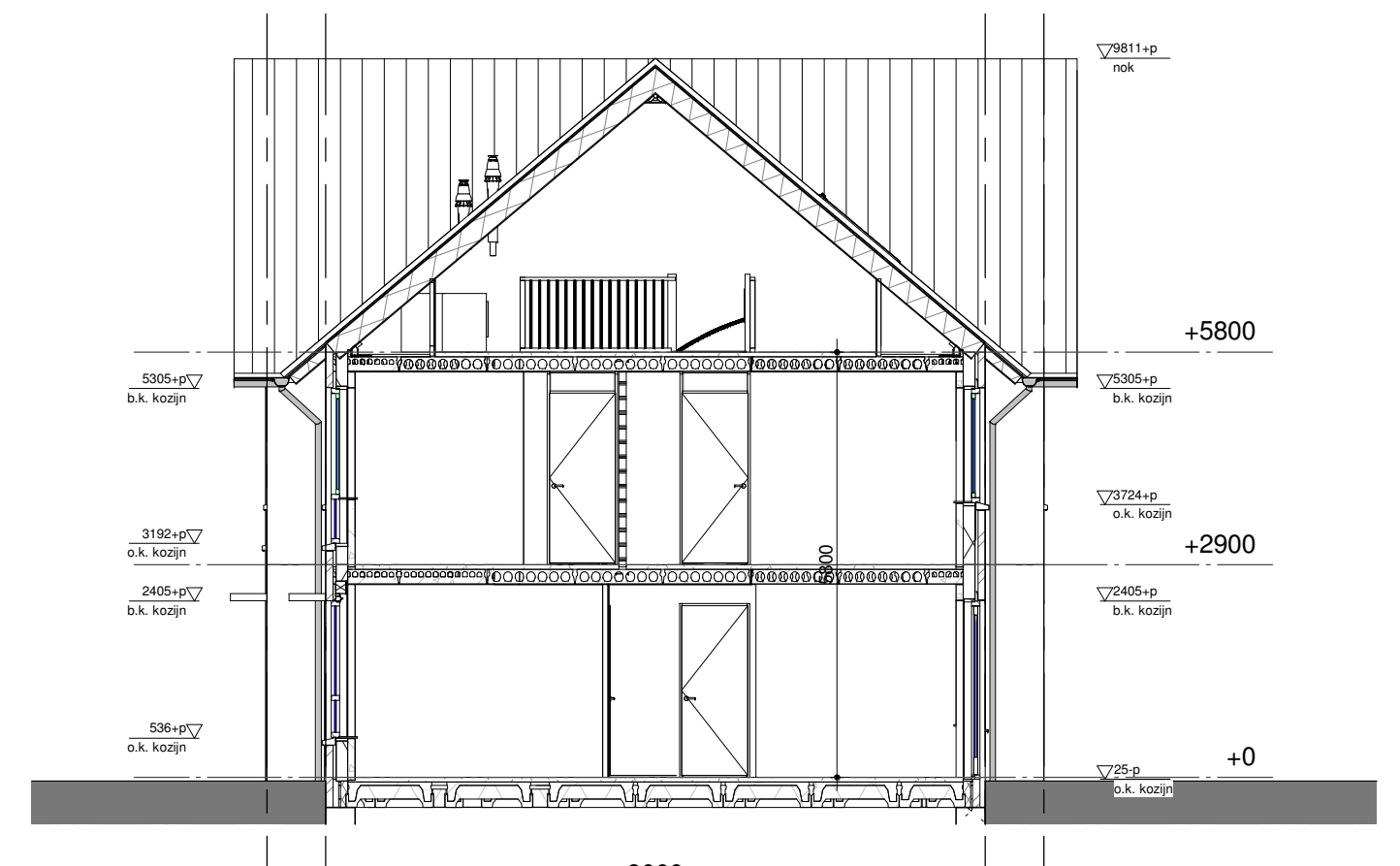
doorsnede B-B 1:100
