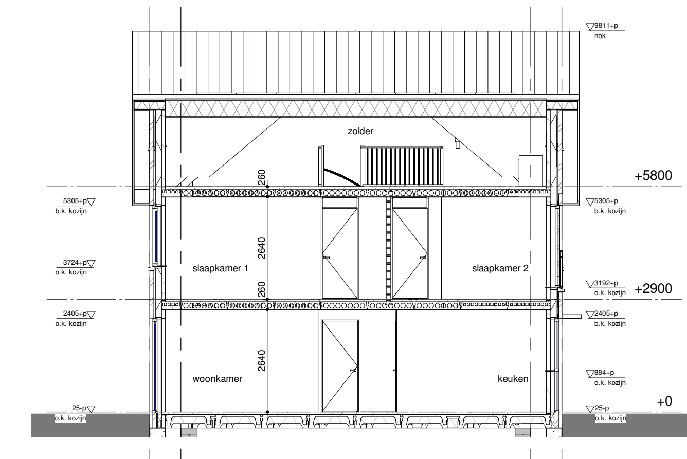
doorsnede A-A 1:100
