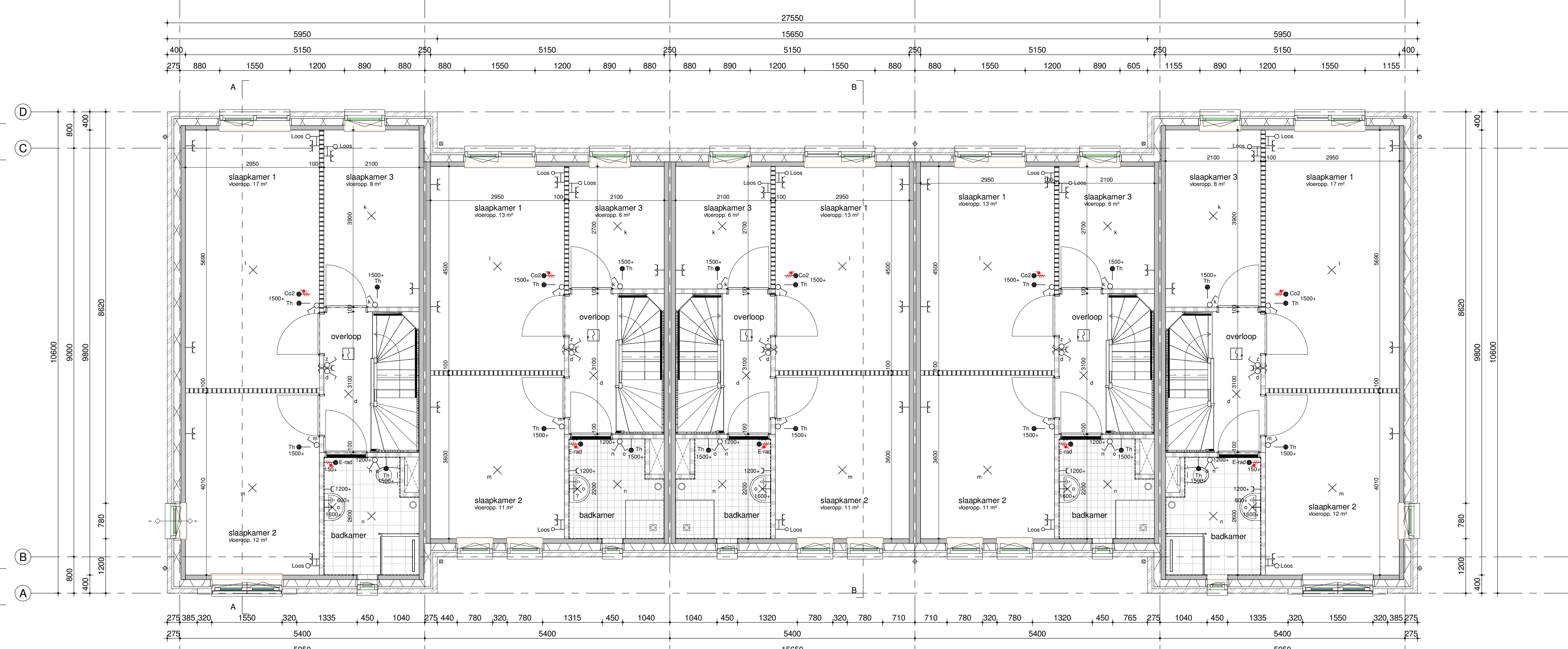
eerste verdieping / 2900+P 1:50
