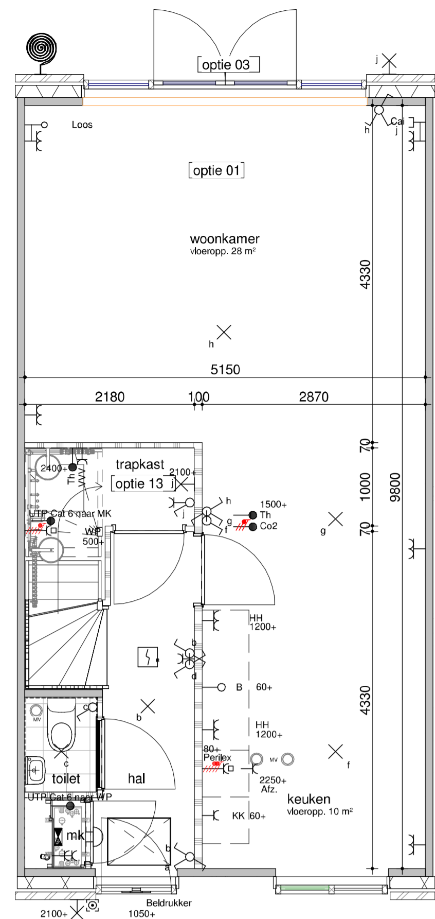
bouwnummer 413 begane grond - optie 1200 1:50
