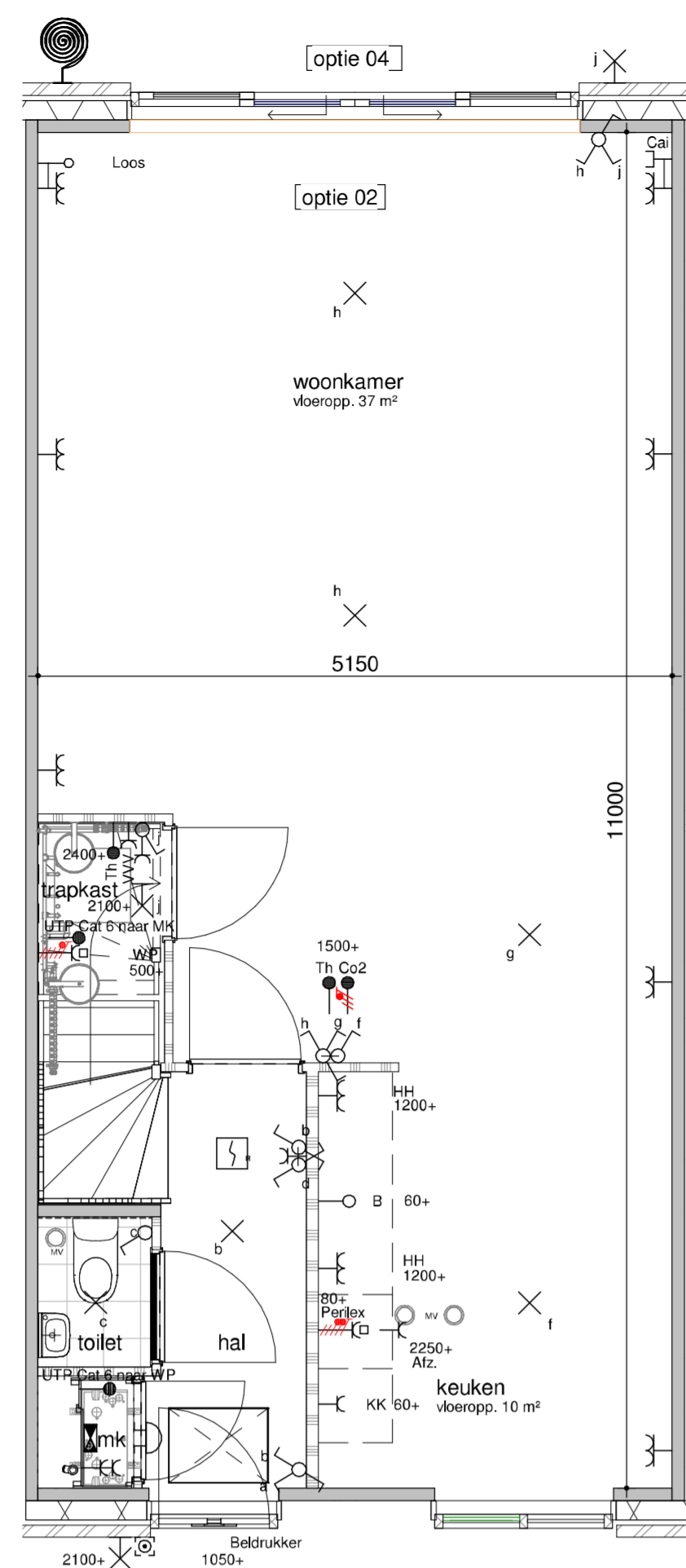
bouwnummer 413 begane grond - optie 2400 1:50
