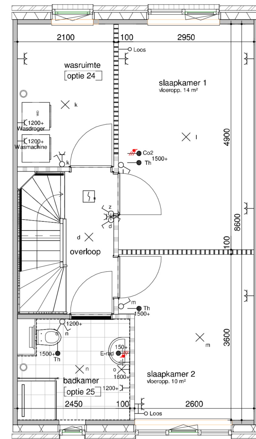
bouwnummer 413 eerste verdieping - vergrote badkamer 1:50
