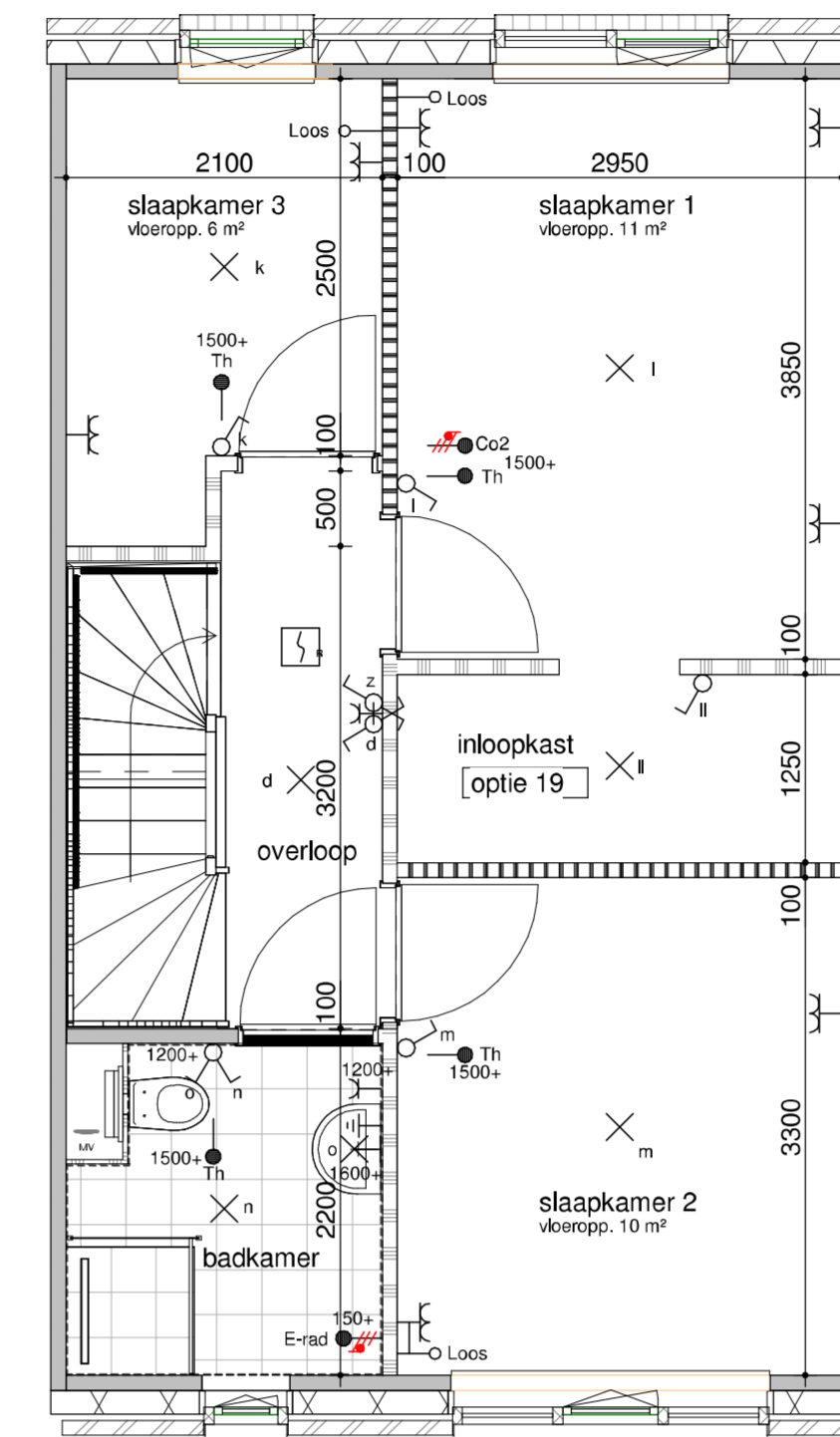
bouwnummer 413 eerste verdieping - inloopkast 1:50
