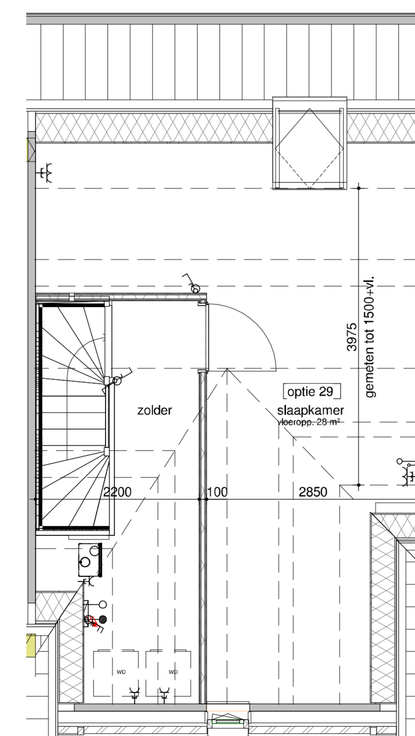
bouwnummer 413 tweede verdieping - zolder L indeling 1:50
