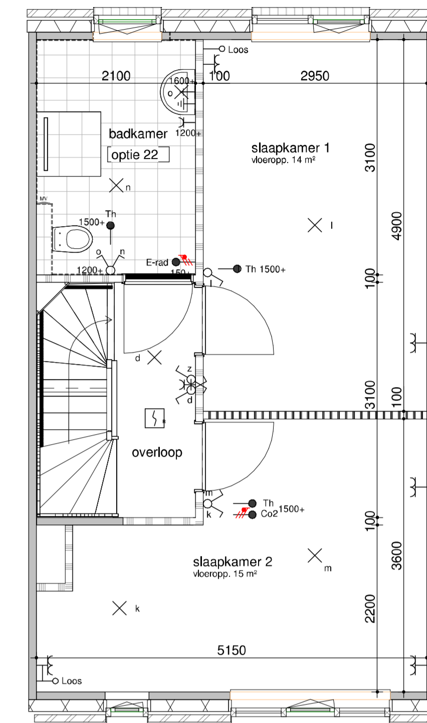
bouwnummer 413 eerste verdieping - badkamer achter 1:50
