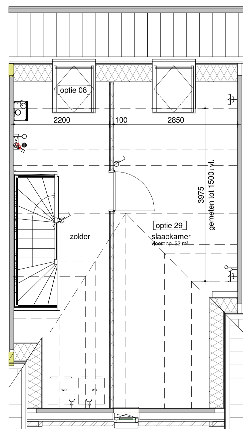
bouwnummer 413 tweede verdieping - zolderindeling 1:50
