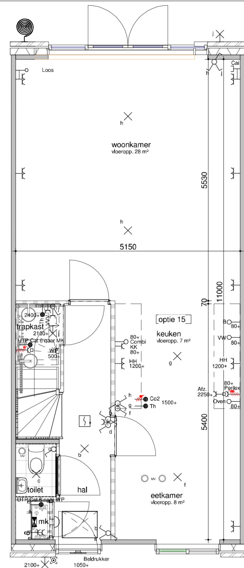
bouwnummer 413 begane grond - optie middenkeuken 1:50
