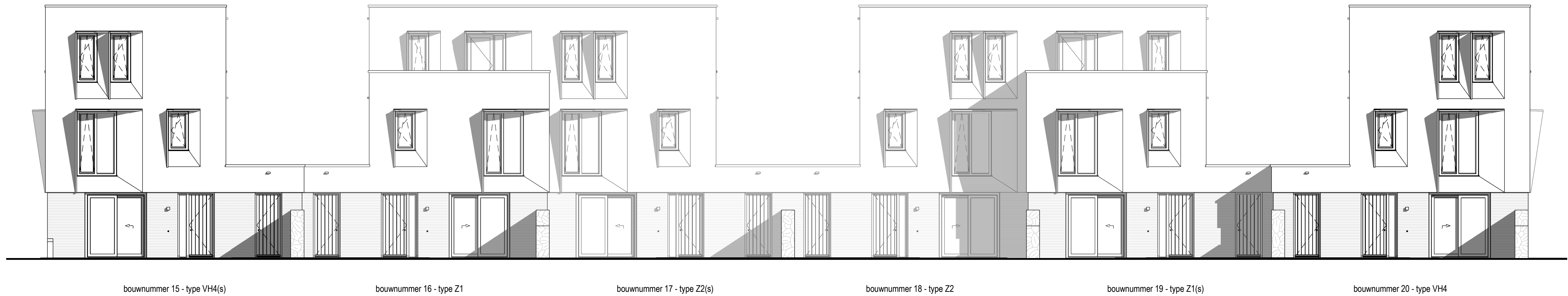
Voorgevel - Blok D 1 : 100
