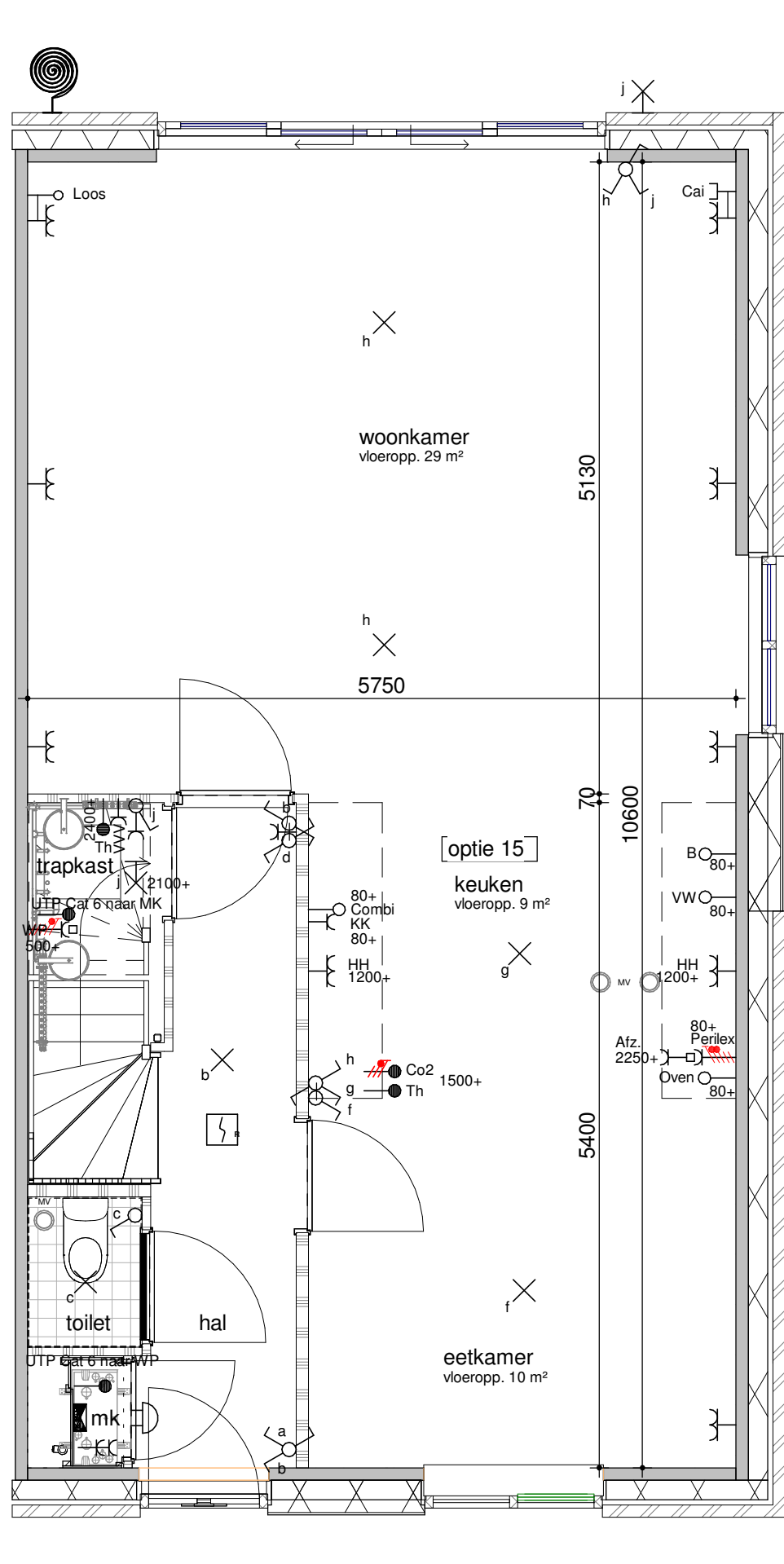
begane grond - optie middenkeuken 1:50
