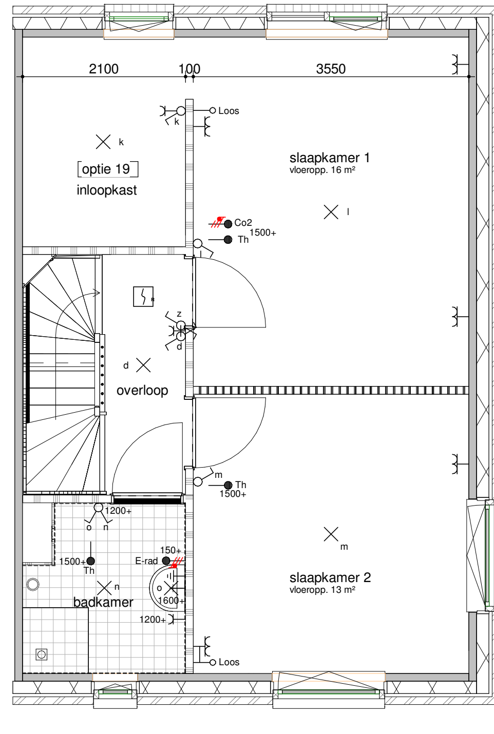
eerste verdieping - inloopkast 1:50
