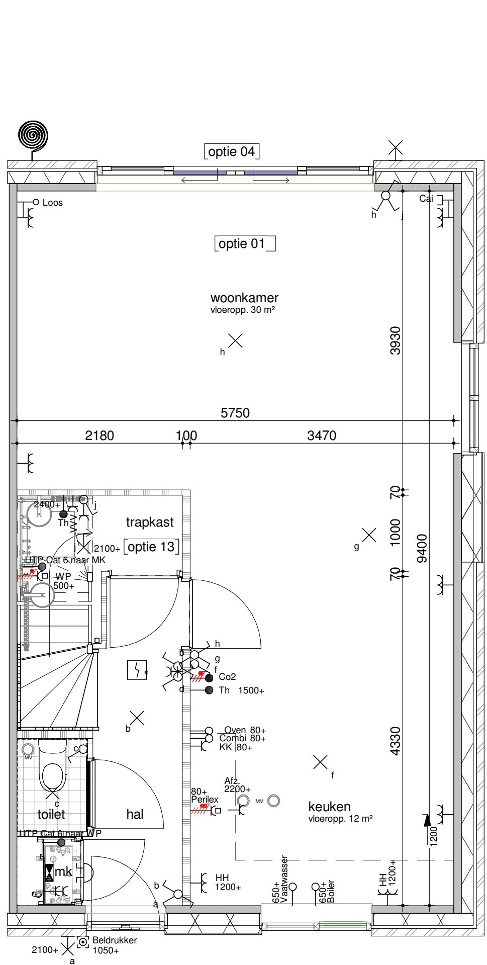
begane grond - optie 1200 1:50
