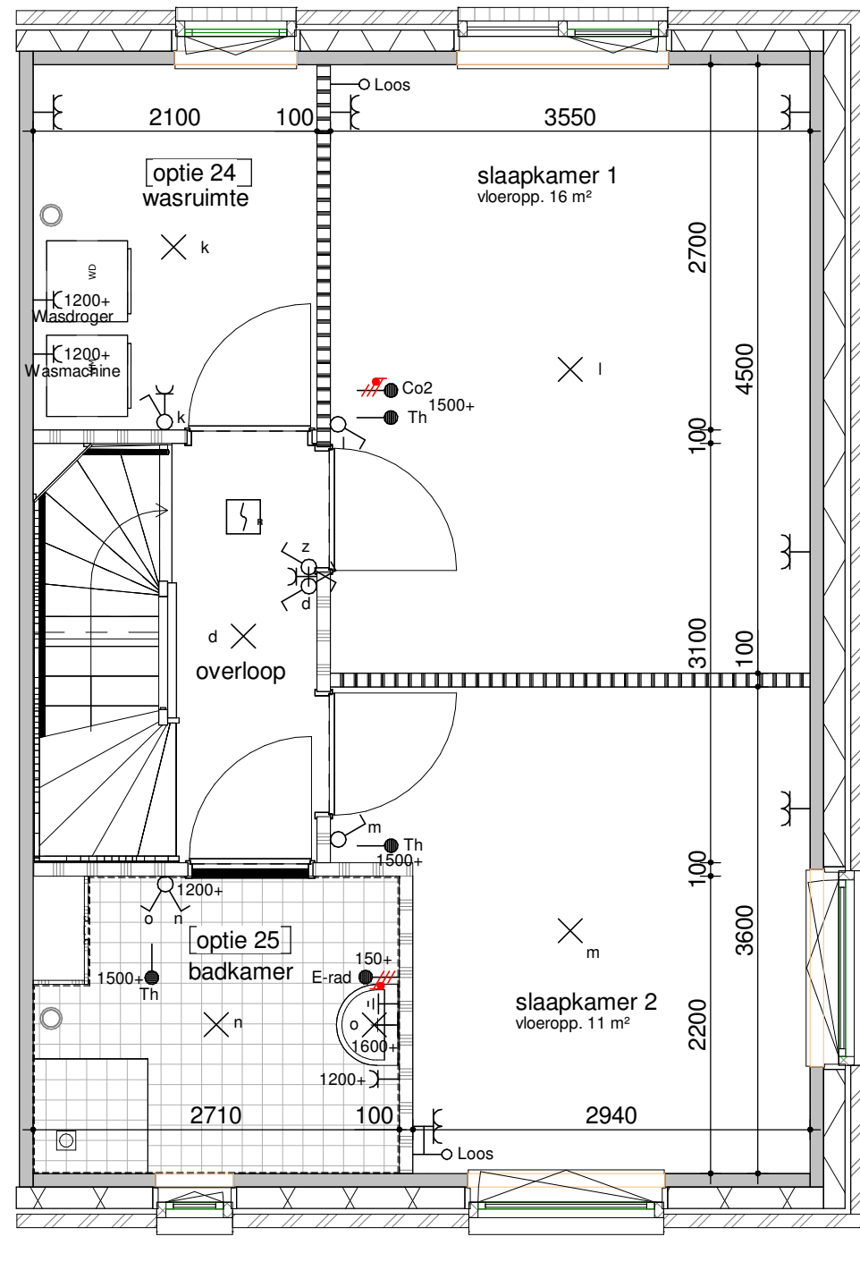
eerste verdieping - vergrote badkamer 1:50
