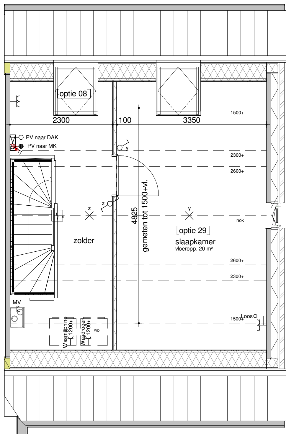
tweede verdieping - zolderindeling 1:50
