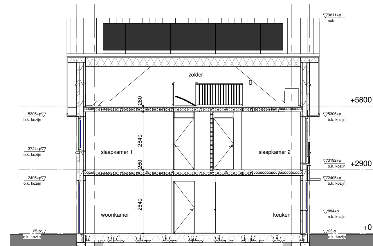
doorsnede A-A
