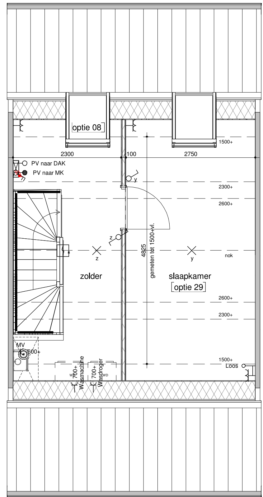
bouwnummer 325, 326, 327 tweede verdieping - zolderindeling 1 : 50
