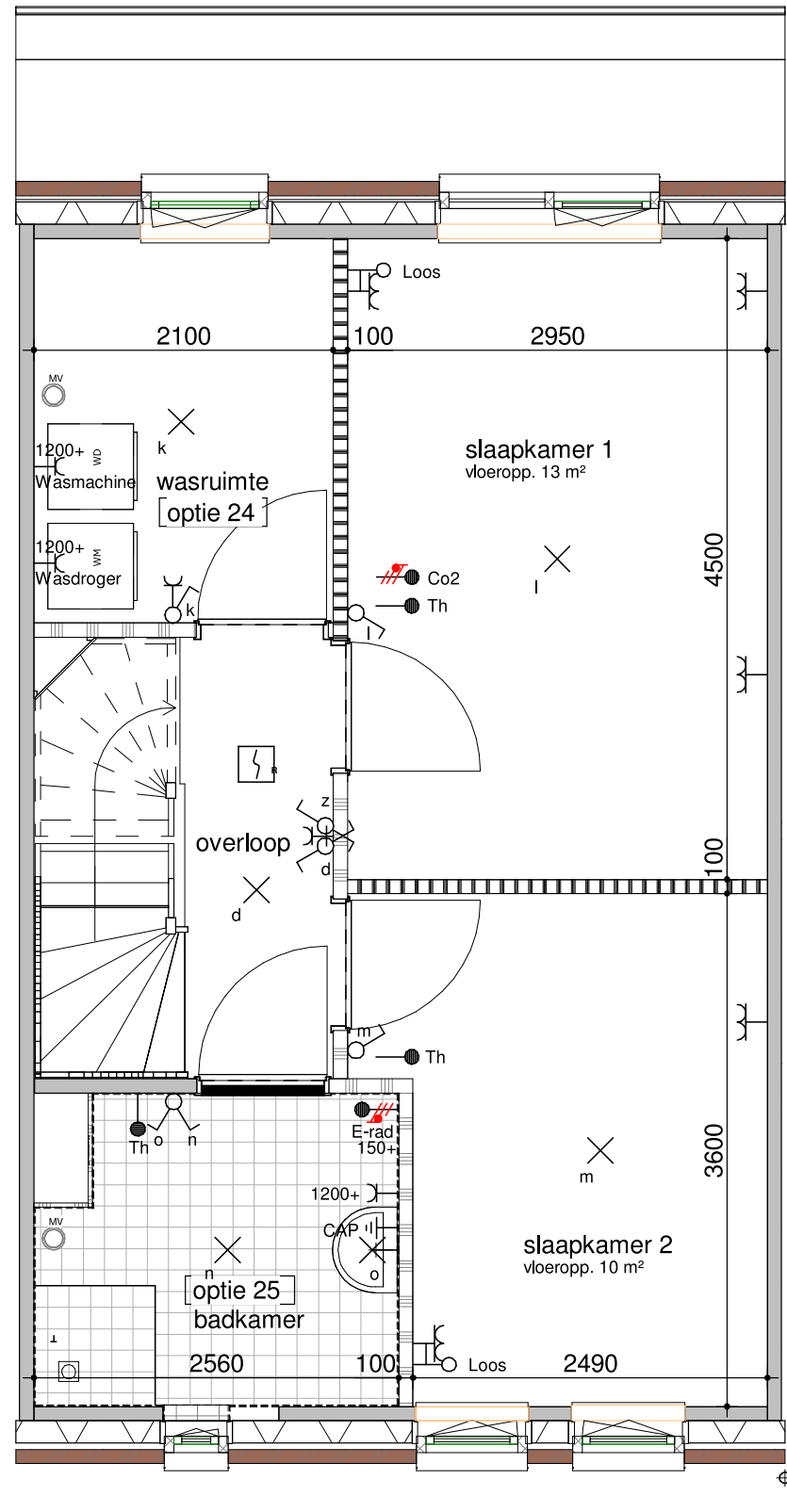
bouwnummer 325, 326, 327 eerste verdieping - vergrote badkamer 1 : 50
