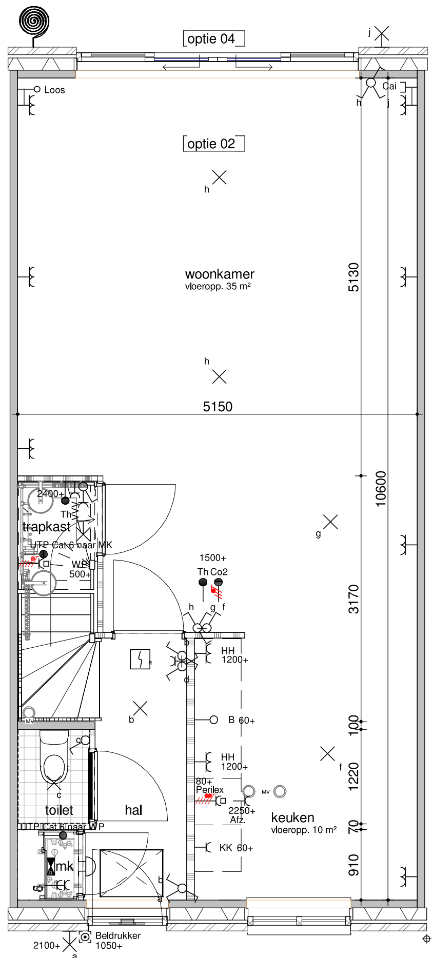
bouwnummer 325, 326, 327 begane grond - optie 2400 1 : 50
