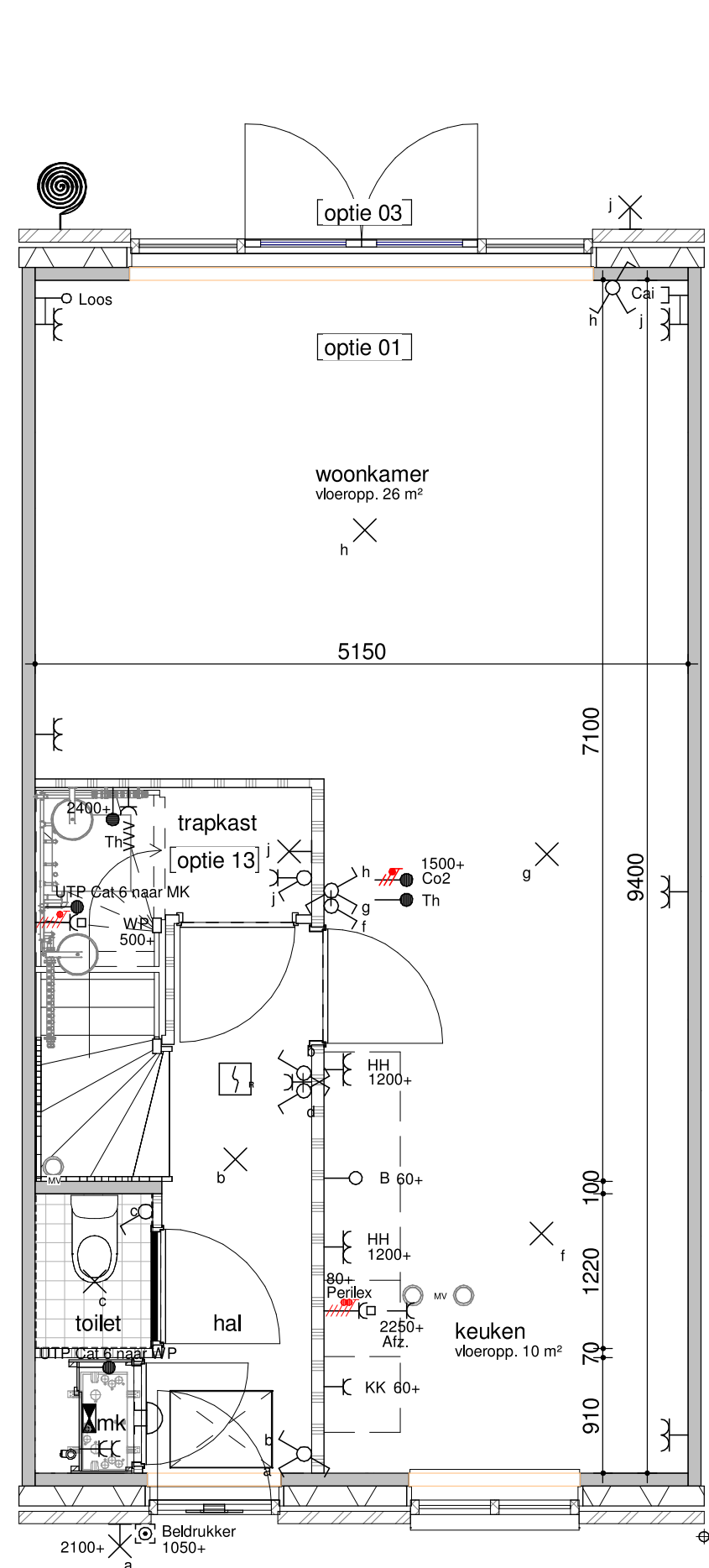
bouwnummer 325, 326, 327 begane grond - optie 1200 1 : 50
