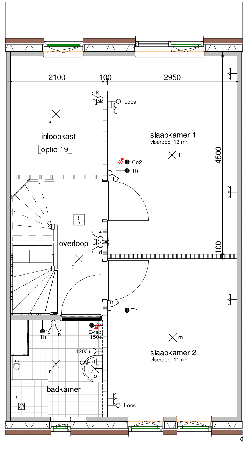
bouwnummer 325, 326, 327 eerste verdieping - inloopkast 1 : 50
