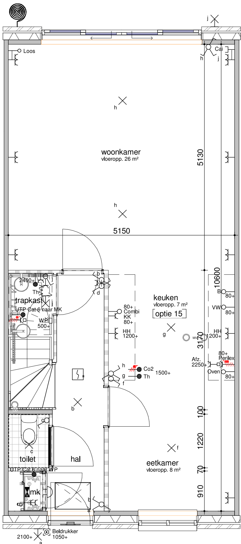
bouwnummer 325, 326, 327 begane grond - optie middenkeuken 1 : 50
