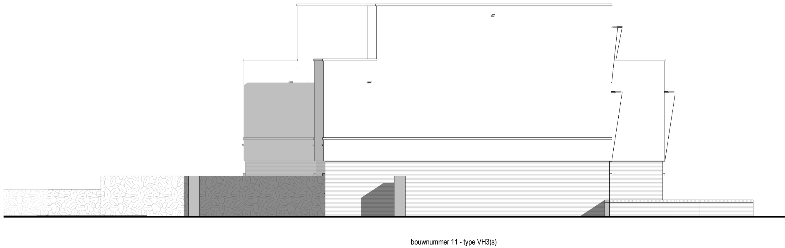
Rechter zijgevel - Blok B 1 : 100
