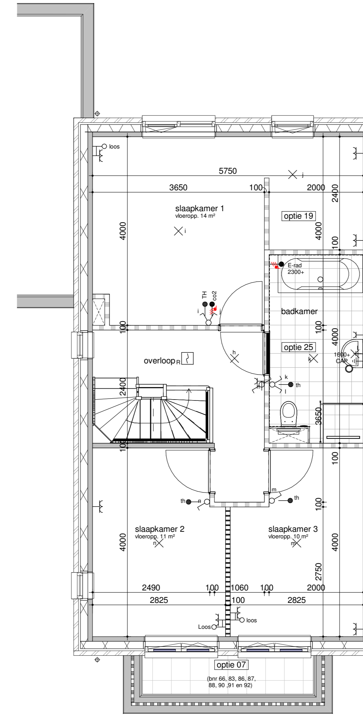
bouwnummer get. 65, 83, 85, 87, 91 gesp. 66, 86, 88, 90, 92 eerste verdieping - vergrote badkamer 1:50
