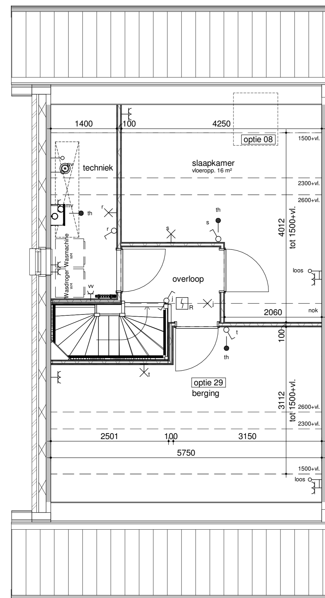
bouwnummer get. 65, 83, 85, 87, 91 gesp. 66, 86, 88, 90, 92 tweede verdieping - zolderindeling 1:50
