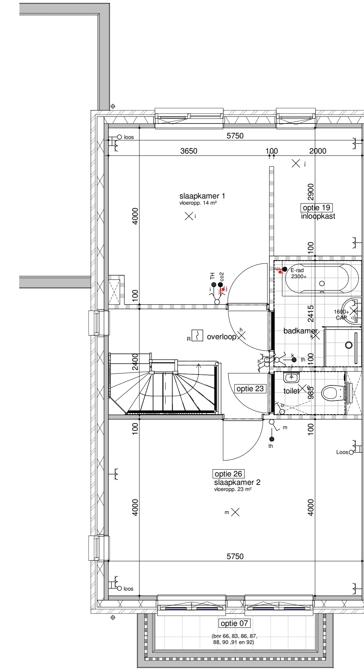
bouwnummer get. 65, 83, 85, 87, 91 gesp. 66, 86, 88, 90, 92 eerste verdieping - samenvoegen slaapkamer 2 en 3 1:50
