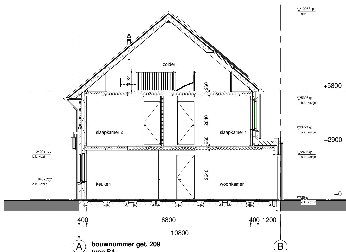
bouwnummer get. 209 type B4 doorsnede B-B 1:100
