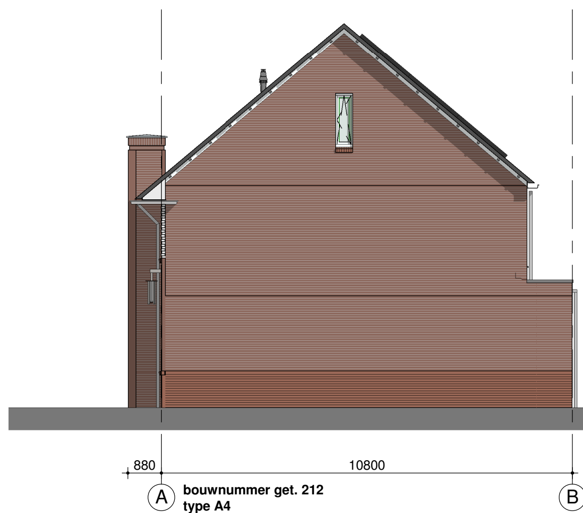
bouwnummer get. 212 type A4 rechter zijgevel 1:100
