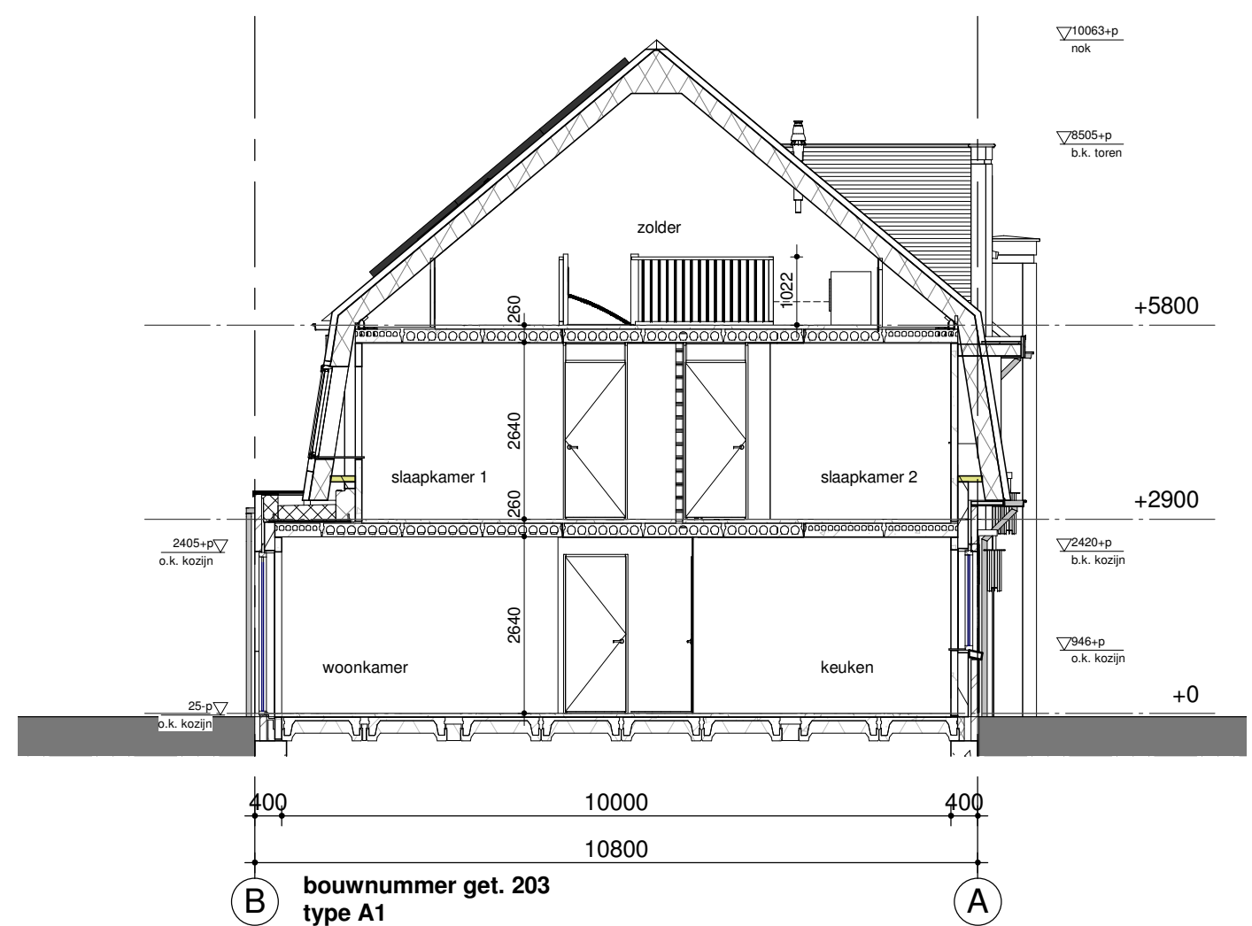
bouwnummer get. 203 type A1 doorsnede A-A 1:100
