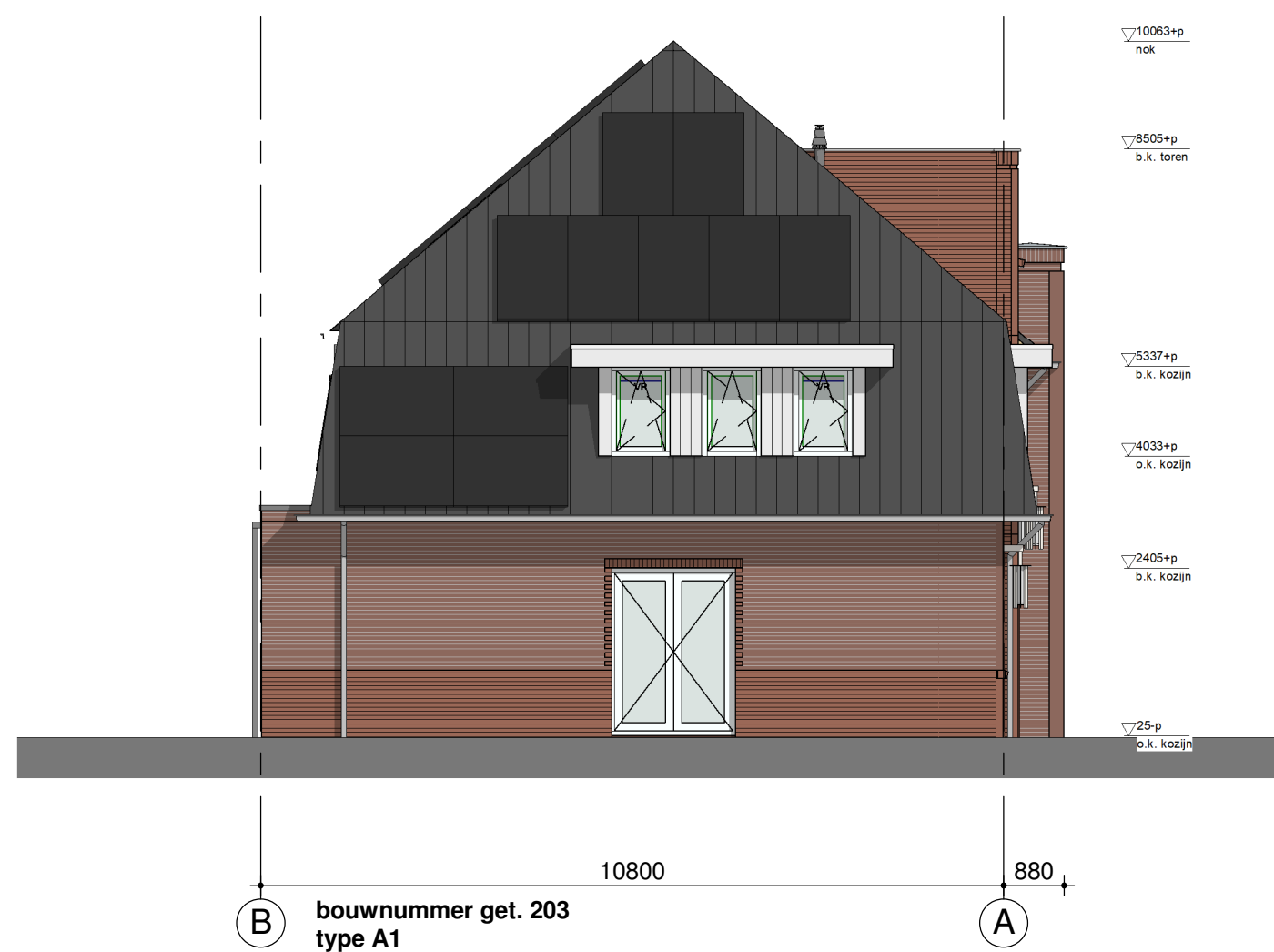
bouwnummer get. 203 type A1 linker zijgevel 1:100
