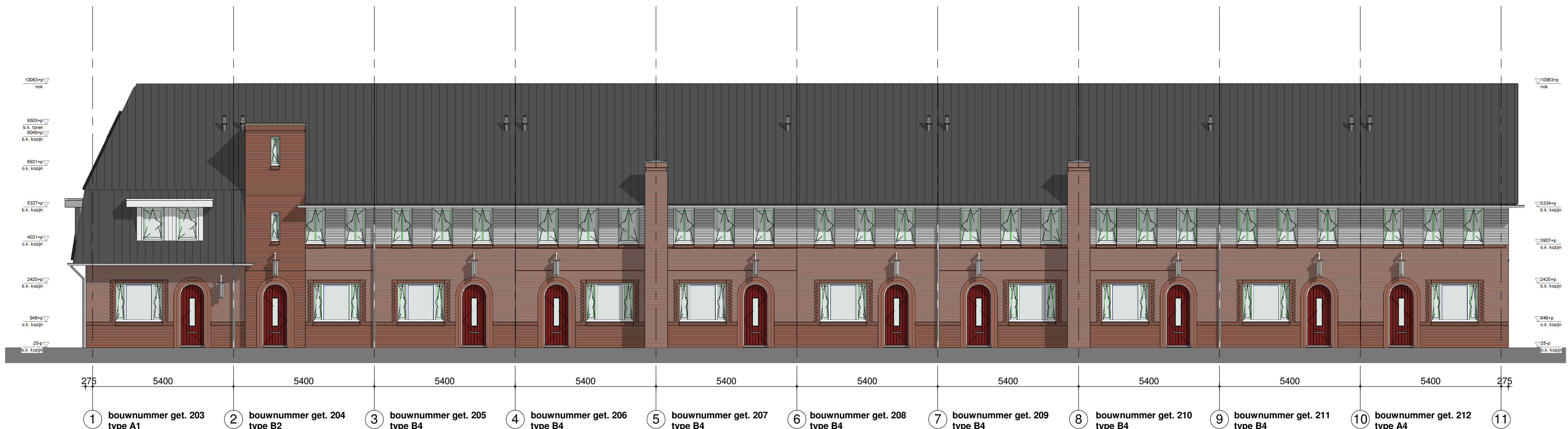
bouwnummer get. 203 type A1 voorgevel 1:100
