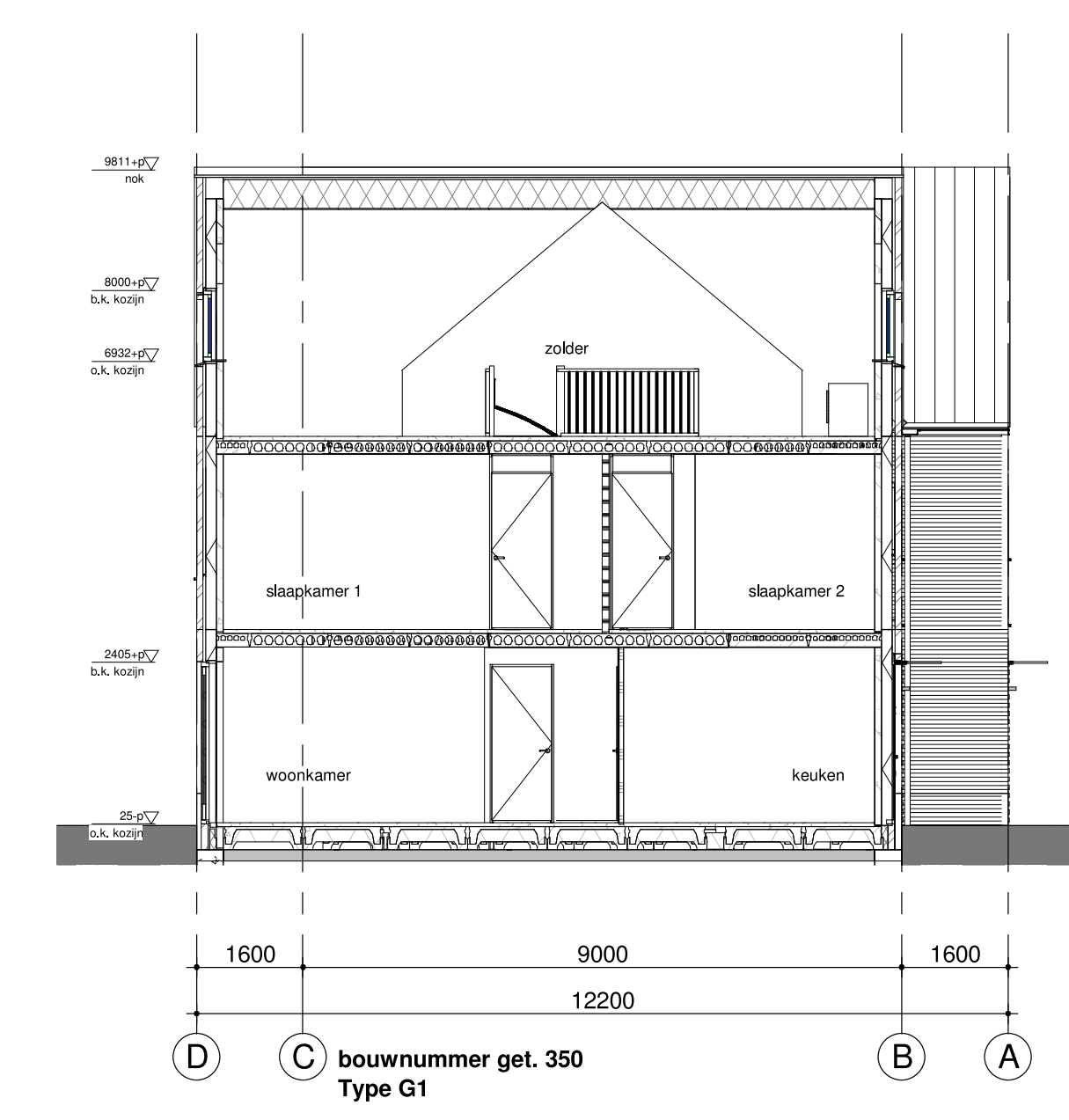
doorsnede A-A 1:100
