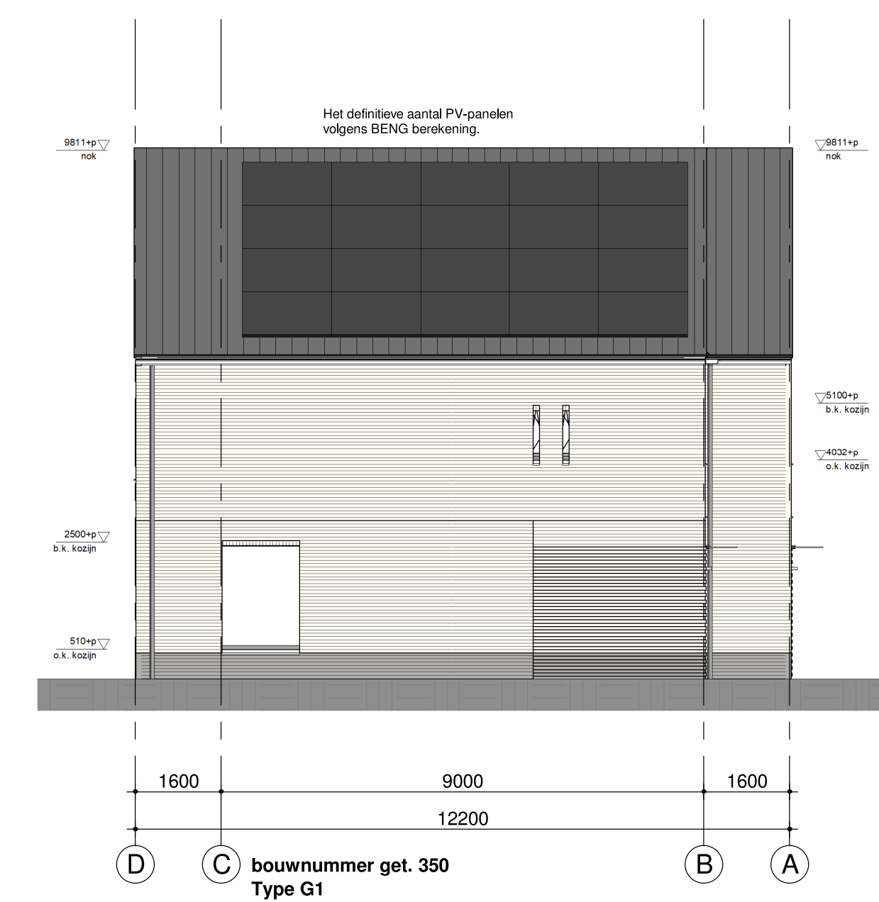
linkerzijgevel 1:100
