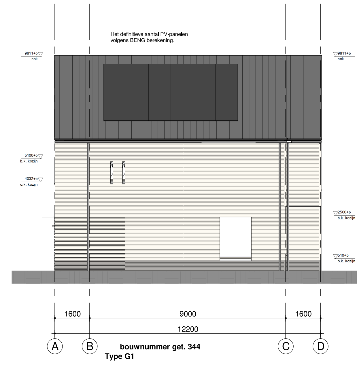
rechterzijgevel 1:100
