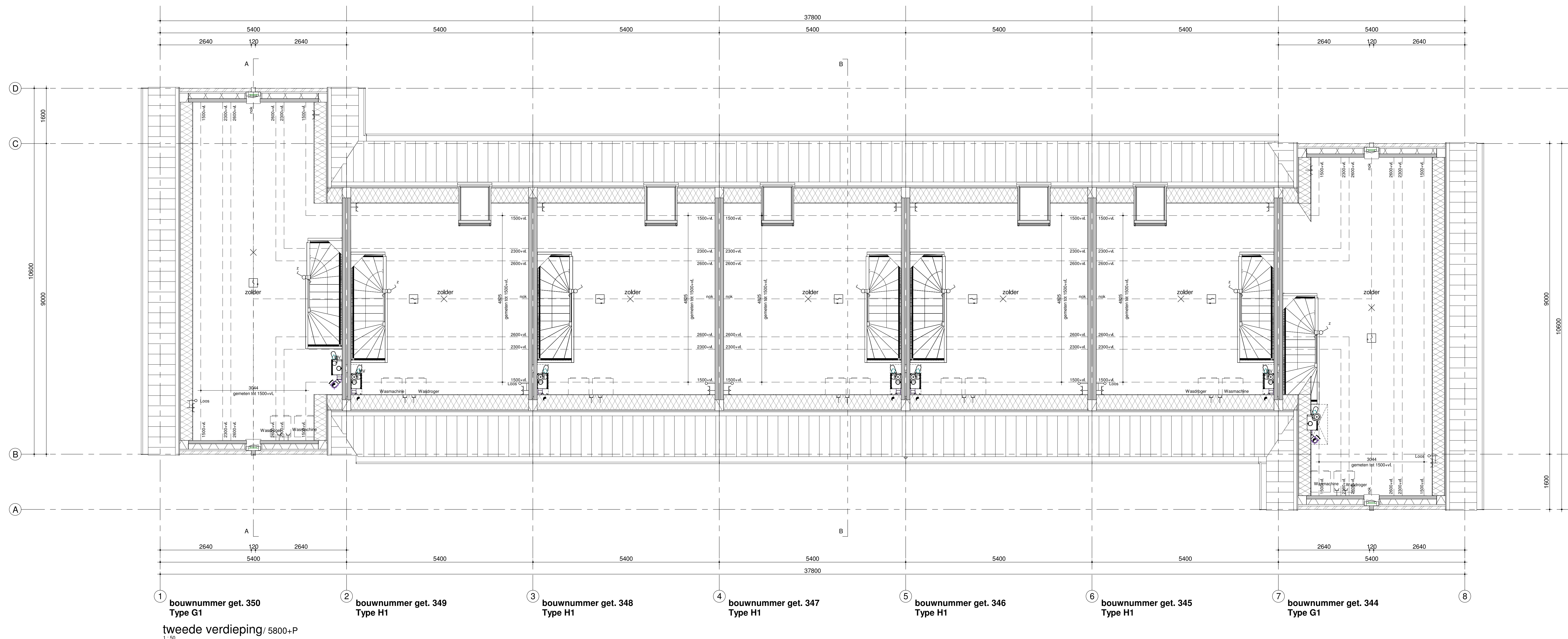
tweede verdieping / 5800+P 1:50
