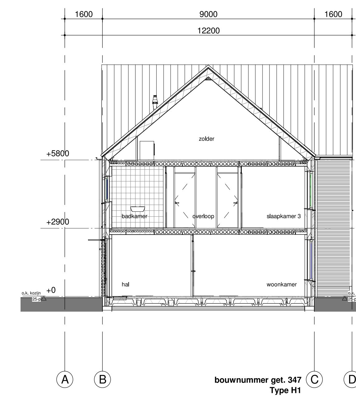
doorsnede B-B 1:100
