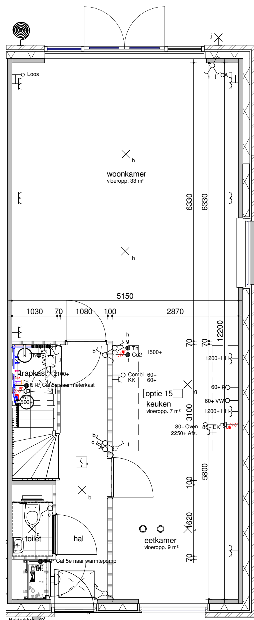
bouwnummer get. 244, 251 begane grond - optie keuken midden 1:50
