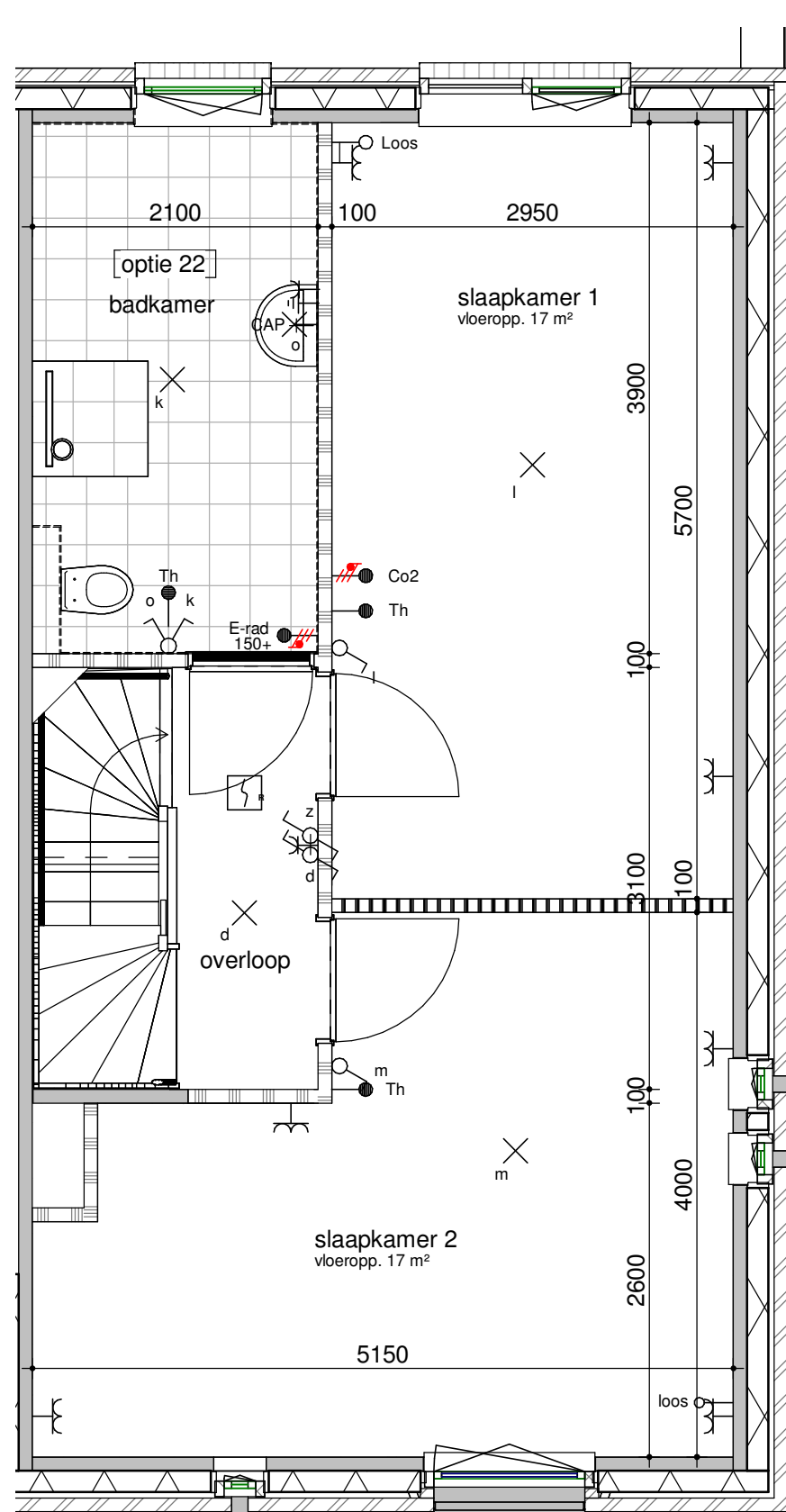
bouwnummer get. 244, 251 eerste verdieping - badkamer achter 1:50
