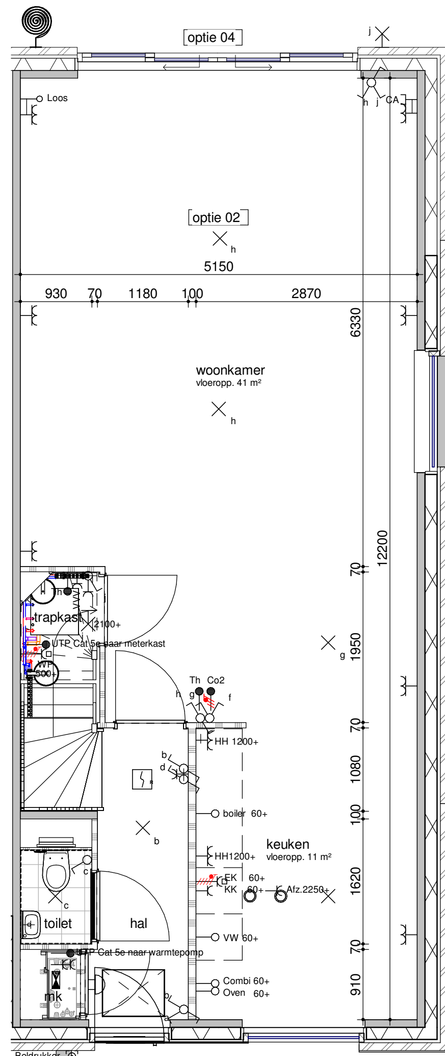
bouwnummer get. 244, 251 begane grond - optie 2400 1:50
