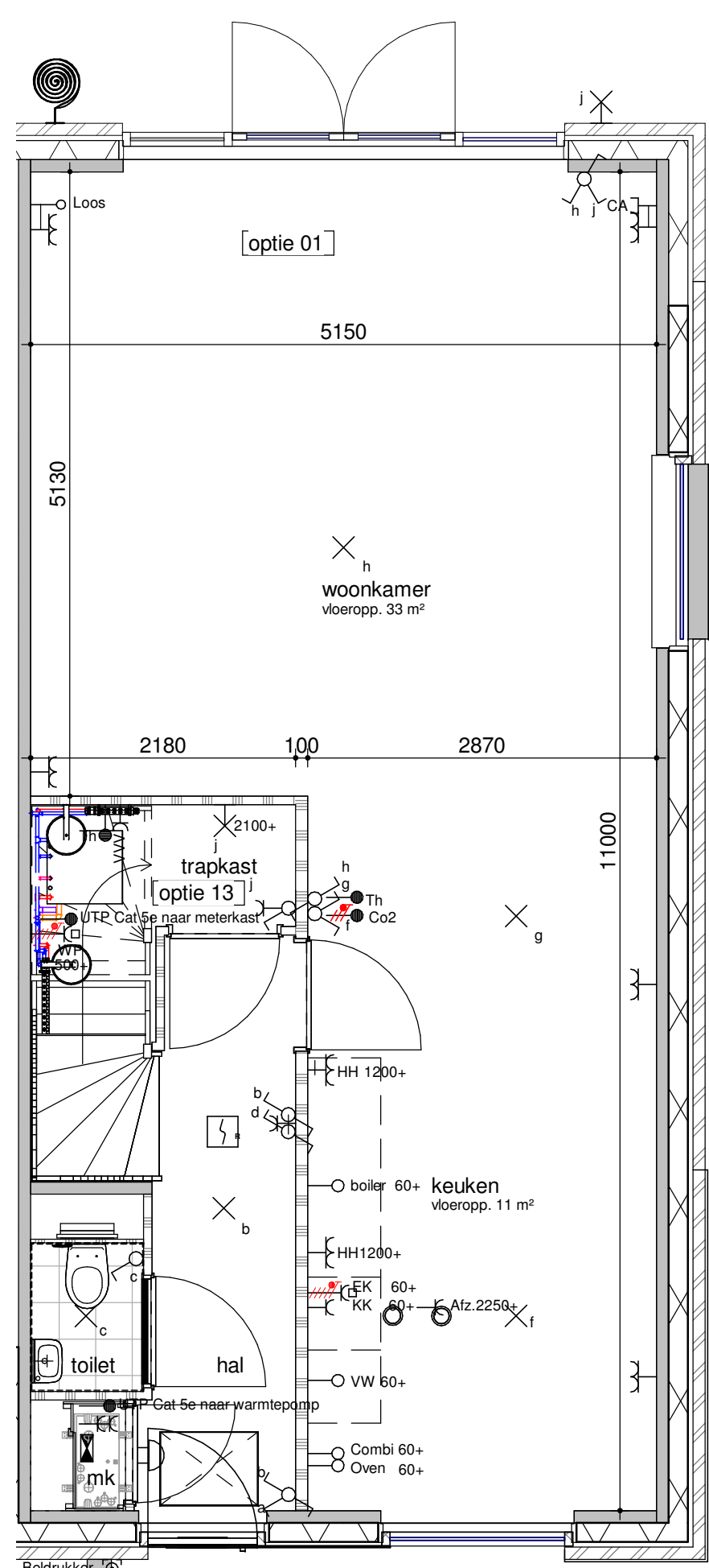
bouwnummer get. 244, 251 begane grond - optie 1200 1:50
