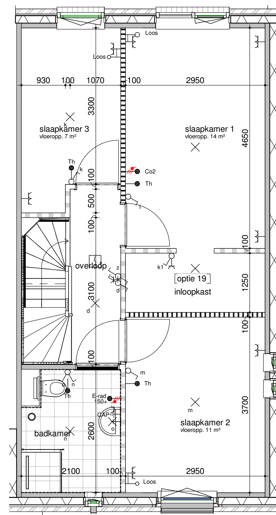
bouwnummer get. 244, 251 eerste verdieping - inloopkast 1:50
