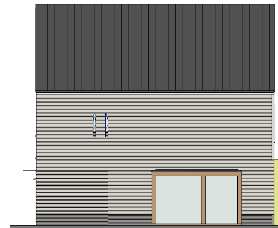
zijgevel - erker 1:100
