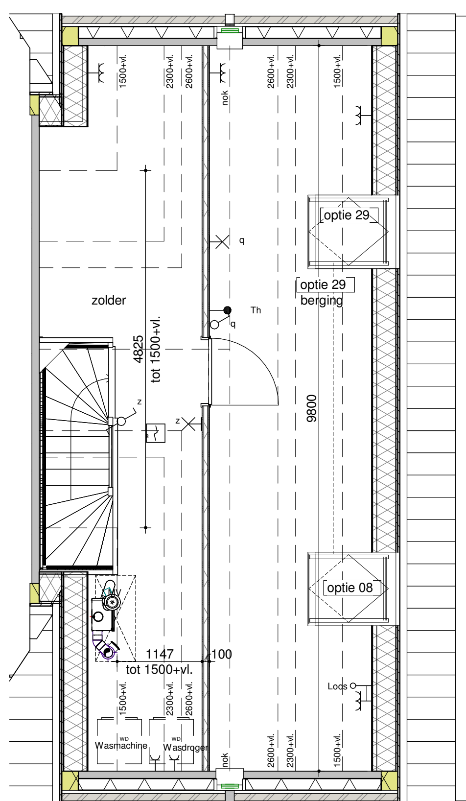
bouwnummer get. 244, 251 tweede verdieping - zolderindeling 1:50
