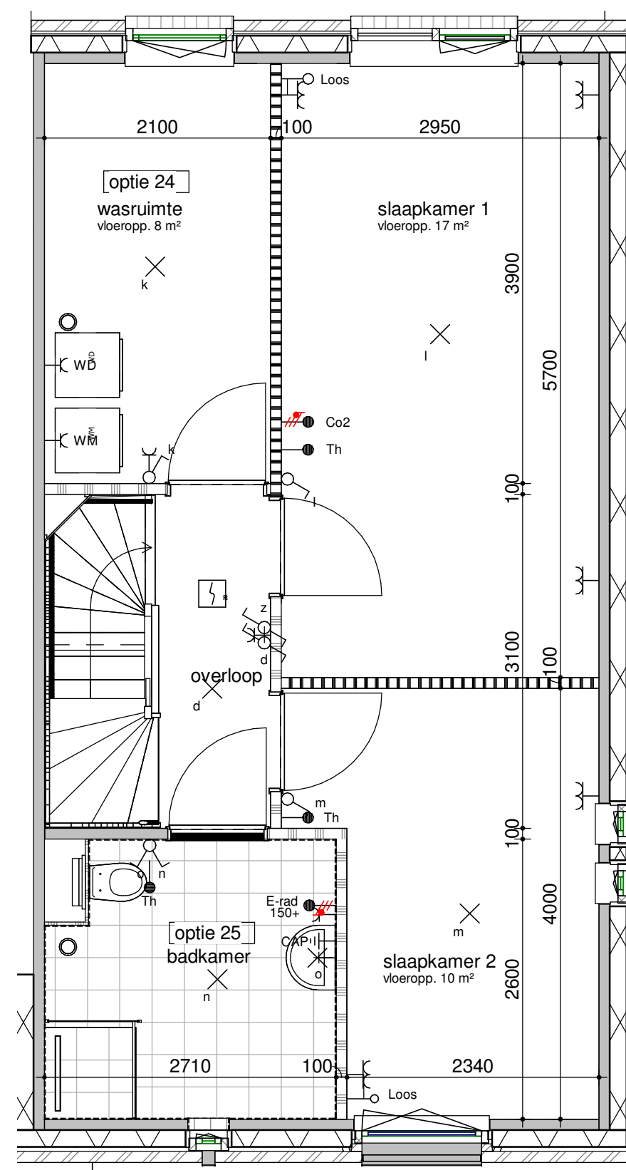
bouwnummer get. 244, 251 eerste verdieping - vergrote badkamer 1:50
