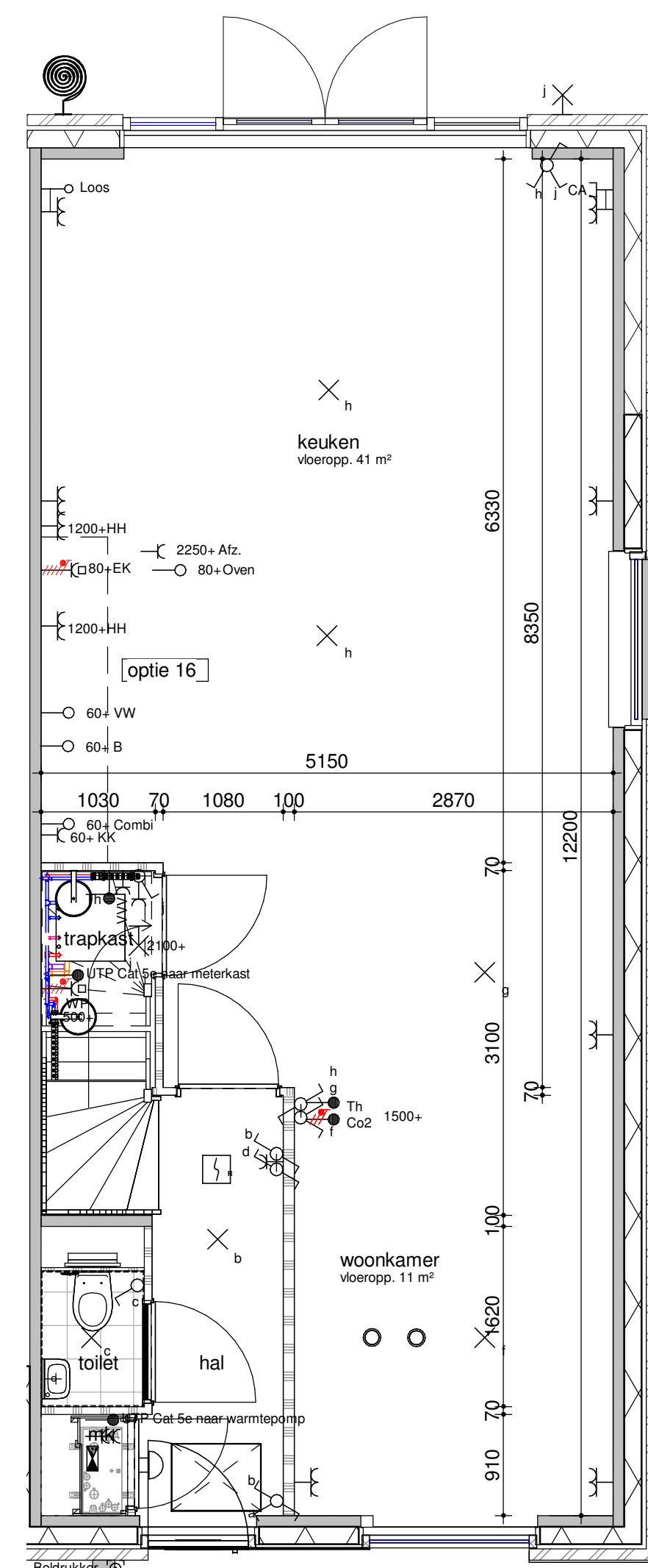
bouwnummer get. 244, 251 begane grond - optie keuken achter 1:50
