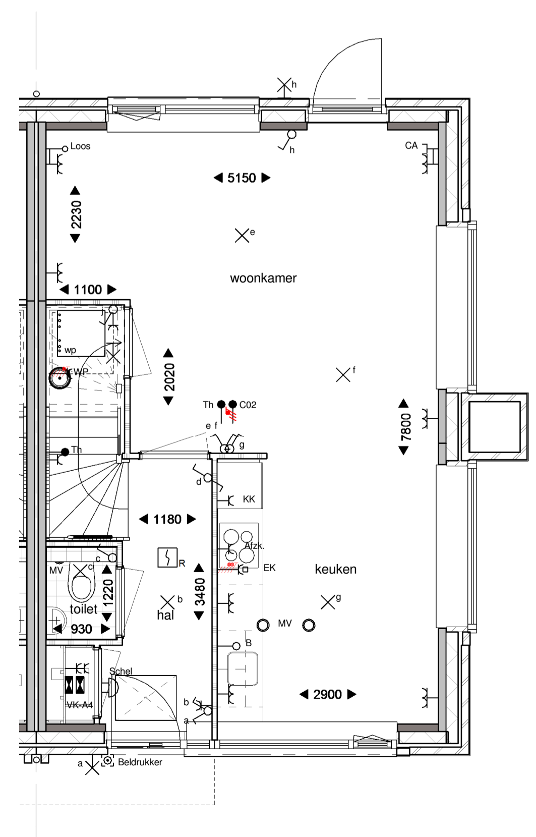
Begane grond
