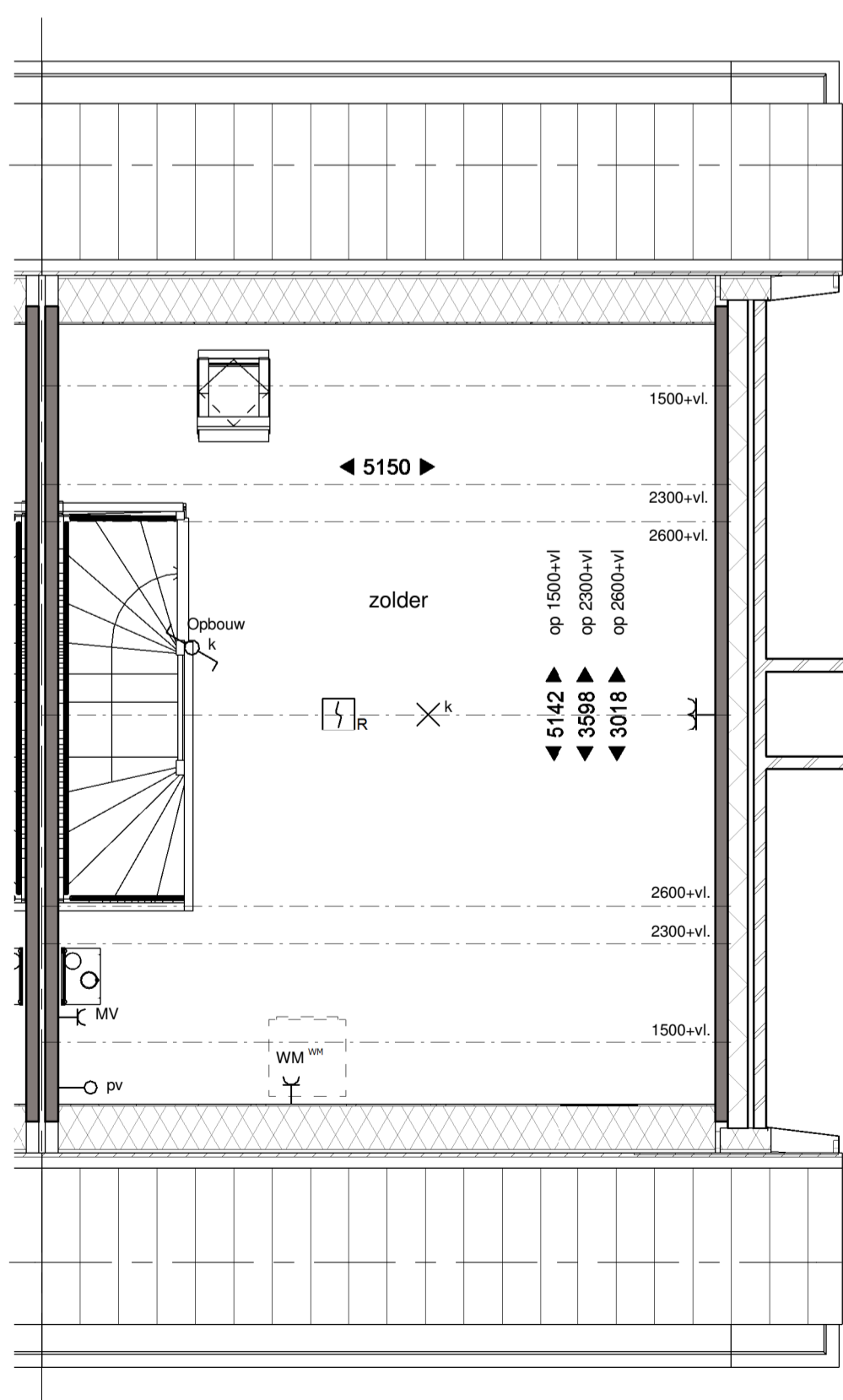
Tweede verdieping
