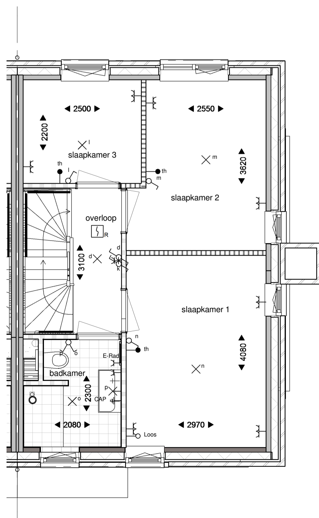
Eerste verdieping
