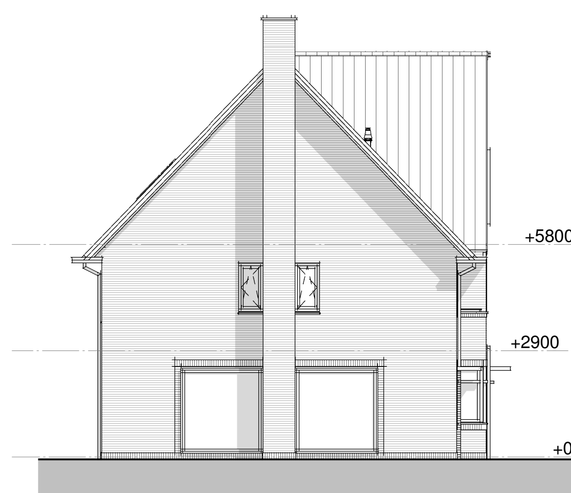
Linkergevel
