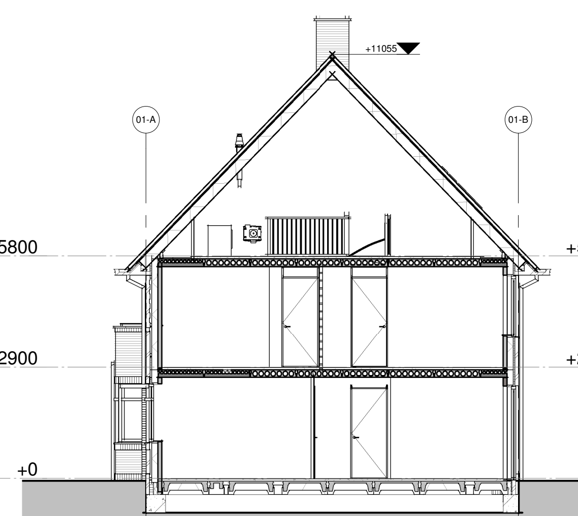
Doorsnede 01-A-A
