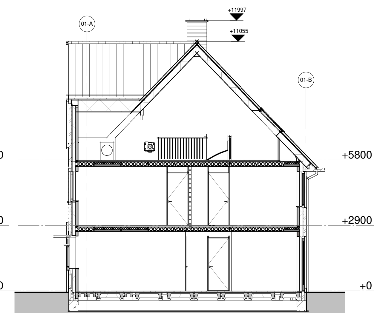
Doorsnede 01-C-C
