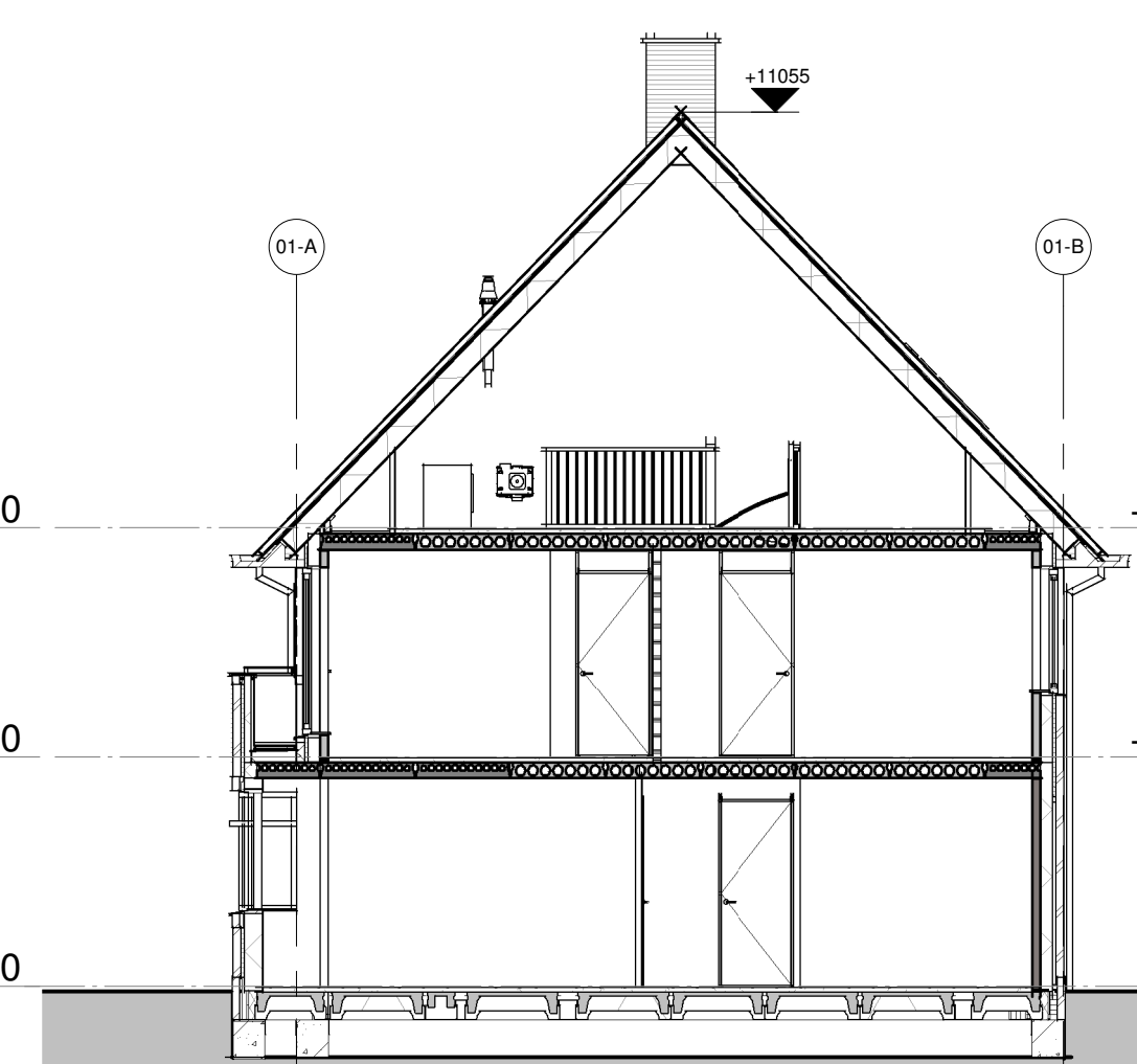
Doorsnede 01-B-B
