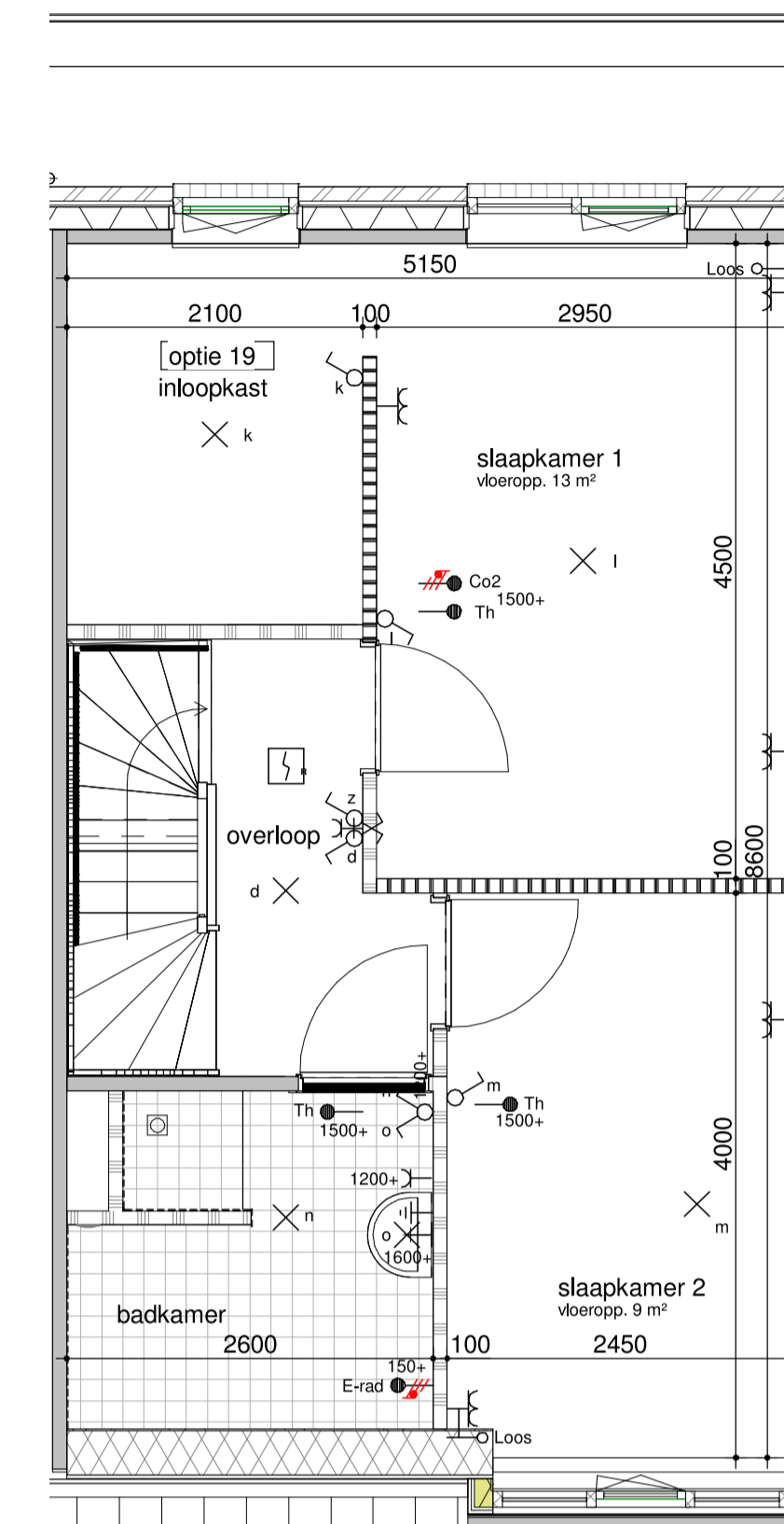
bouwnummer 352, 353, 354, 355, 414, 415, 416, 417 eerste verdieping - inloopkast 1:50
