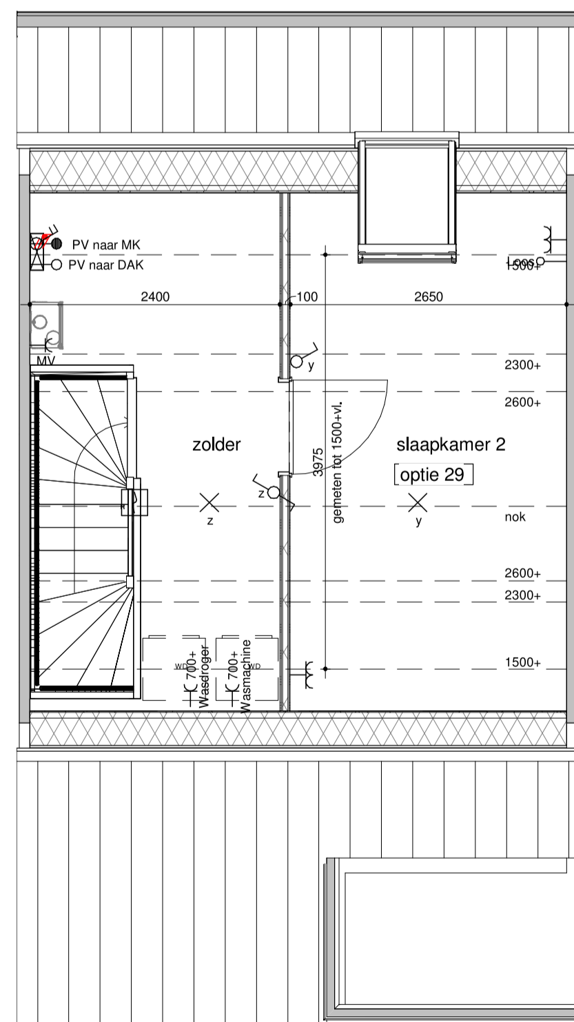
bouwnummer 352, 353, 354, 355, 414, 415, 416, 417 tweede verdieping - zolderindeling 1:50
