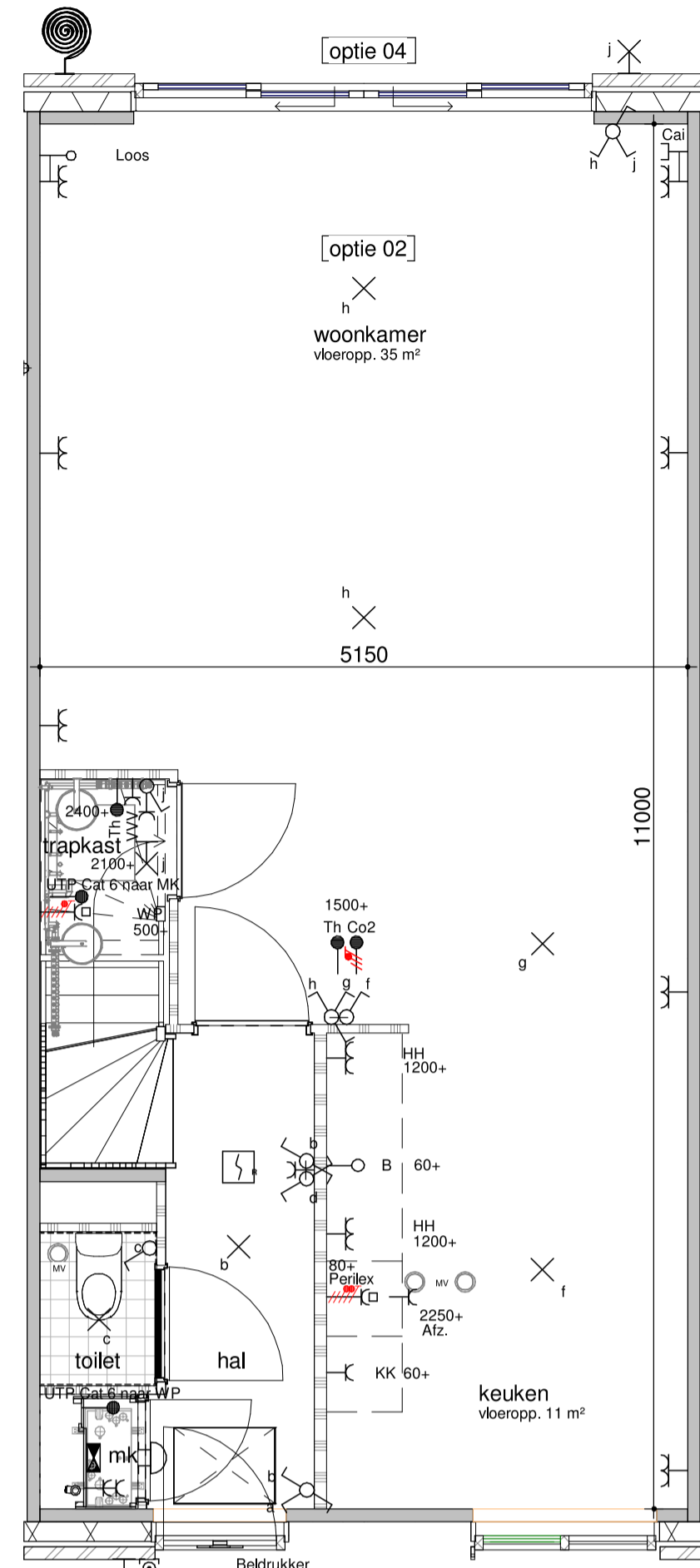
bouwnummer 352, 353, 354, 355, 414, 415, 416, 417 begane grond - optie 2400 1:50
