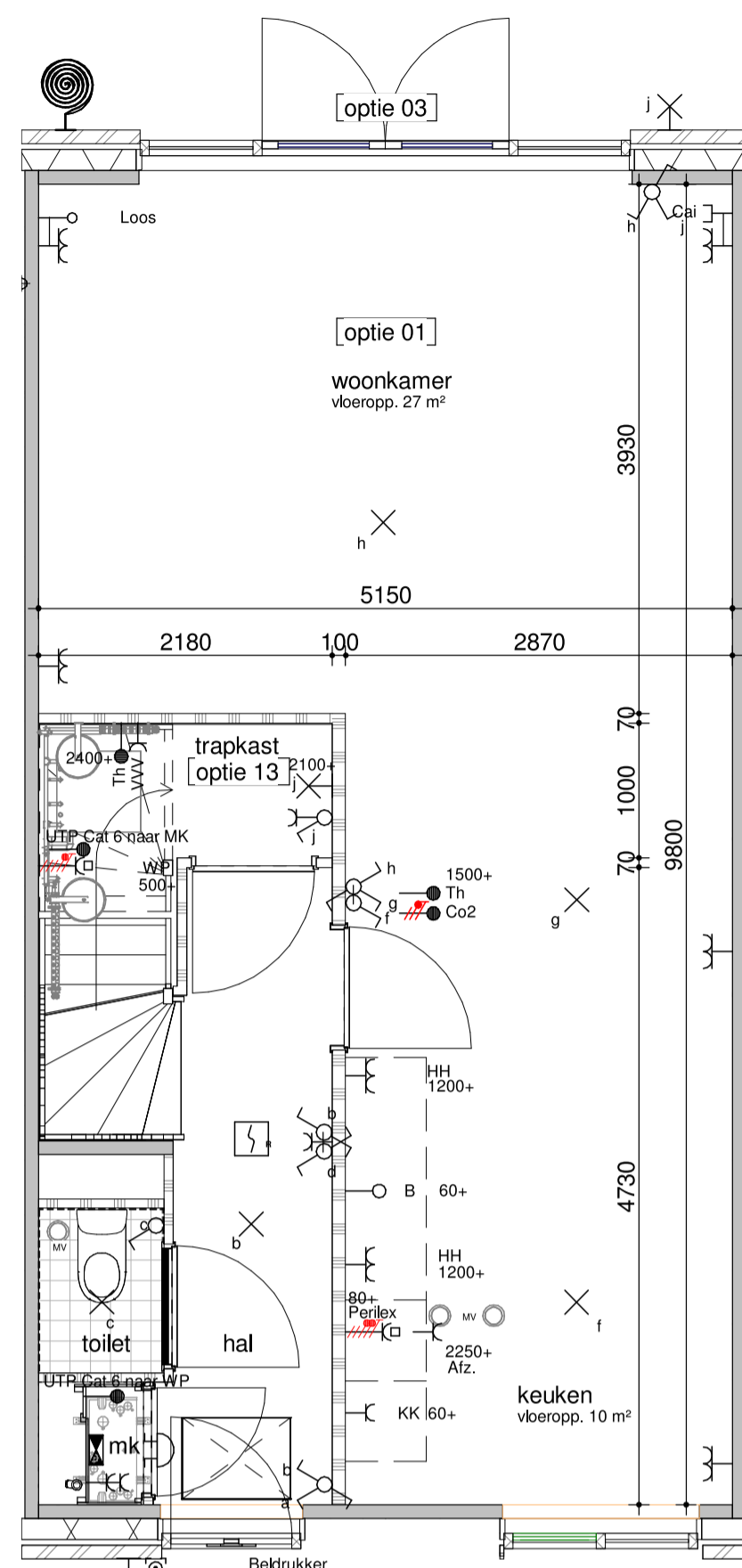
bouwnummer 352, 353, 354, 355, 414, 415, 416, 417 begane grond - optie 1200 1:50
