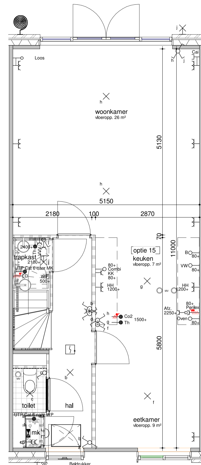
bouwnummer 352, 353, 354, 355, 414, 415, 416, 417 begane grond - optie middenkeuken 1:50
