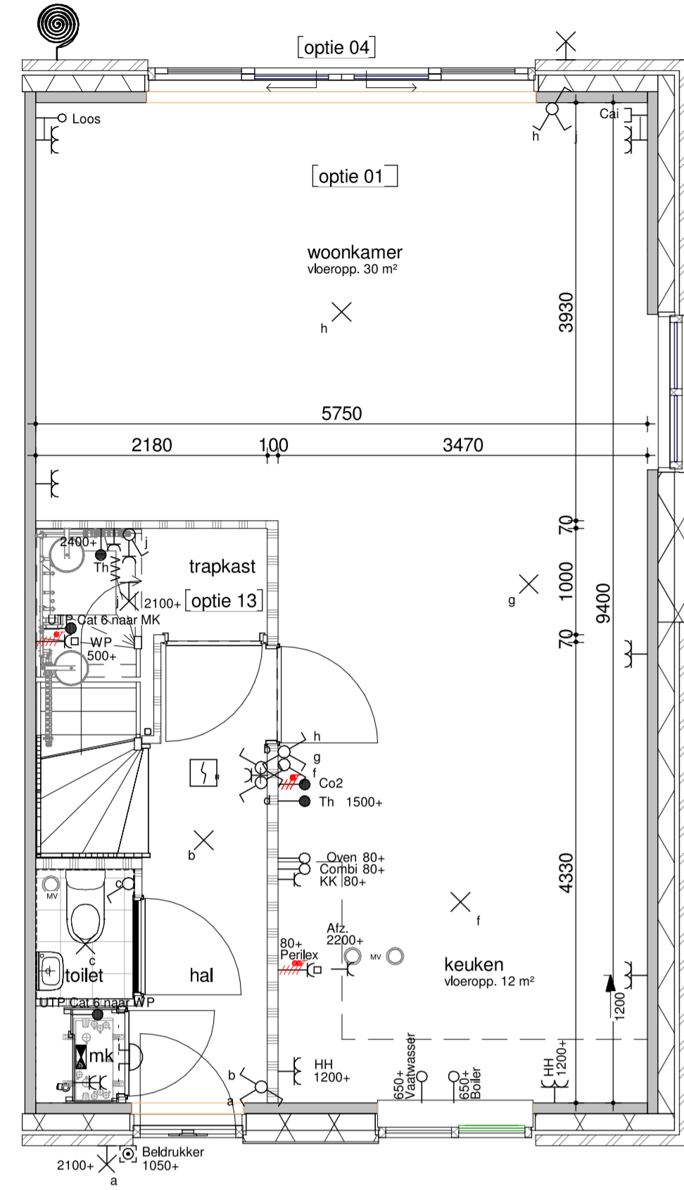
bwnr. 412 (gespiegeld) begane grond - optie 1200 1:50
