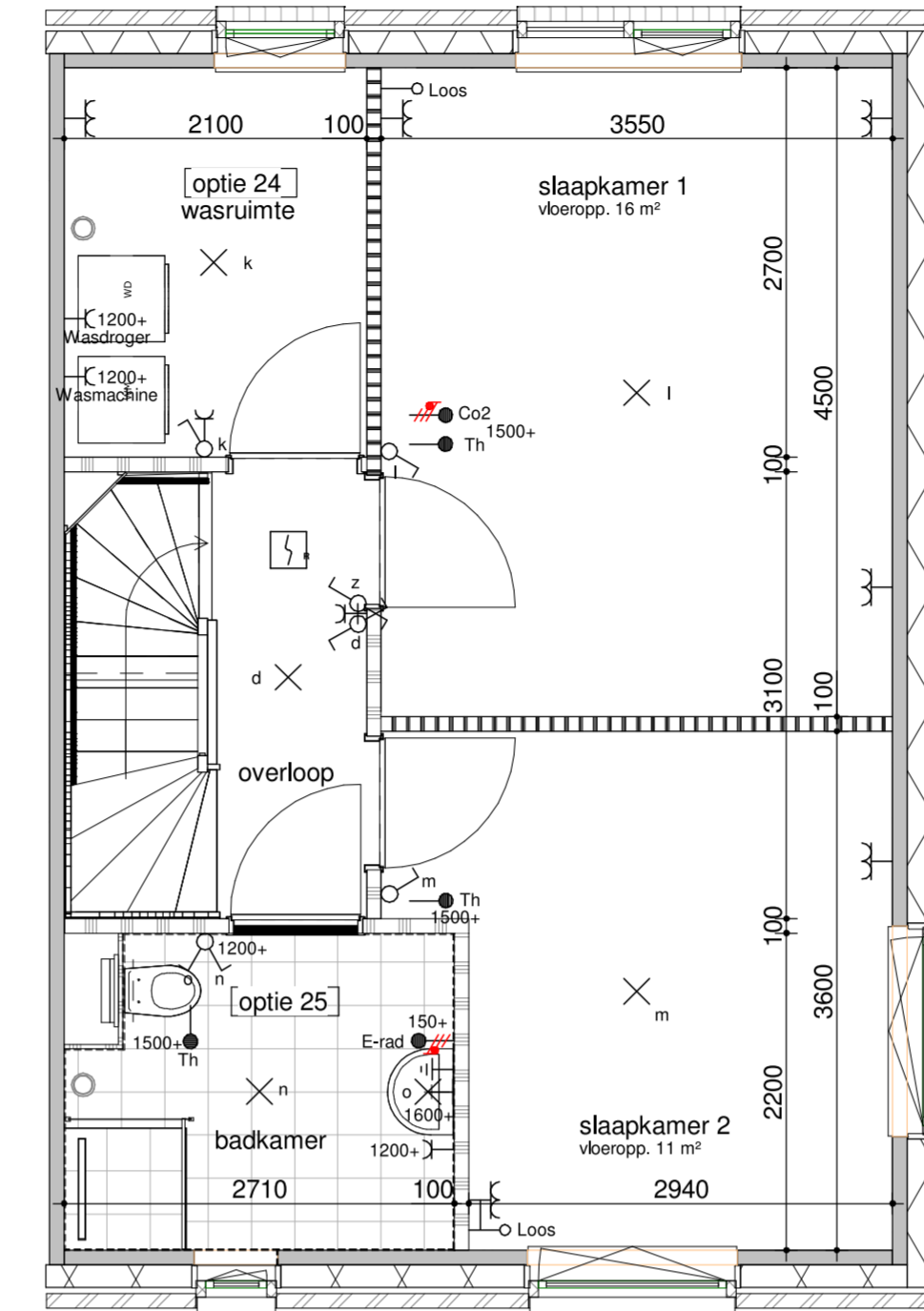
bwnr. 412 (gespiegeld) eerste verdieping - vergrote badkamer 1:50
