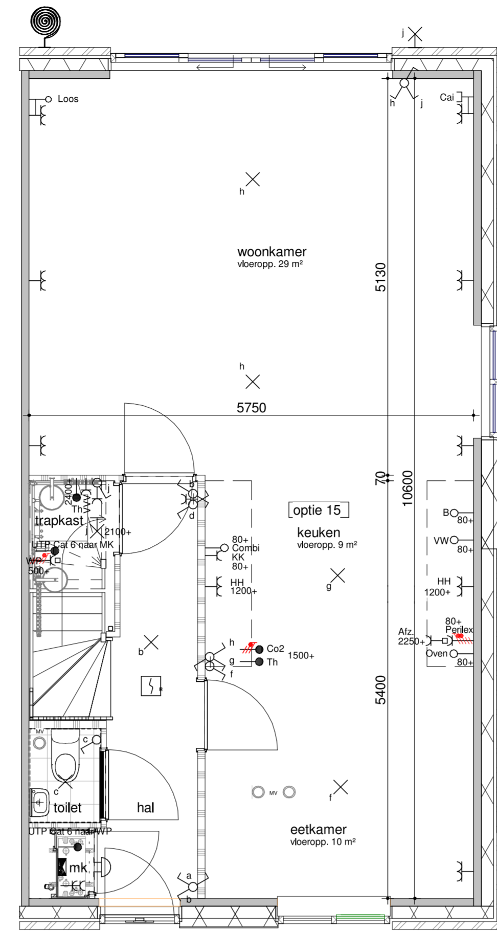
bwnr. 412 (gespiegeld) begane grond - optie middenkeuken 1:50
