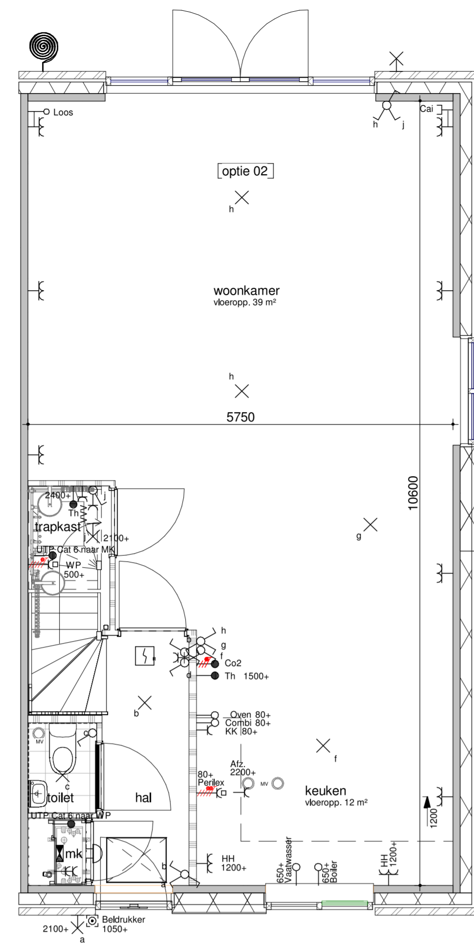
bwnr. 412 (gespiegeld) begane grond - optie 2400 1:50
