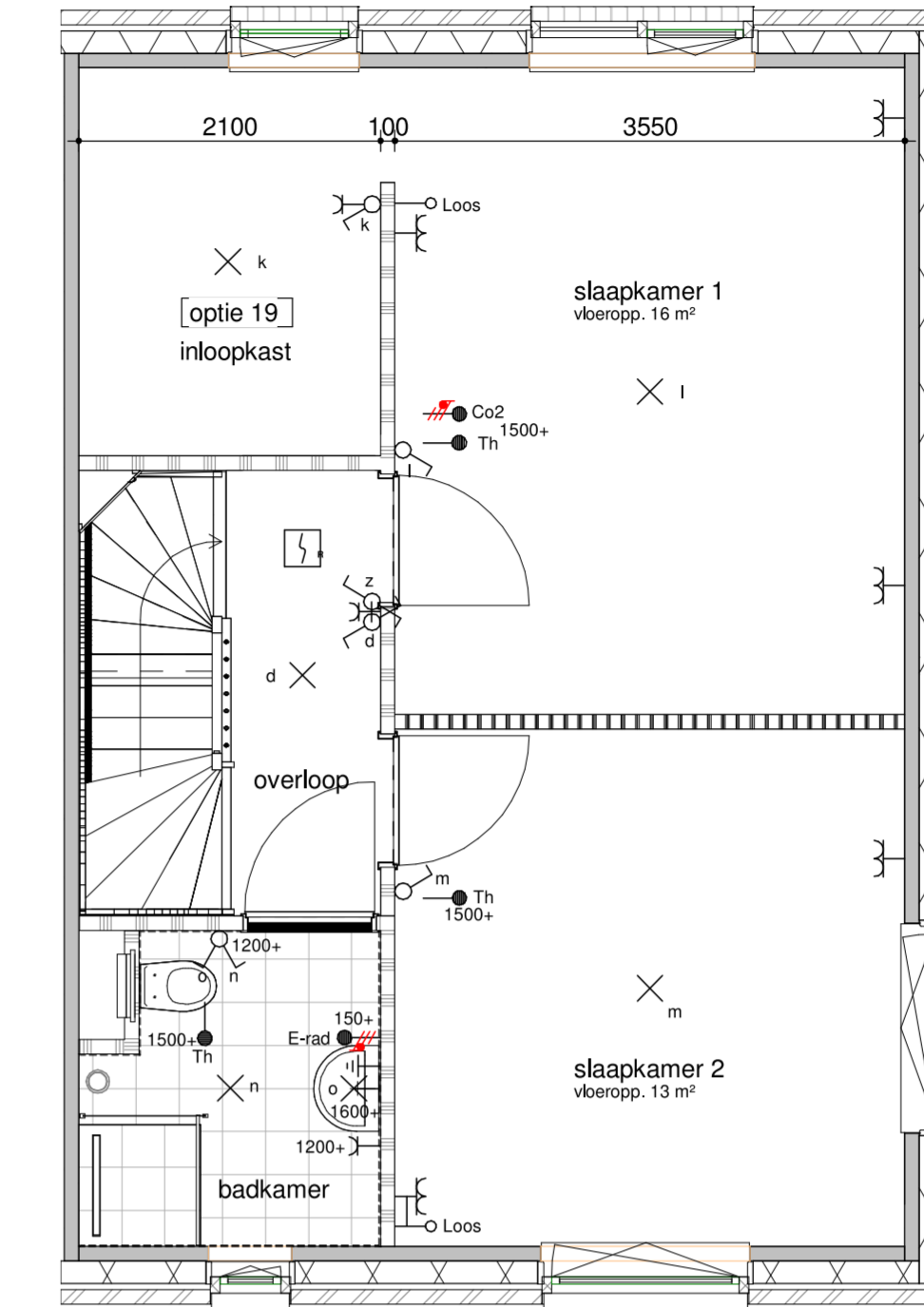
bwnr. 412 (gespiegeld) eerste verdieping - inloopkast 1:50
