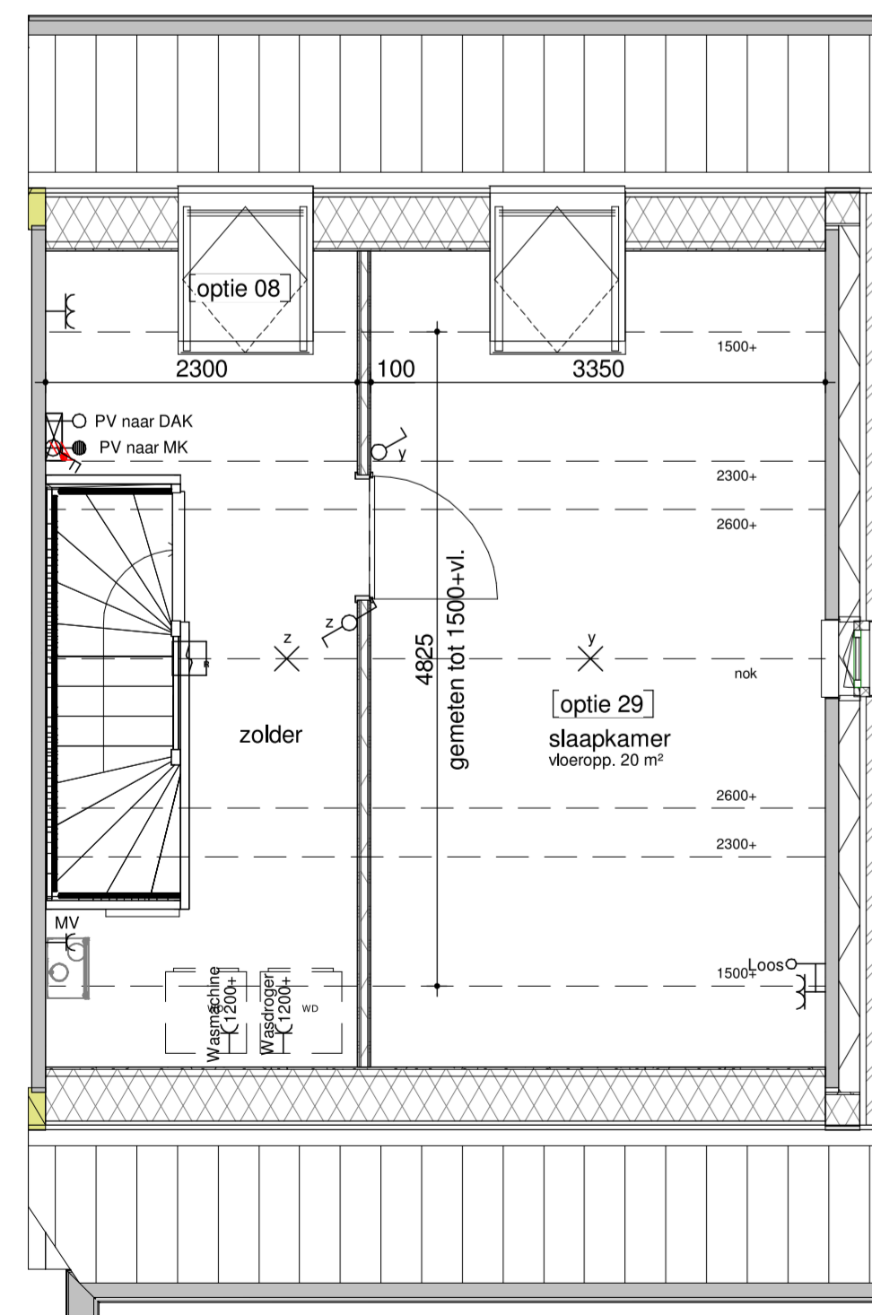
bwnr. 412 (gespiegeld) tweede verdieping - zolderindeling 1:50
