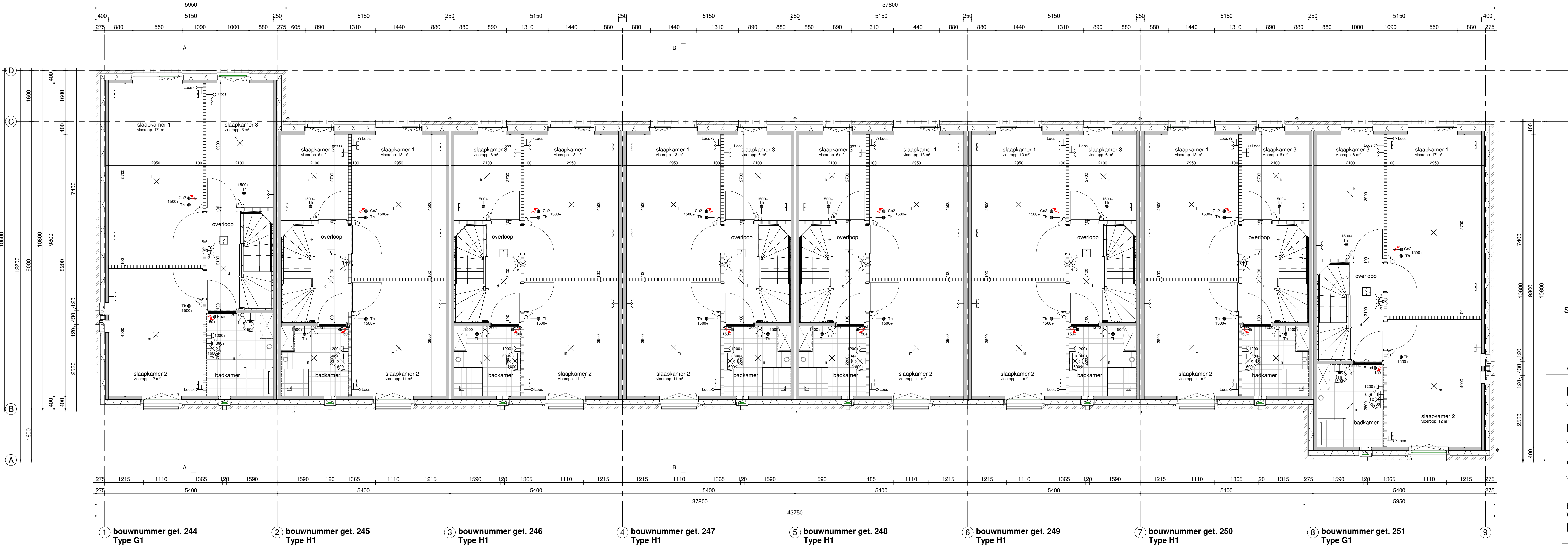
eerste verdieping 1:50
