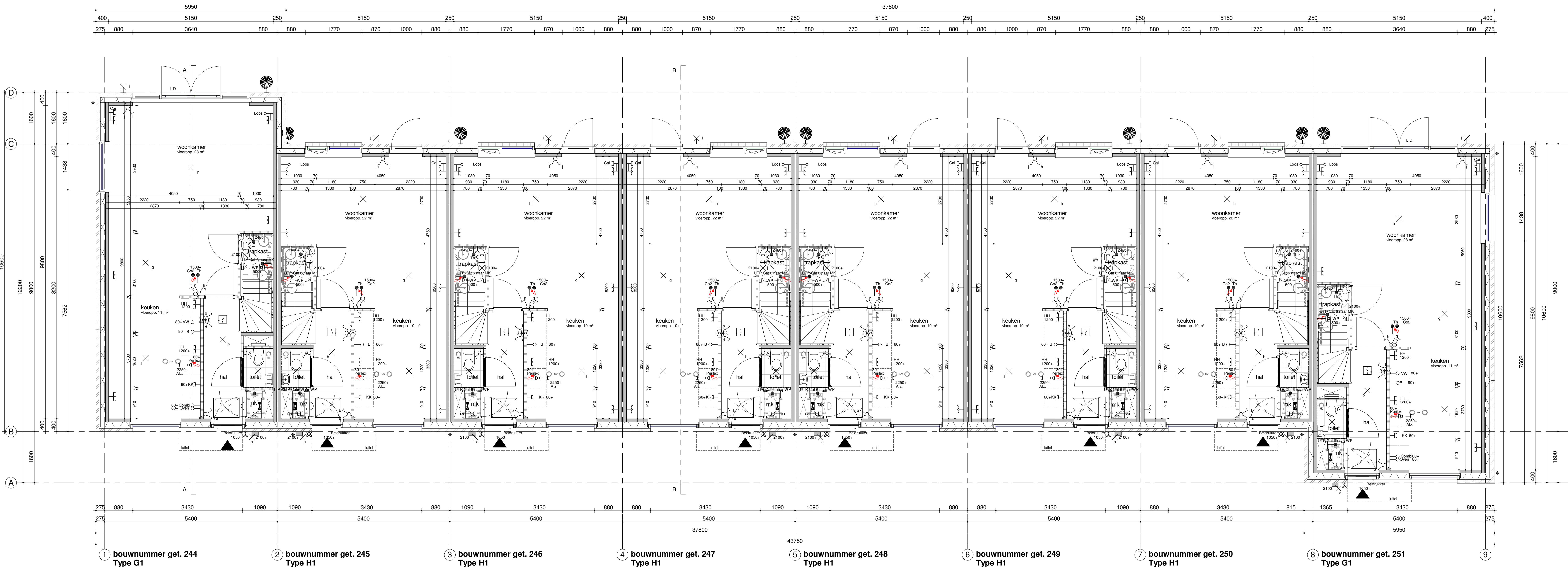
Begane grond 1:50
