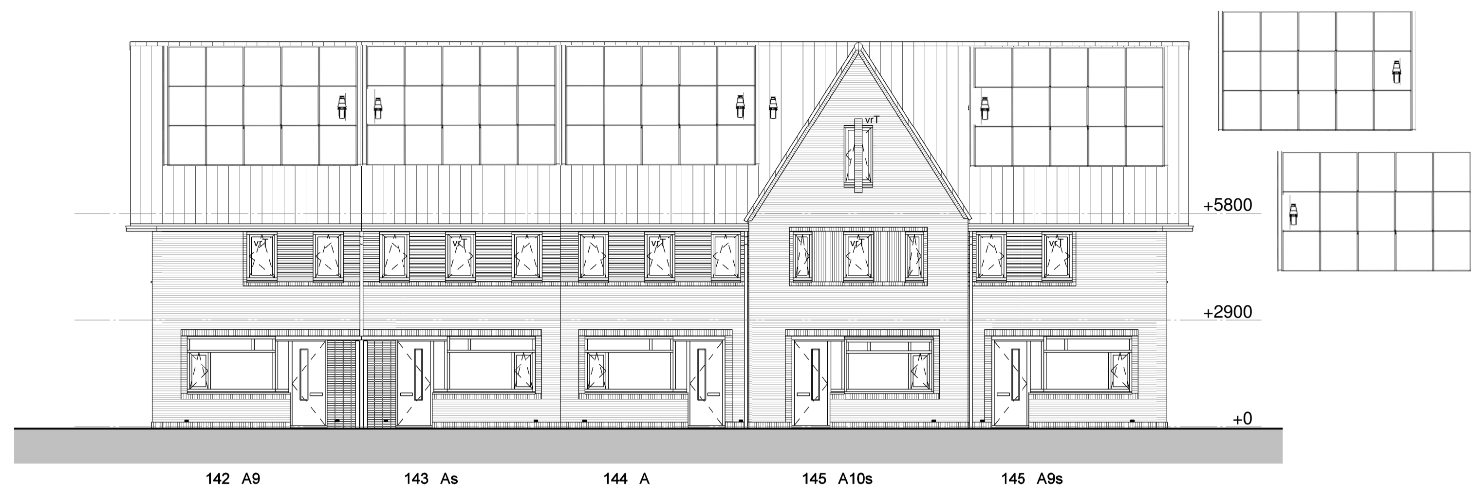
Voorgevel Blok 15 zonder dakkapel
