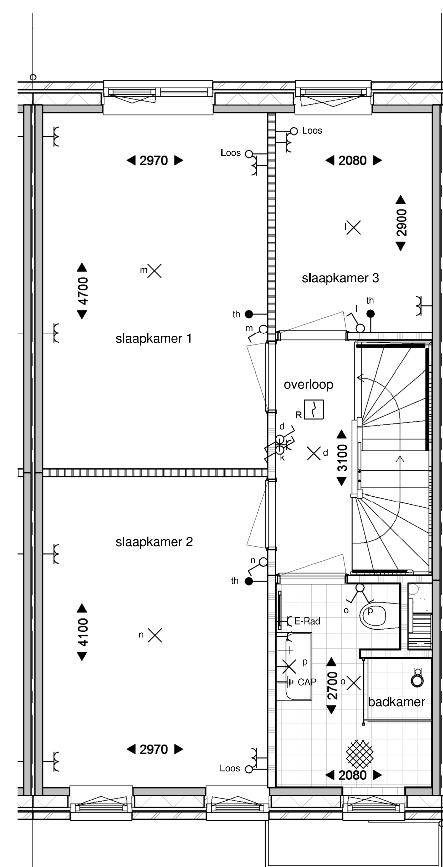
Eerste verdieping
