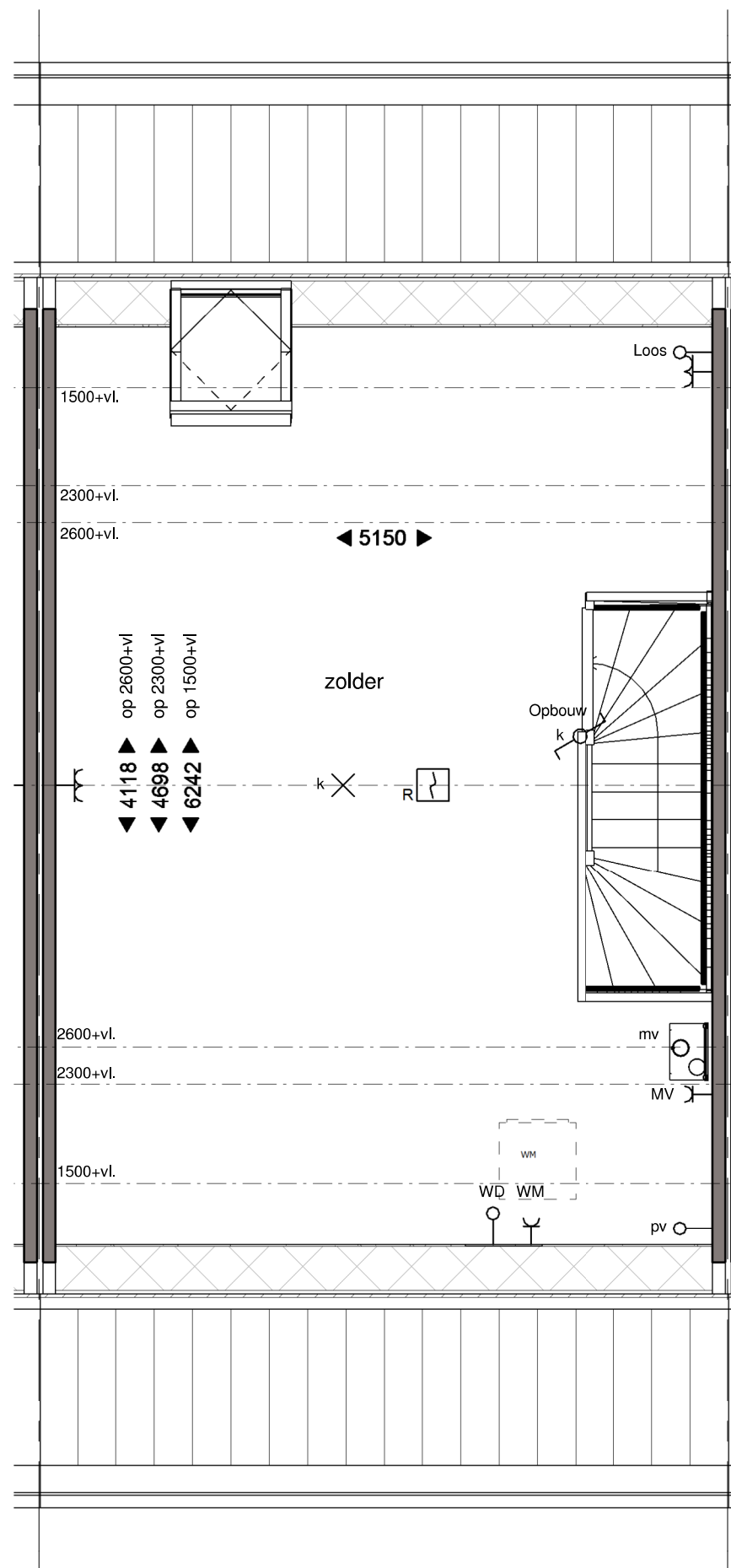
Tweede verdieping
