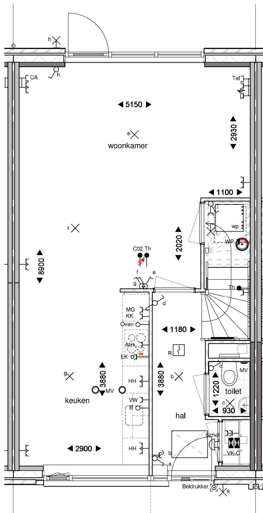
Begane grond
