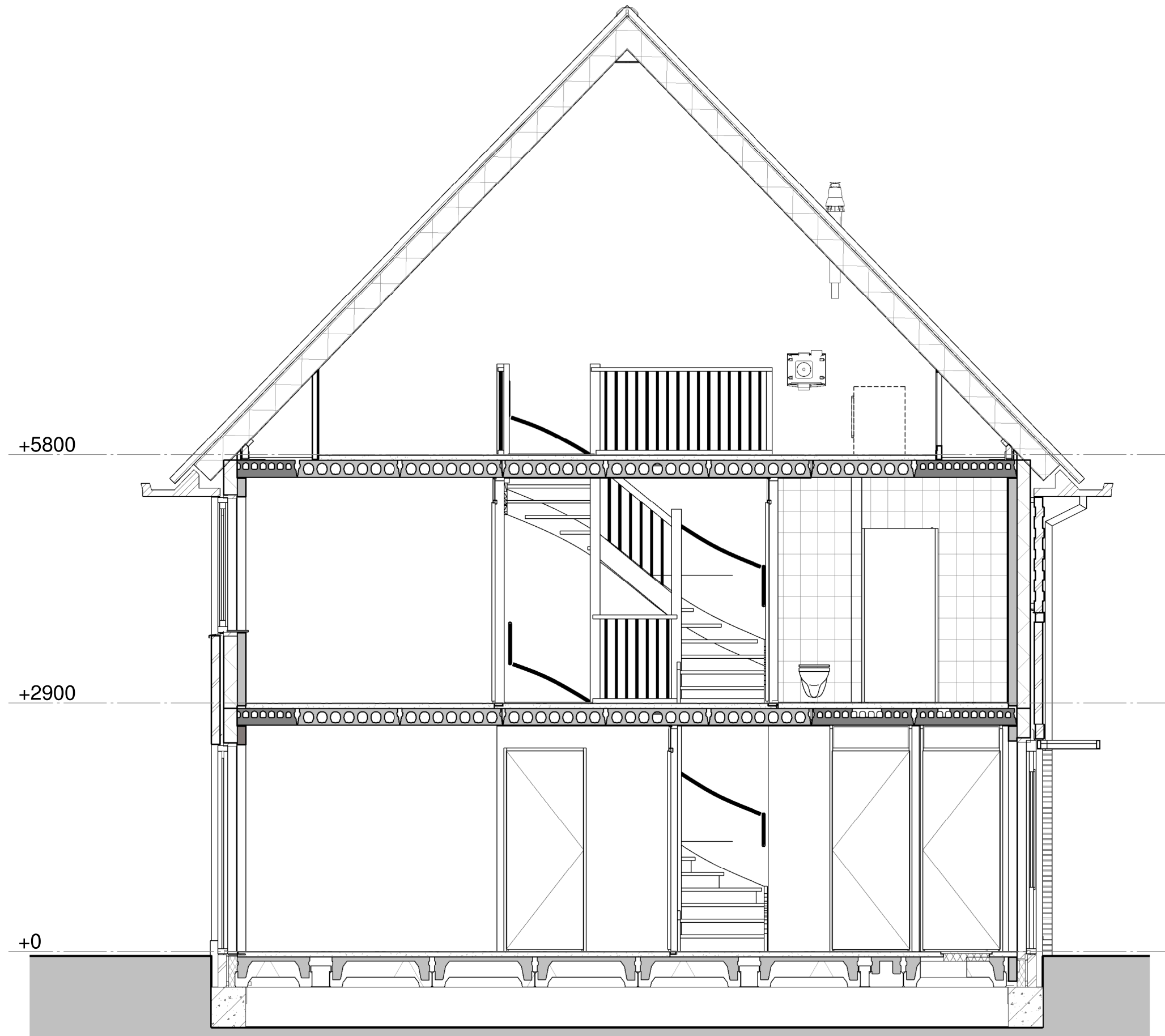
Doorsnede
