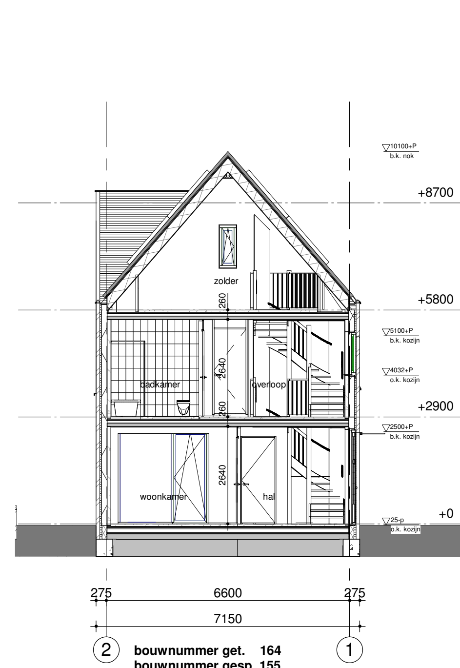
doorsnede AA 1:100
