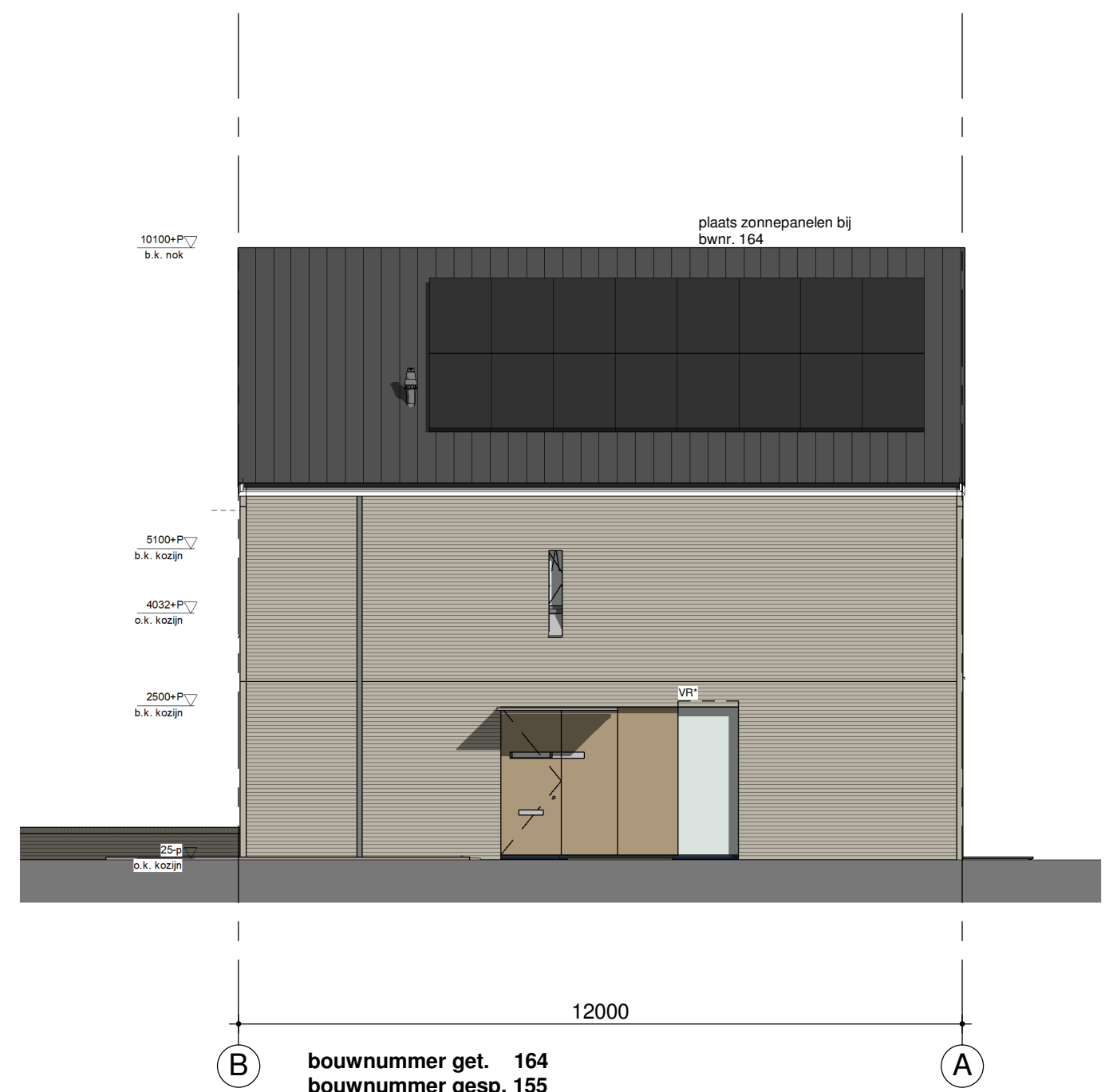
linker zijgevel 1:100
