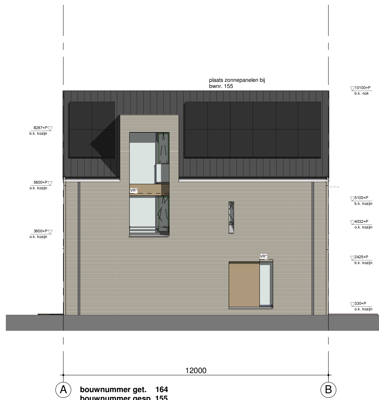
rechter zijgevel 1:100
