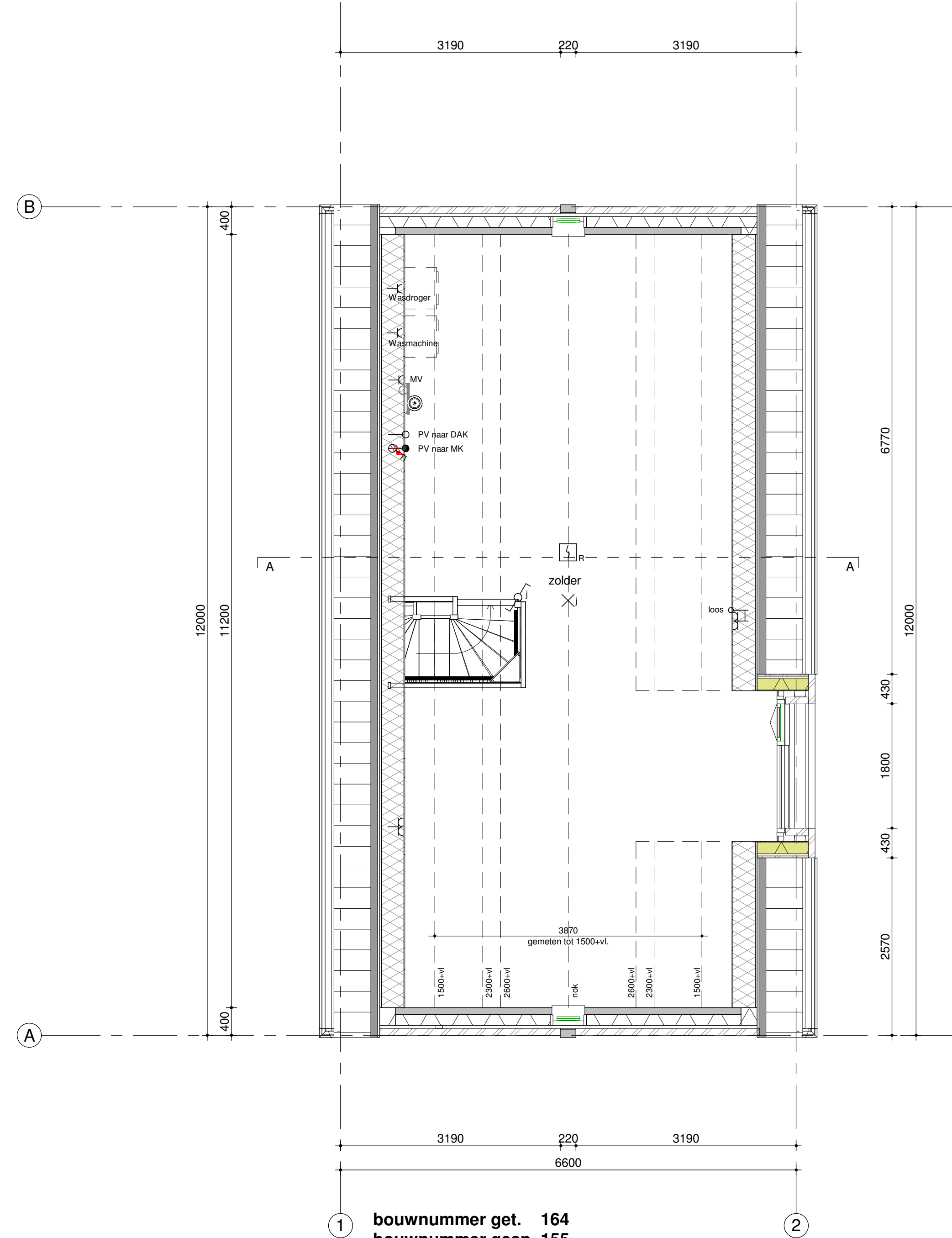
tweede verdieping / 5800+P 1:50
