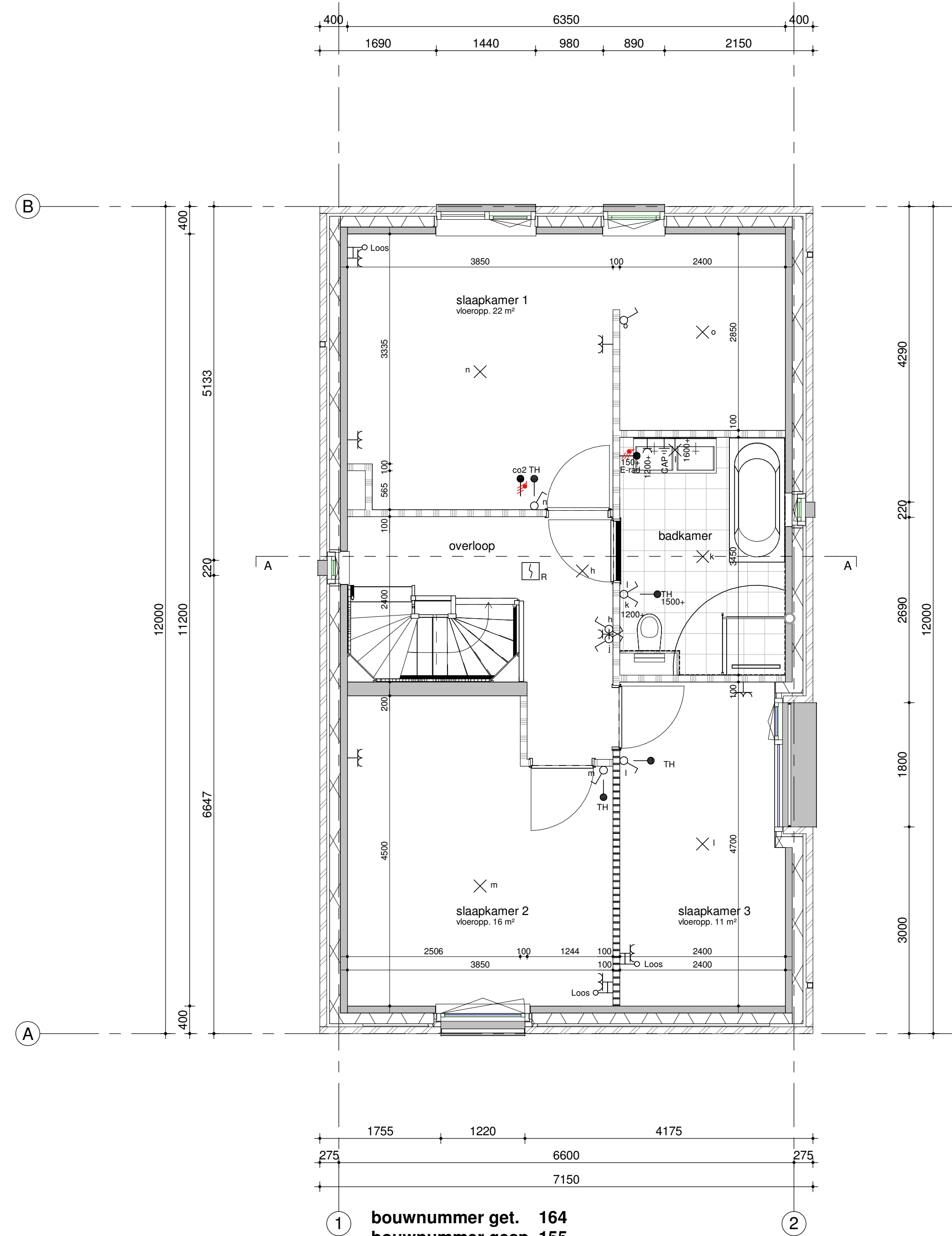
eerste verdieping / 2900+P 1:50
