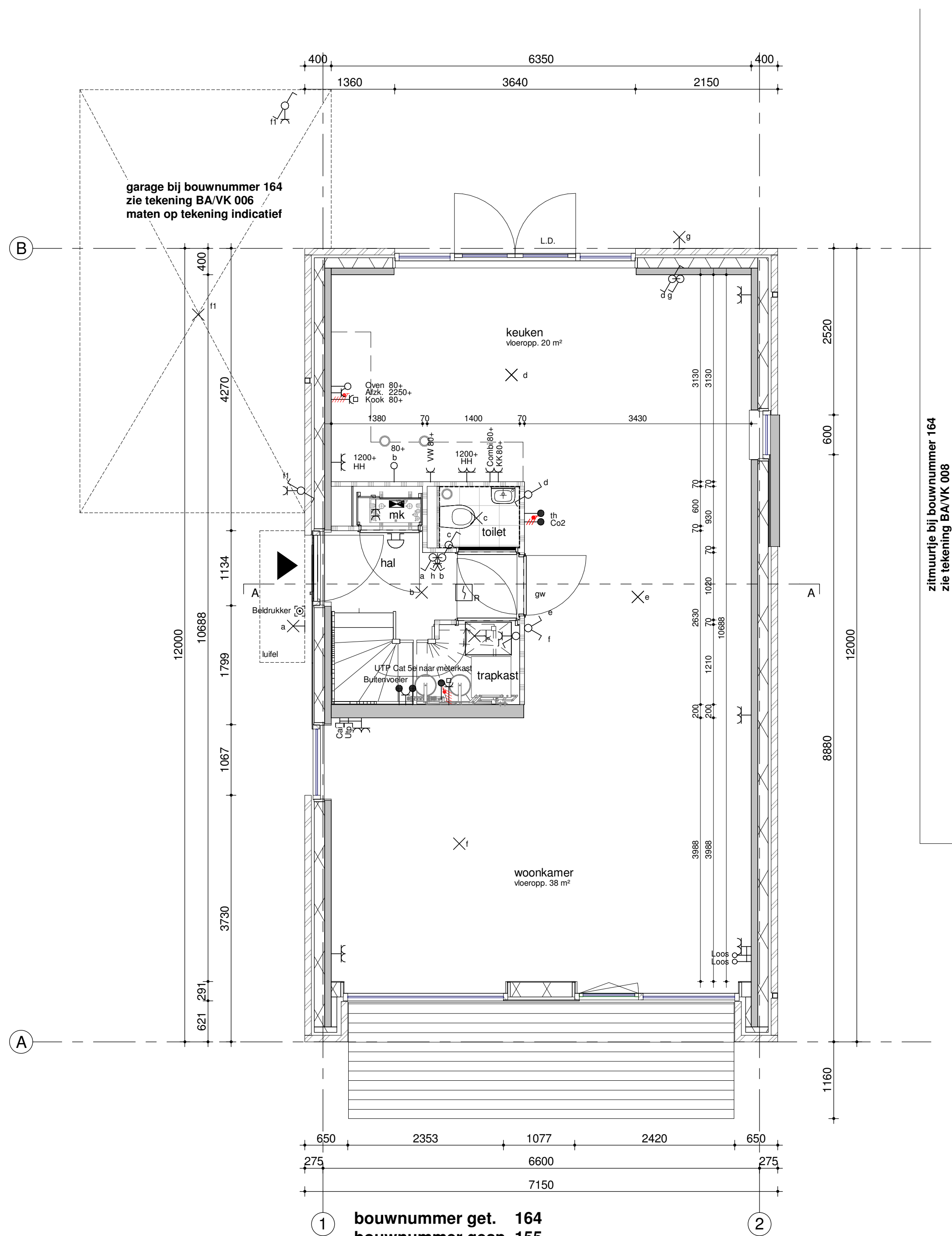
begane grond / PEIL=0 1:50
