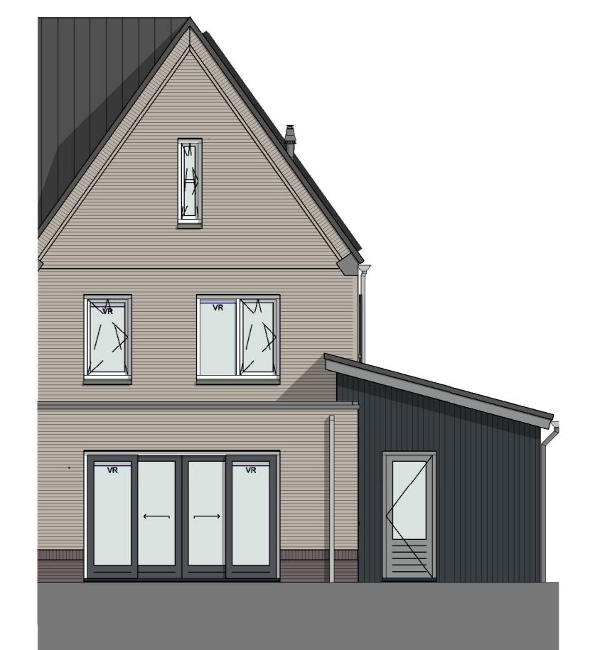
achtergevel - 1200 uitbouw + schuifpui 1:100
