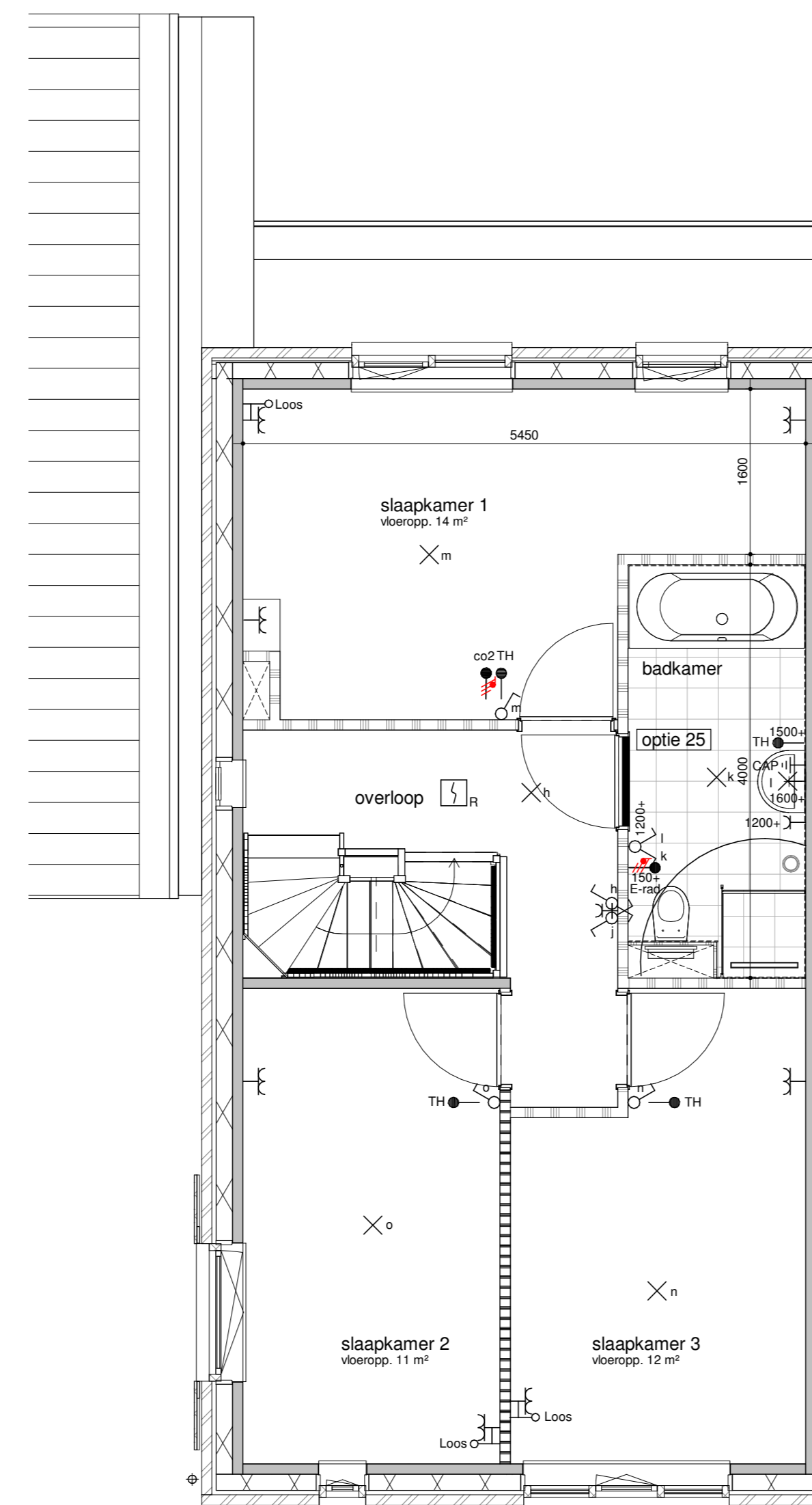
bouwnummer get. 242 eerste verdieping - vergrote badkamer 1:50
