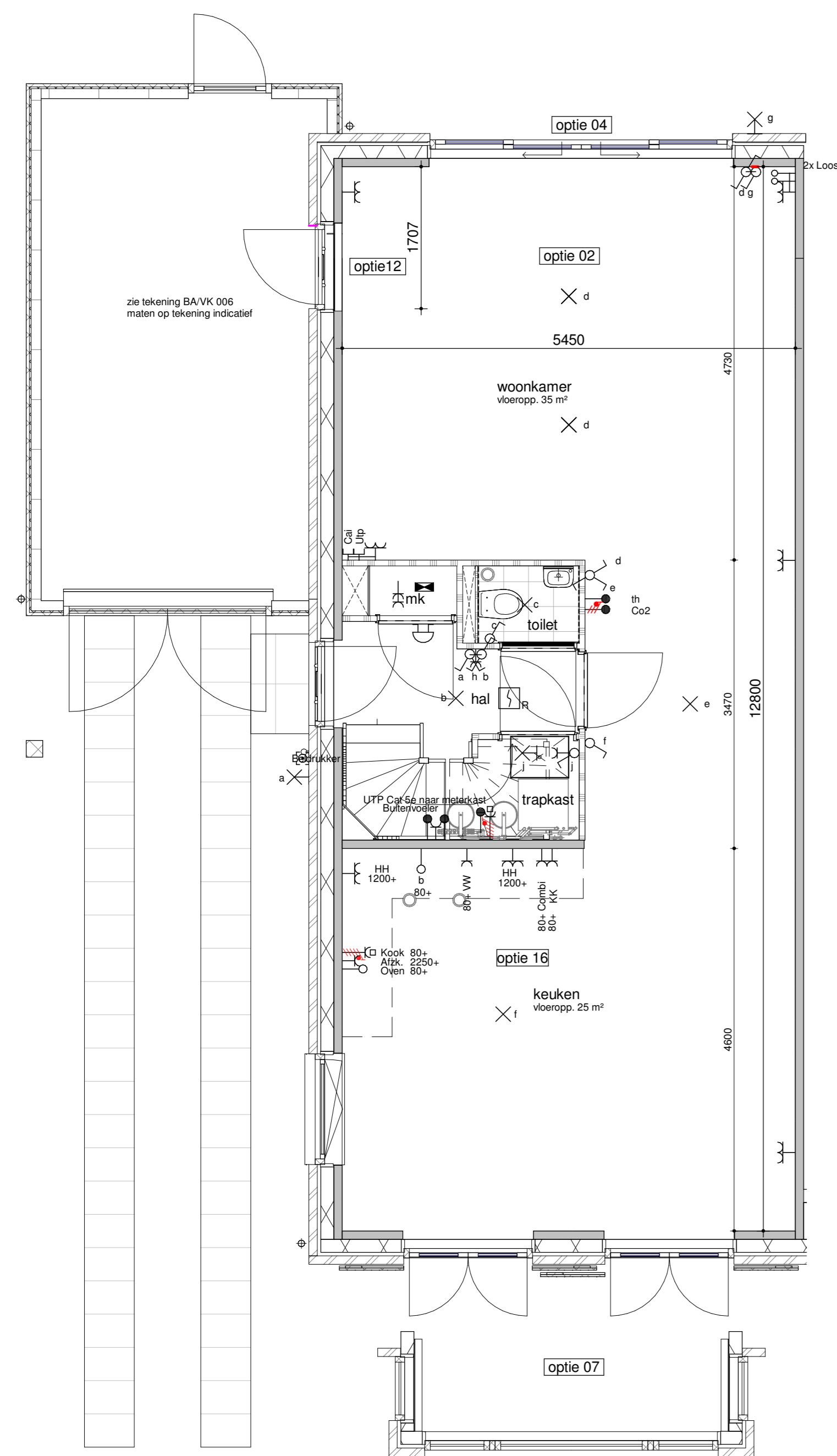
bouwnummer get. 242 begane grond - optie 240 1:50
