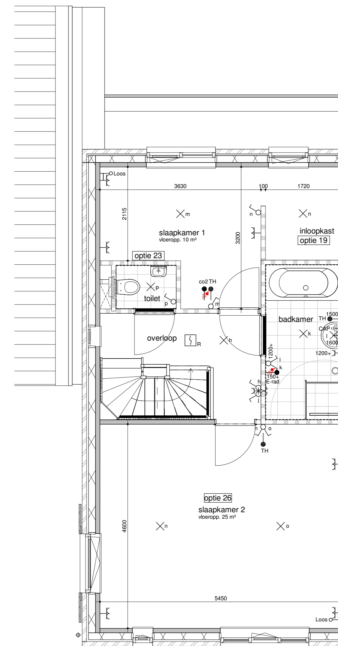
bouwnummer get. 242 eerste verdieping - samenvoegen slaapkamer 2 en 3 1:50
