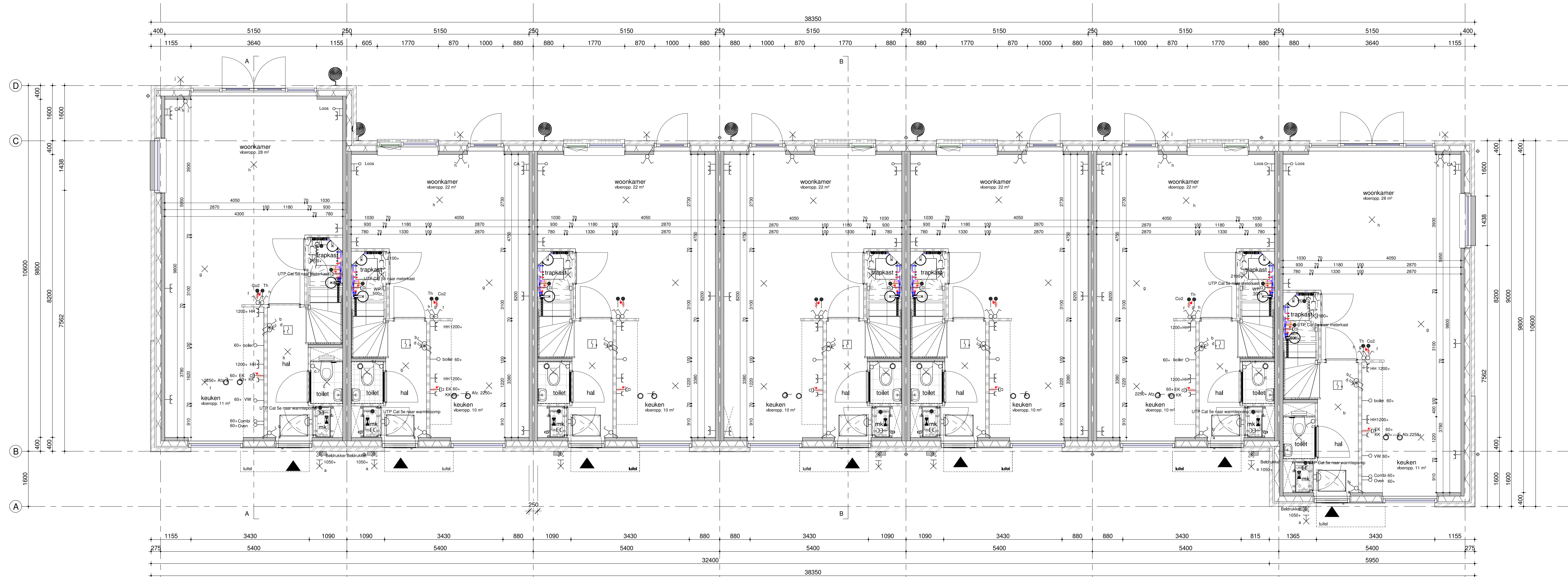
1 bouwnummer get. 350 Type G1 Begane grond / PEIL=0 1:50 2 bouwnummer get. 349 Type H1 3 bouwnummer get. 348 Type H1 4 bouwnummer get. 347 Type H1 5 bouwnummer get. 346 Type H1 6 bouwnummer get. 345 Type H1 7 bouwnummer get. 344 Type G1
