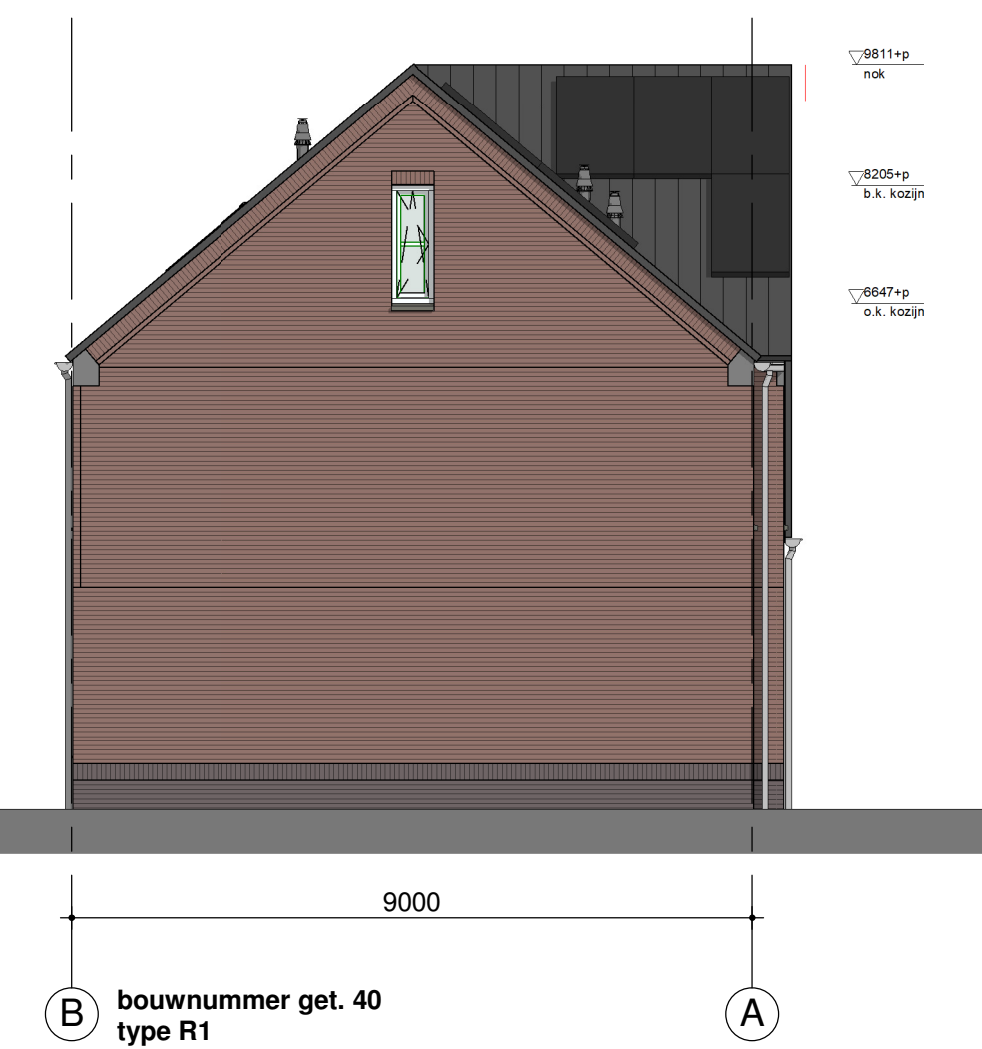
linker zijgevel 1:100
