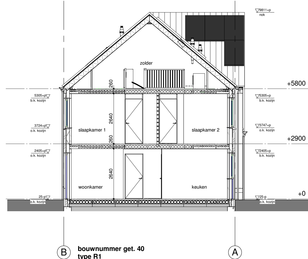
doorsnede A-A 1:100
