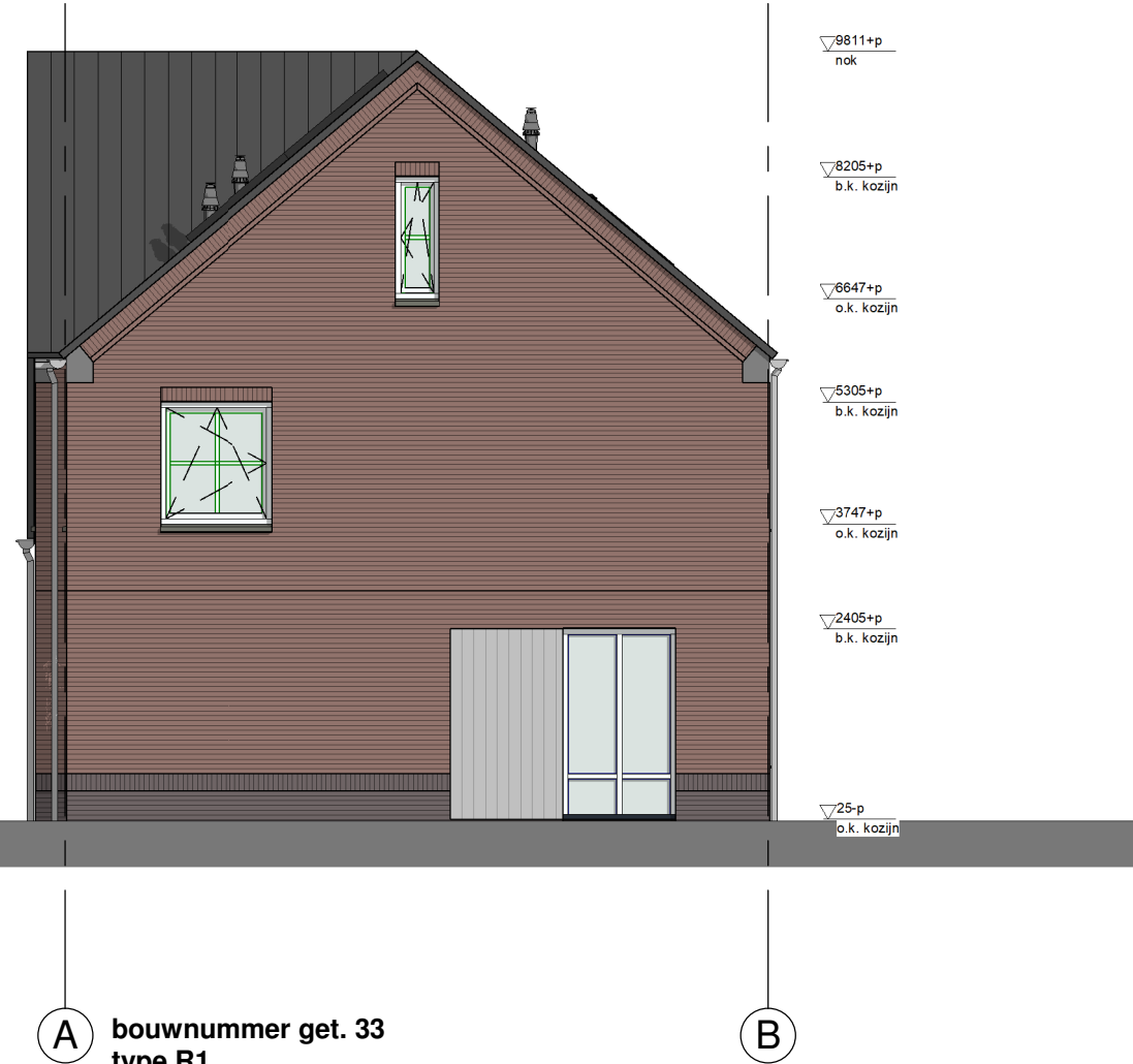
rechter zijgevel 1:100
