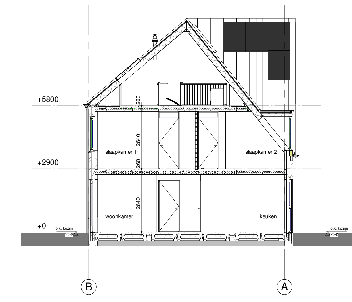
doorsnede B-B 1:100
