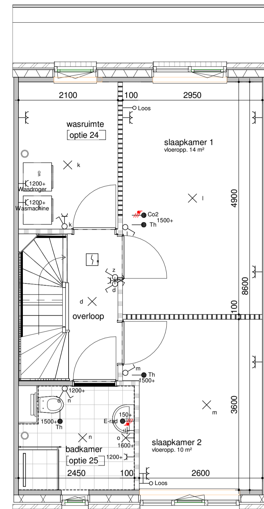
eerste verdieping - vergrote badkamer
