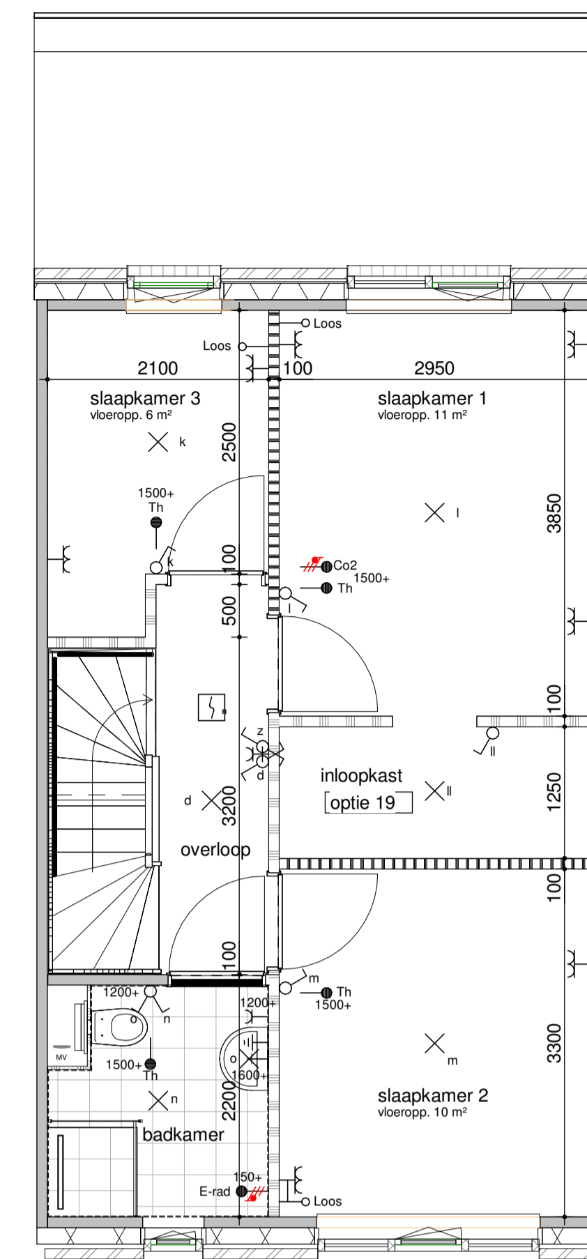
eerste verdieping - inloopkast
