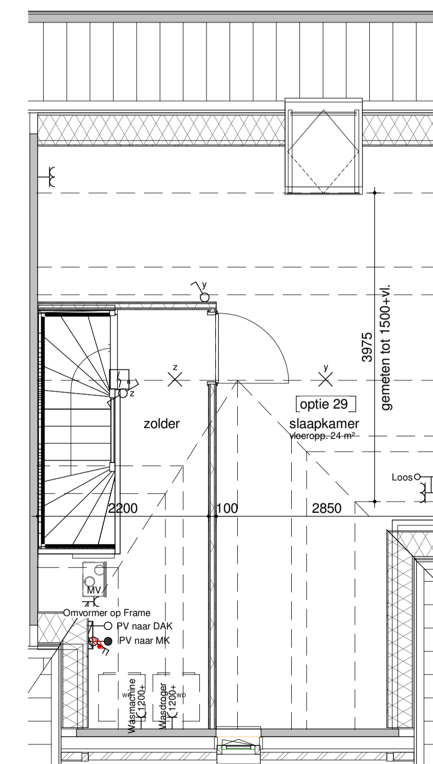
tweede verdieping - zolder L indeling
