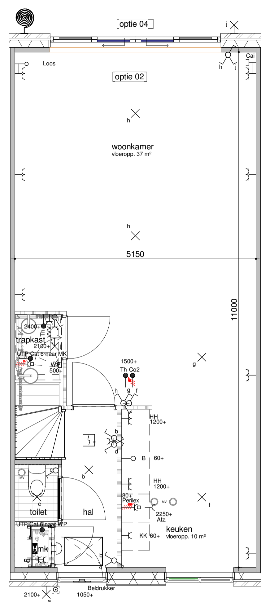
begane grond - optie 2400
