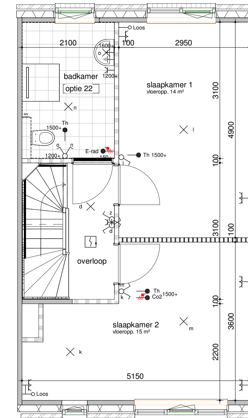
eerste verdieping - badkamer achter
