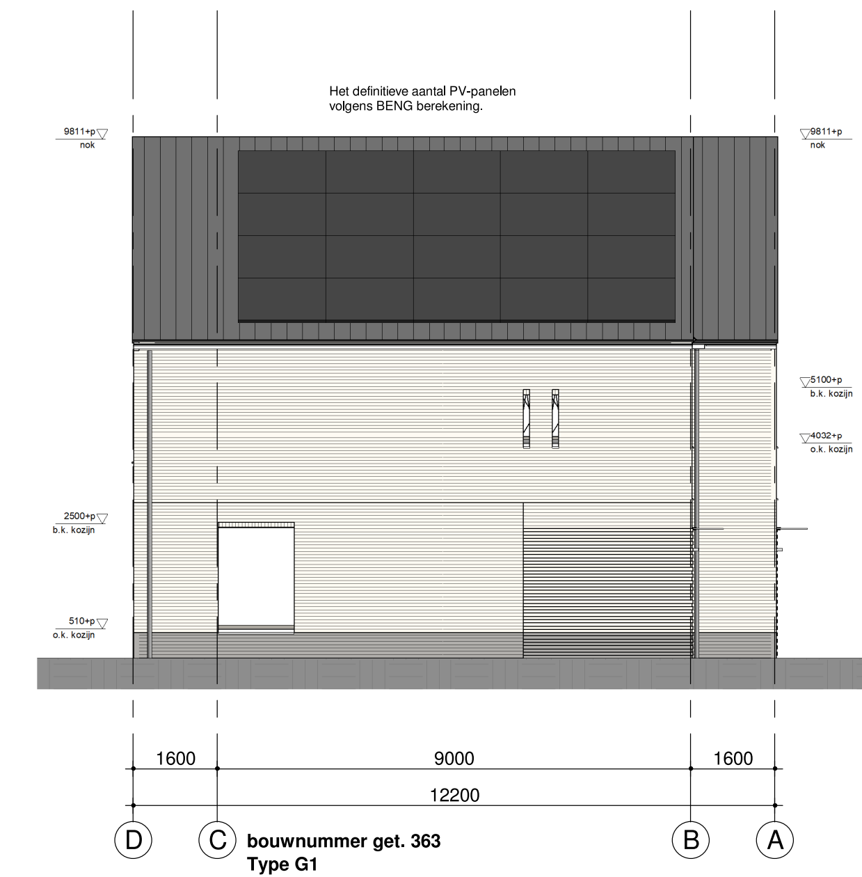
linkerzijgevel 1:100
