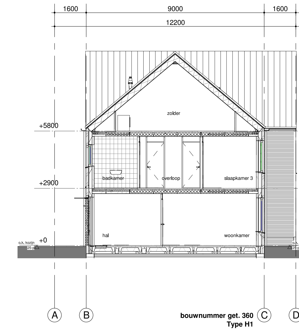
doorsnede B-B 1:100
