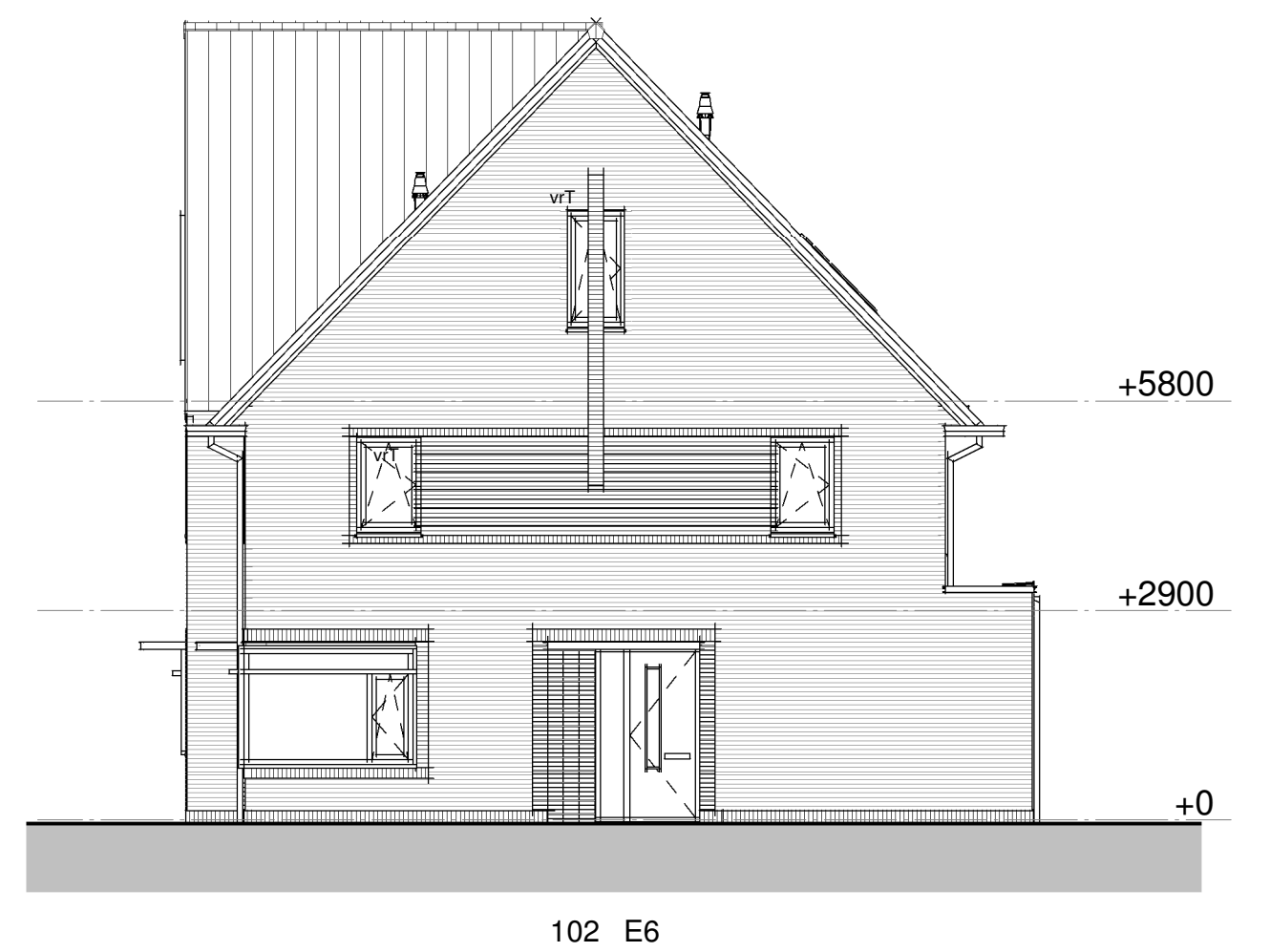
Rechtergevel
