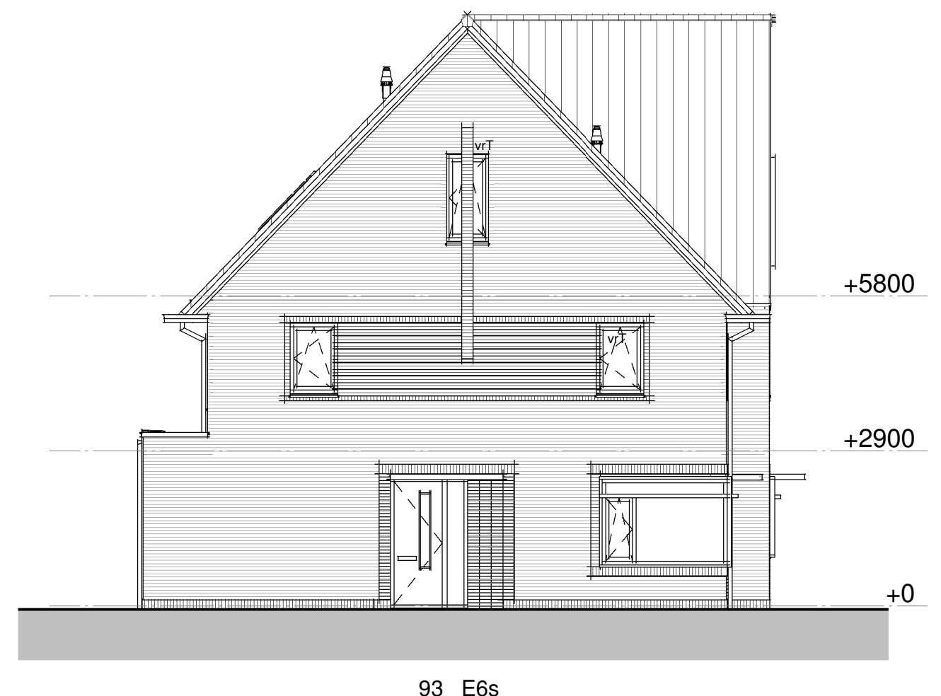
Linkergevel
