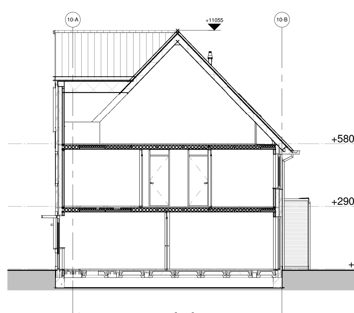
Doorsnede 10-C-C
