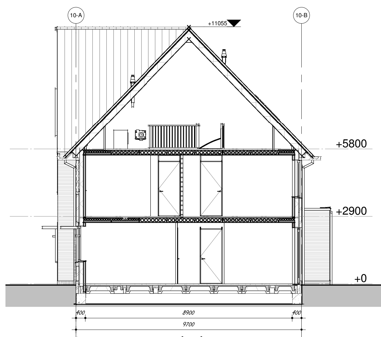
Doorsnede 10-A-A
