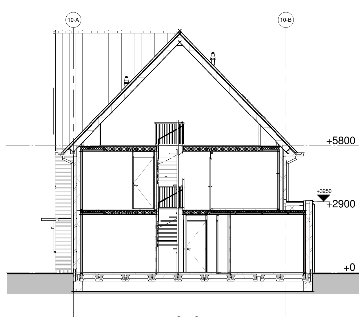
Doorsnede 10-B-B
