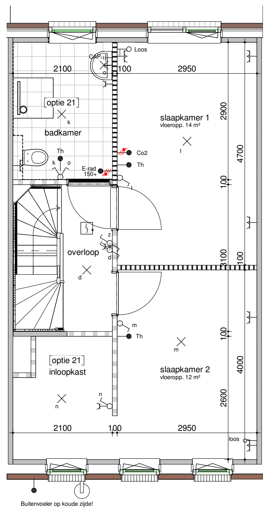
bouwnummer get. 103, 104, 105, 106, 107, 108, 130, 131, 132, 133, 134, 135, 136, 137 eerste verdieping - badkamer achter + inloopkast
