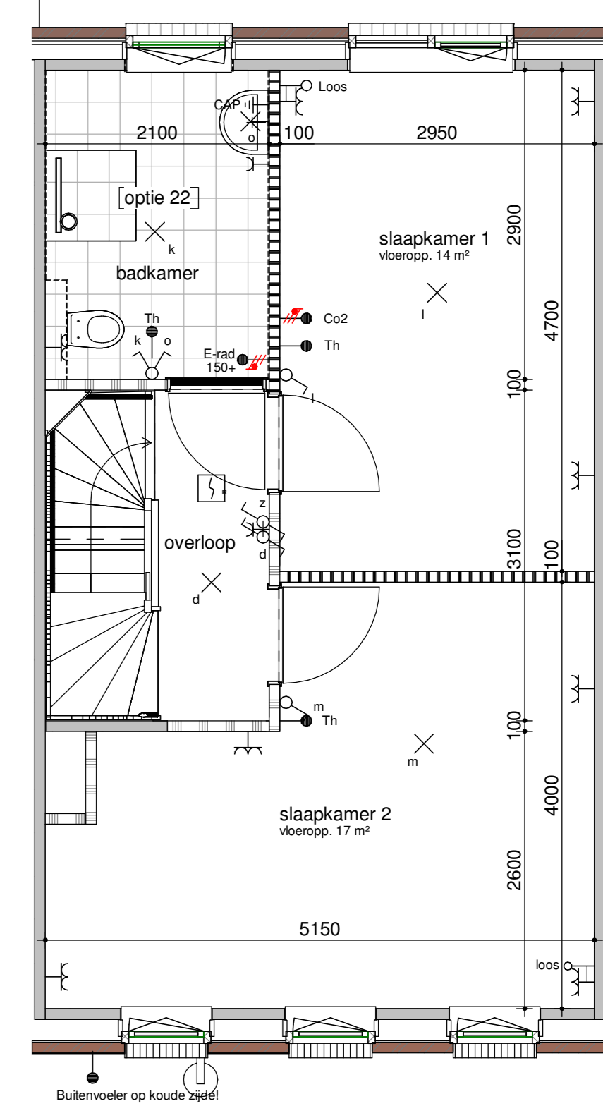
bouwnummer get. 103, 104, 105, 106, 107, 108, 130, 131, 132, 133, 134, 135, 136, 137 eerste verdieping - badkamer achter
