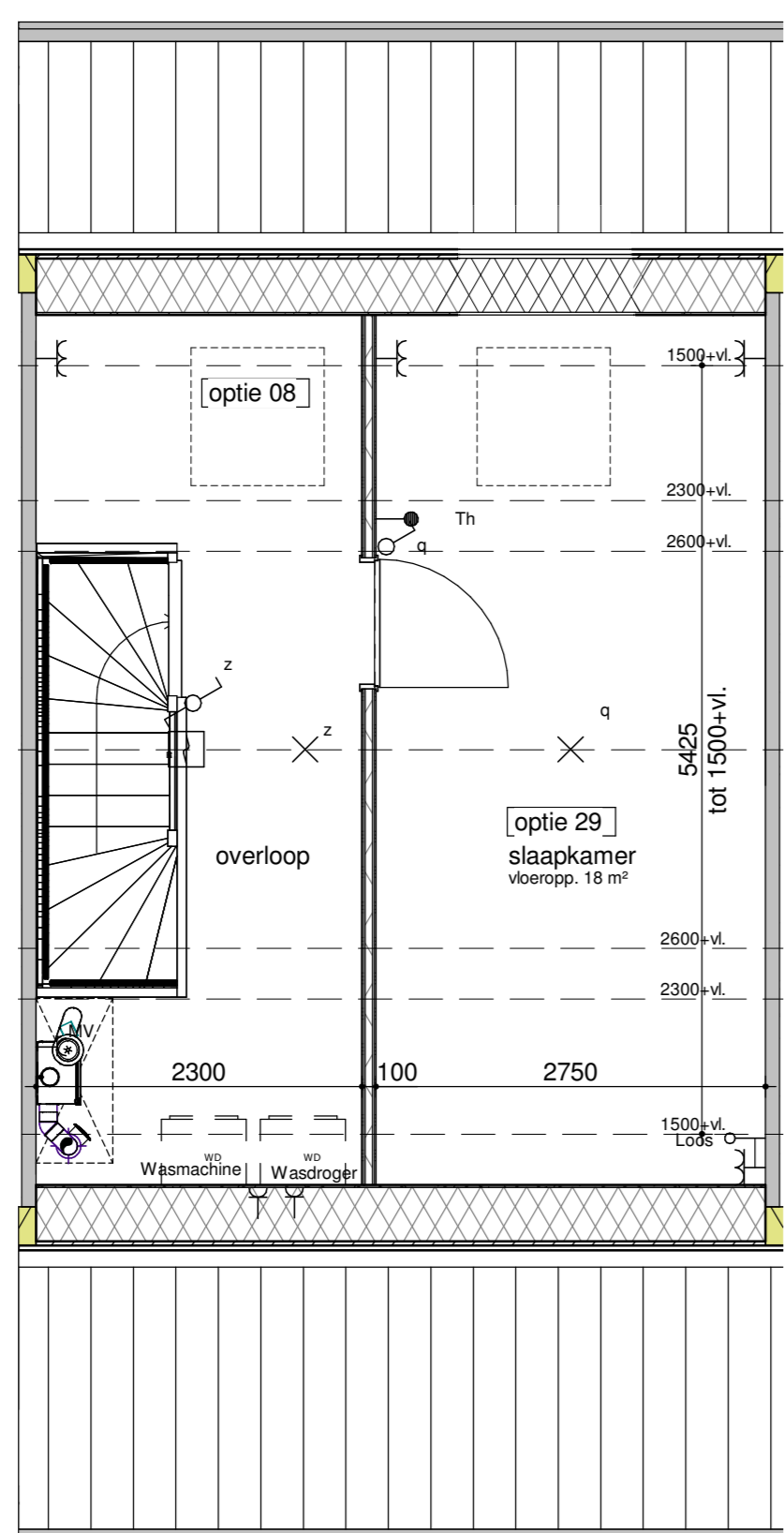
bouwnummer get. 102, 103, 104, 105, 106, 107, 108, 109 129, 130, 131, 132, 133, 134, 135, 136, 137 tweede verdieping - zolderindeling
