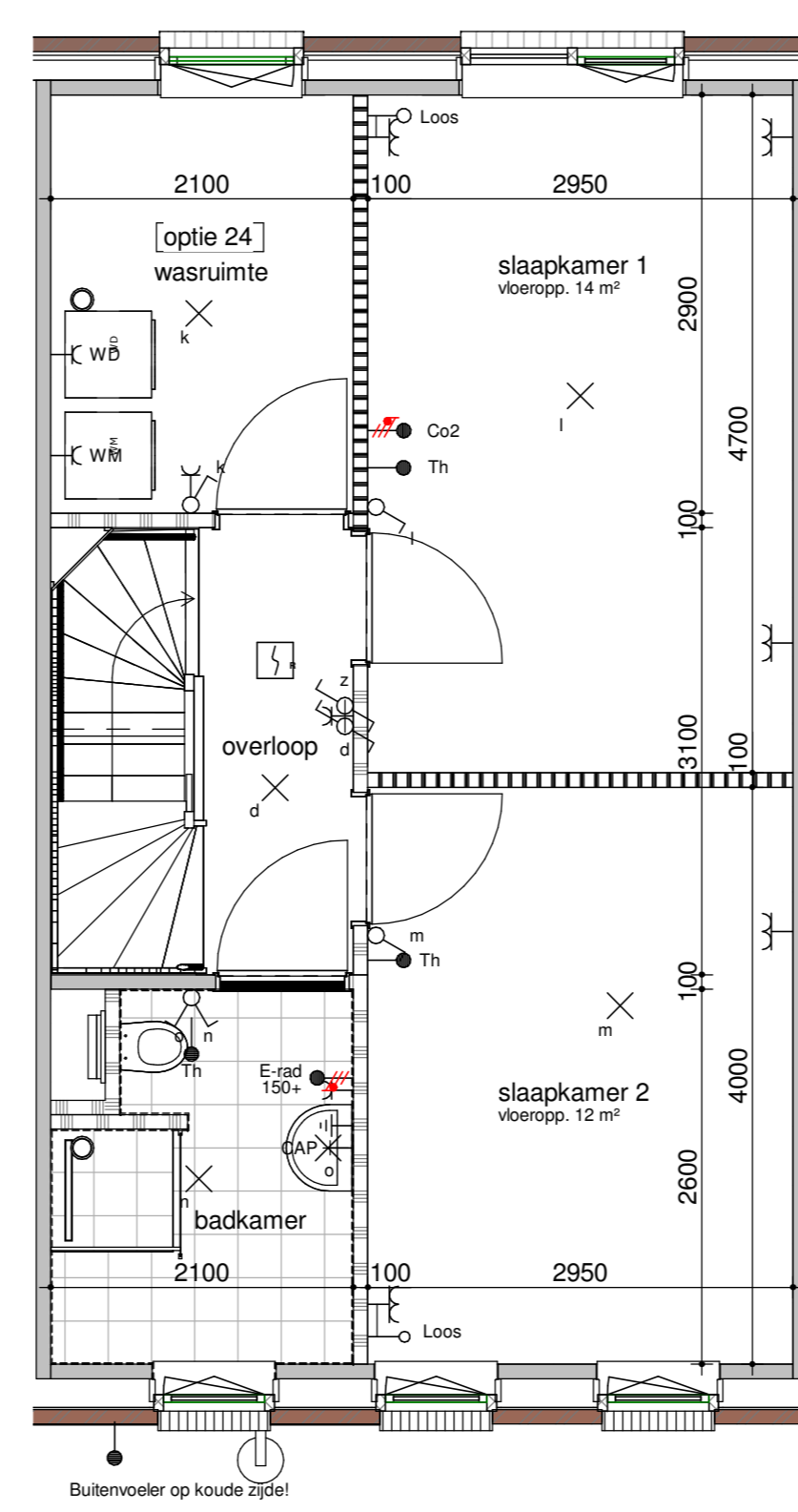
bouwnummer get. 102, 103, 104, 105, 106, 107, 108, 109 129, 130, 131, 132, 133, 134, 135, 136, 137 eerste verdieping - wasruimte
