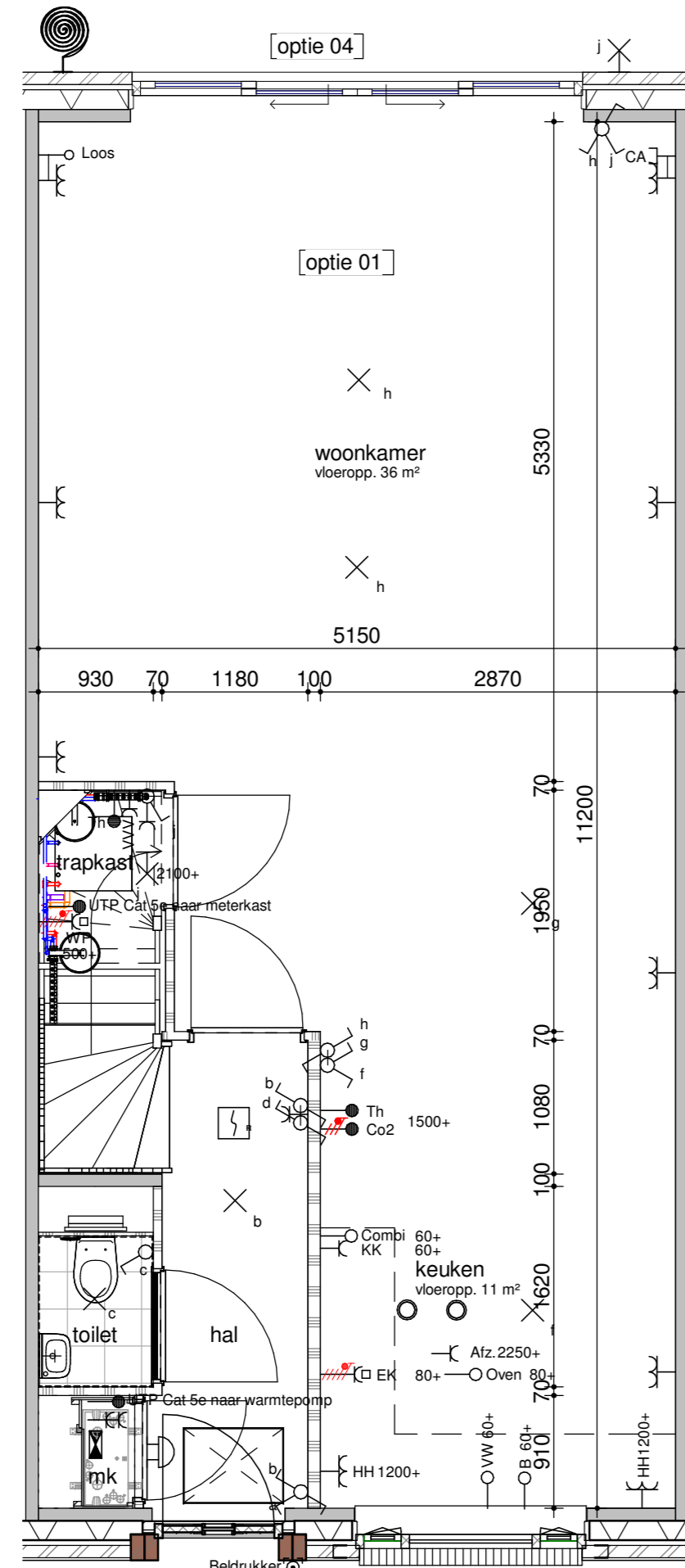
bouwnummer get. 102, 103, 104, 105, 106, 107, 108, 109 129, 130, 131, 132, 133, 134, 135, 136, 137 begane grond - optie 1200
