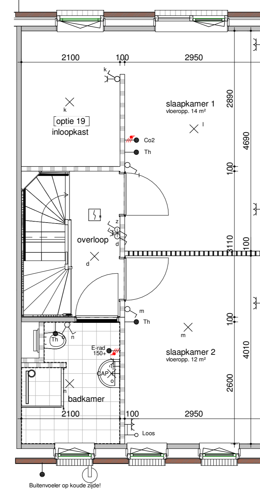
bouwnummer get. 102, 103, 104, 105, 106, 107, 108, 109 129, 130, 131, 132, 133, 134, 135, 136, 137 eerste verdieping - inloopkast
