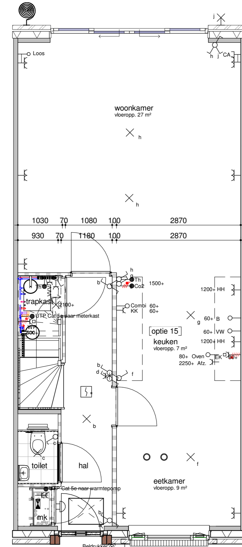
bouwnummer get. 103, 104, 105, 106, 107, 108, 130, 131, 132, 133, 134, 135, 136, 137 begane grond - optie middenkeuken
