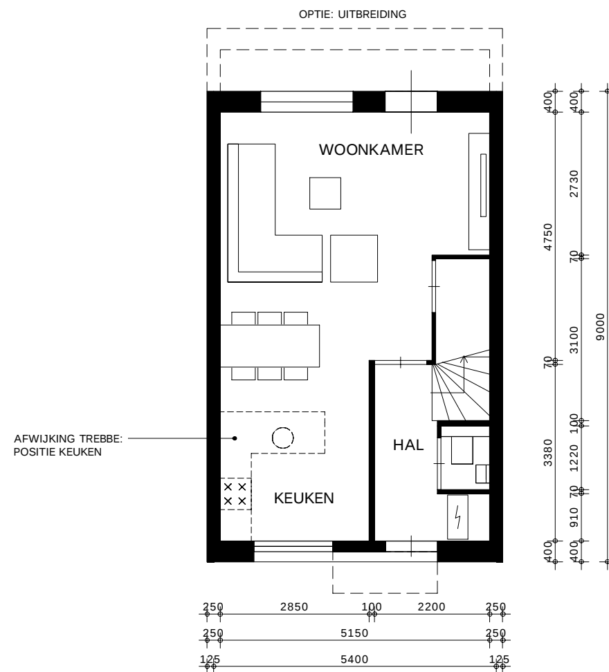
BEGANE GROND
