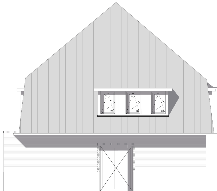
zijgevel
