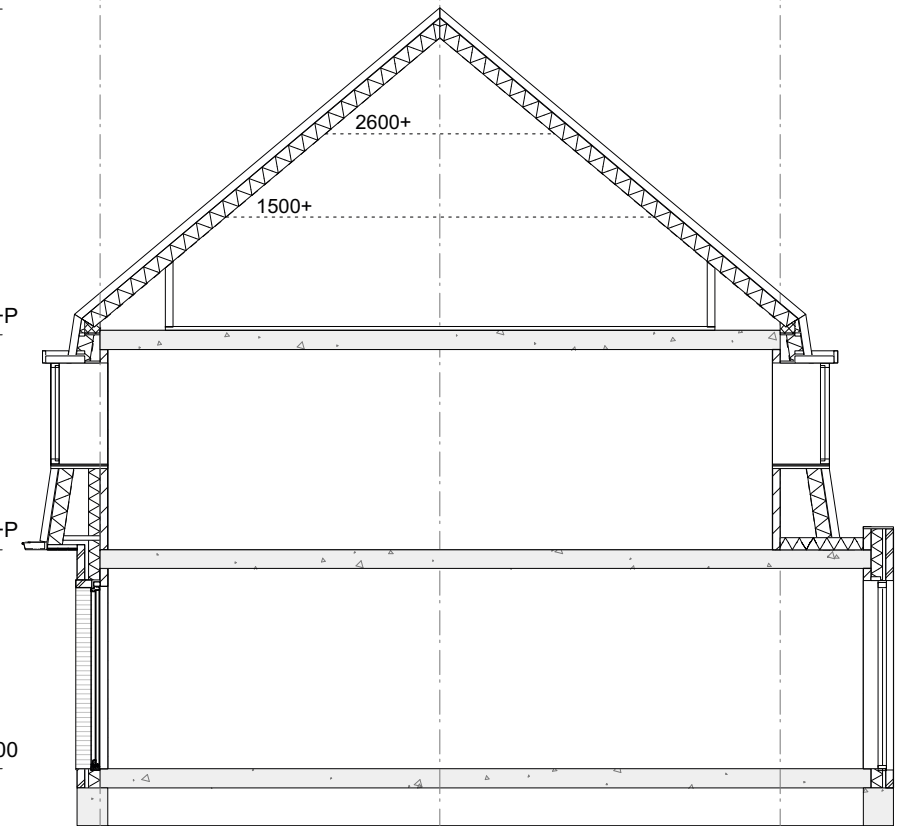
doorsnede
