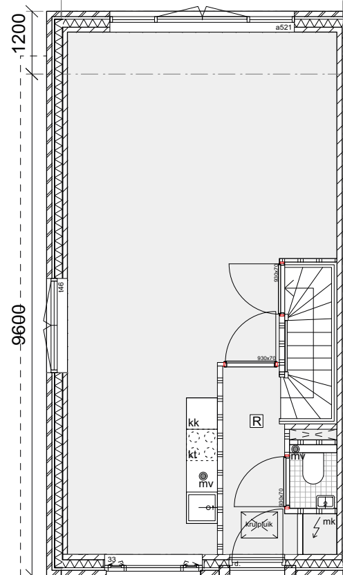
begane grond
