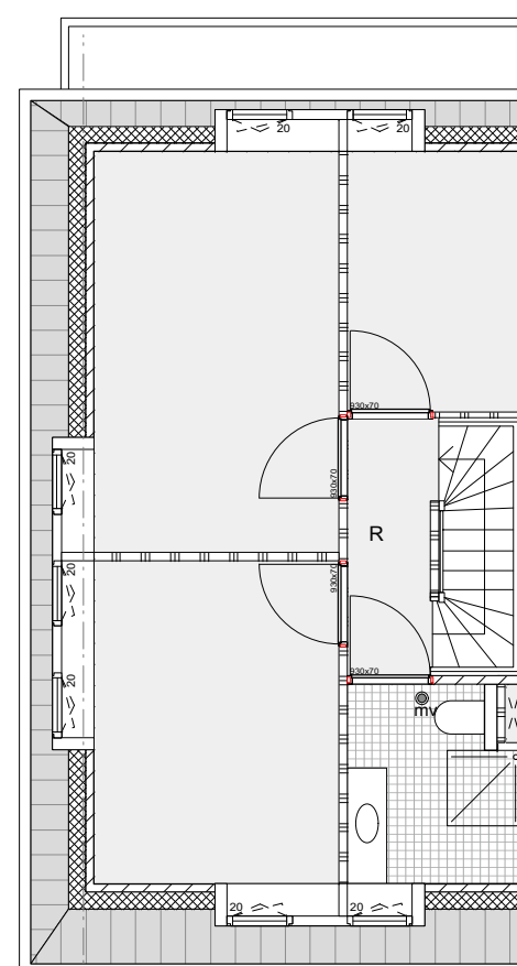
1e verdieping
