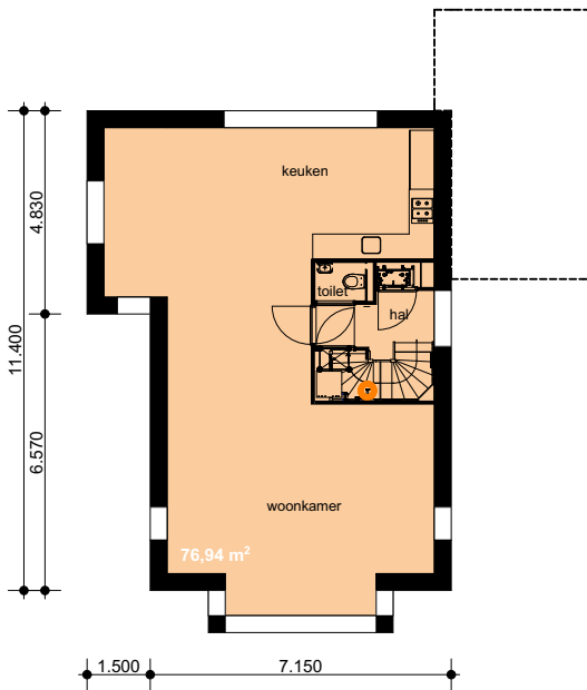
begane grond
