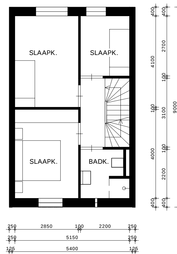
1e VERDIEPING
