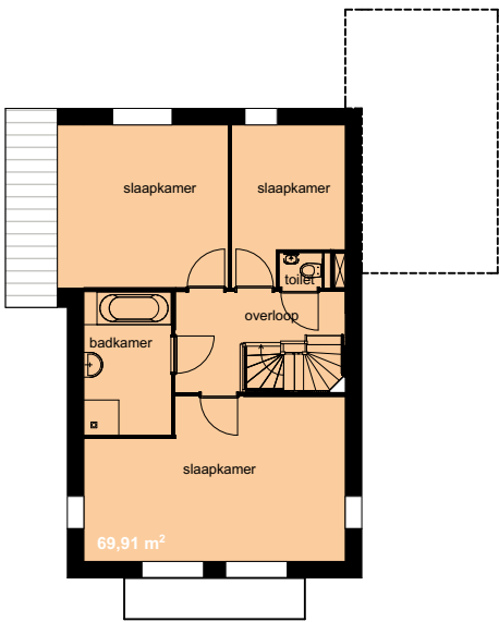
1e verdieping
