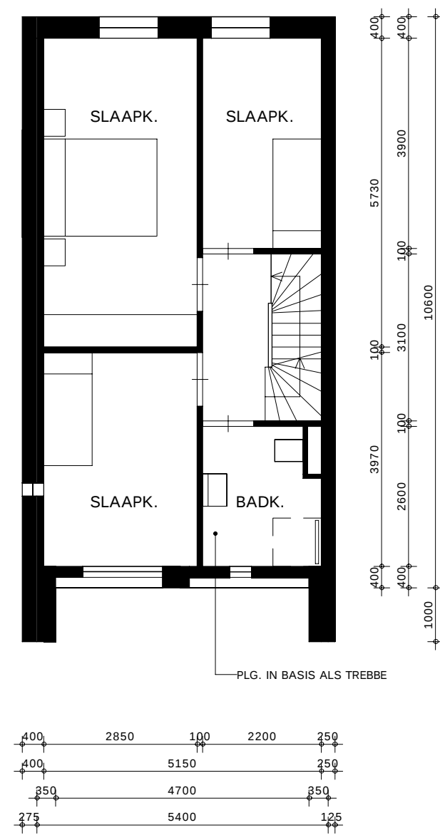
1e VERDIEPING
