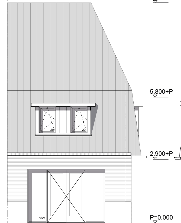
achtergevel
