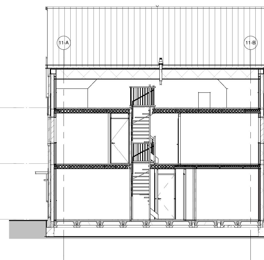
Doorsnede 11-B-B
