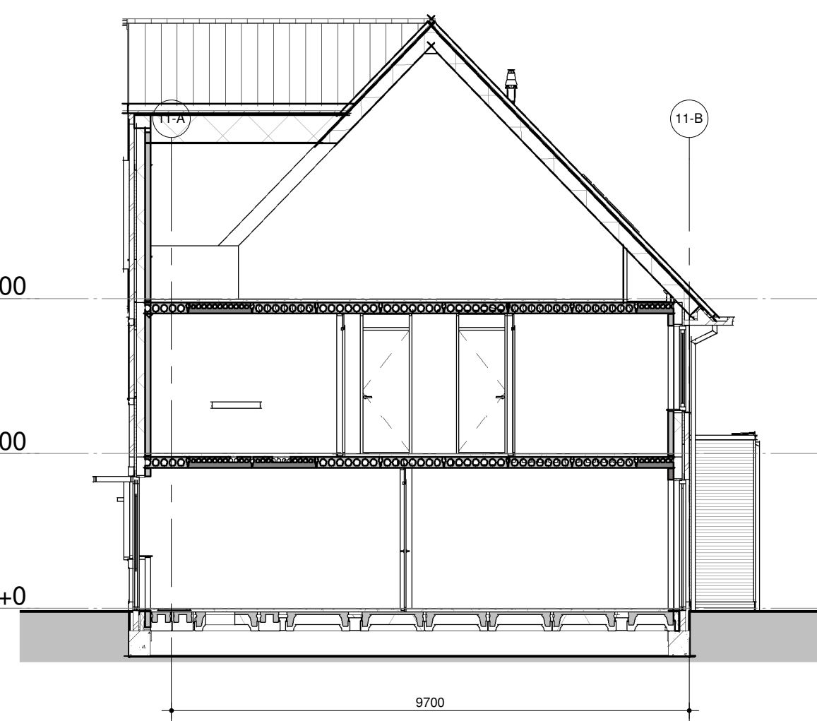
Doorsnede 11-A-A
