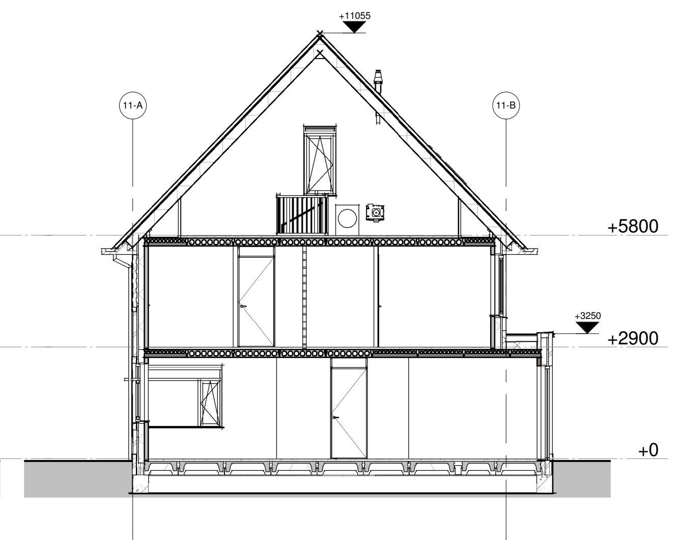
Doorsnede 11-C-C
